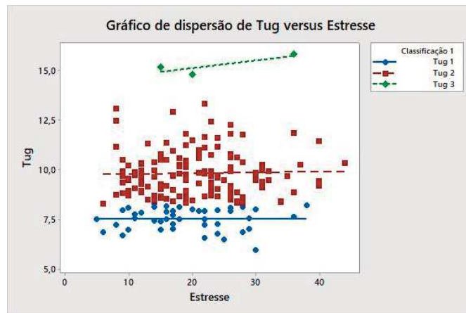
Figura 3. Dispersão entre TUG e estresse de acordo com o desempenho no teste TUG.
