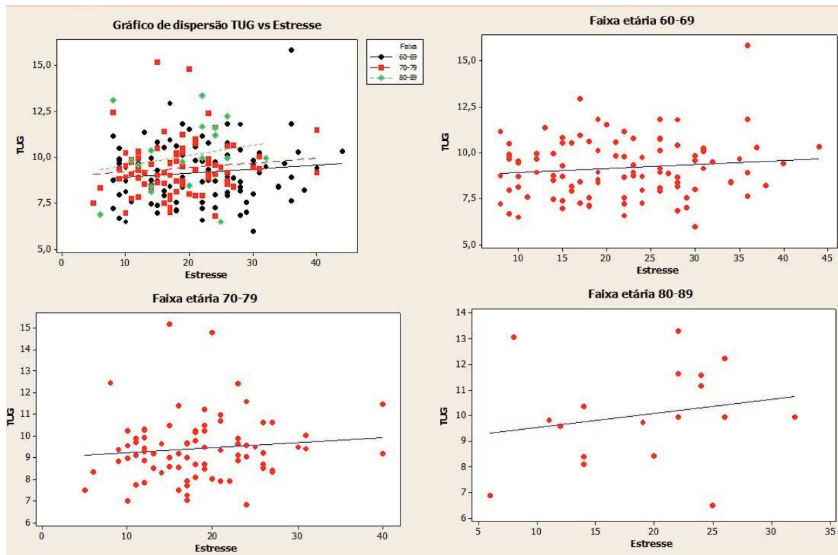
Figura 2. Gráfico de dispersão entre TUG e Estresse de acordo com faixa etária.
