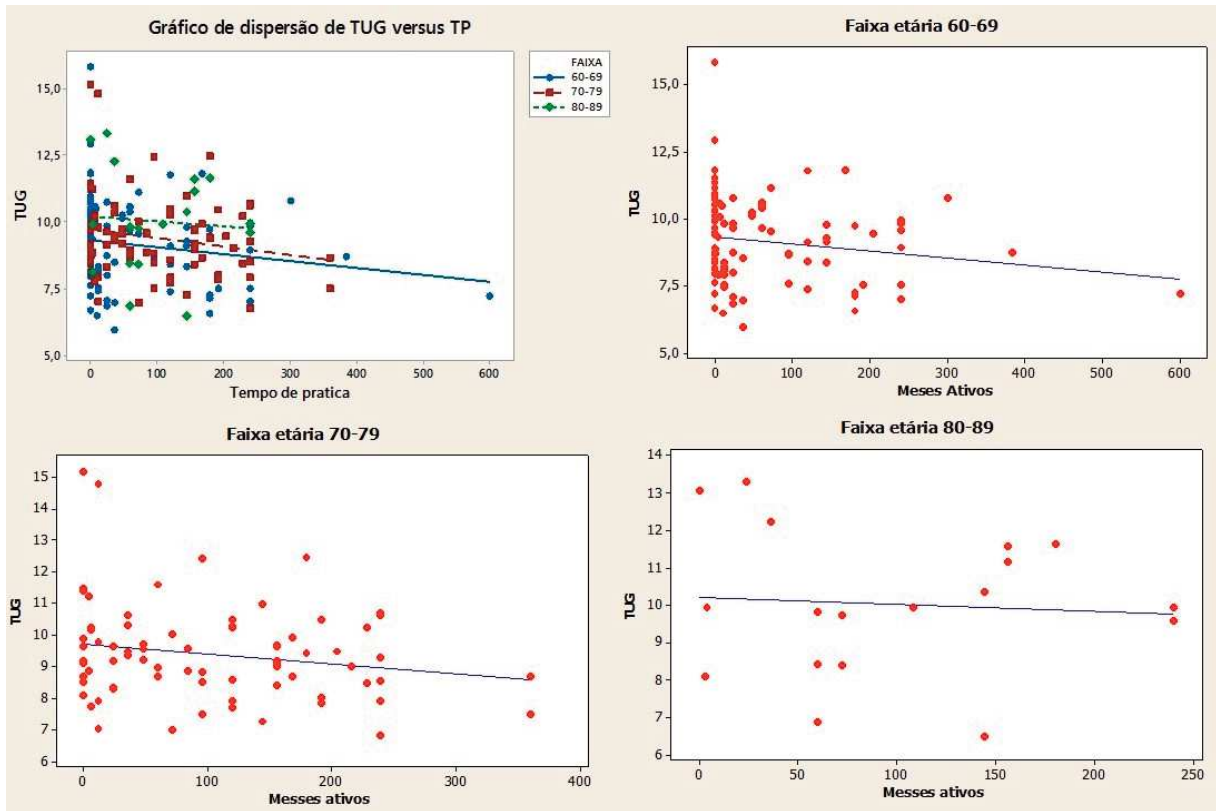
Figura 1. Gráficos de dispersão entre TUG e o tempo de prática (TP) de acordo com faixa etária.
