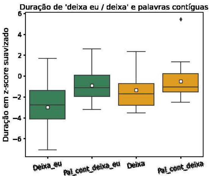
Figura 2 - Boxplot da duração em z-score suavizado
