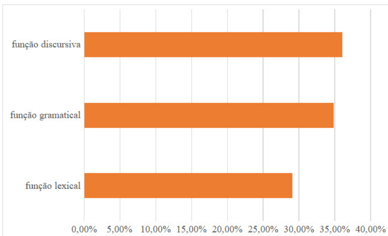
Gráfico 1 - Descrição da funcionalidade do verbo deixar em textos orais espontâneos
