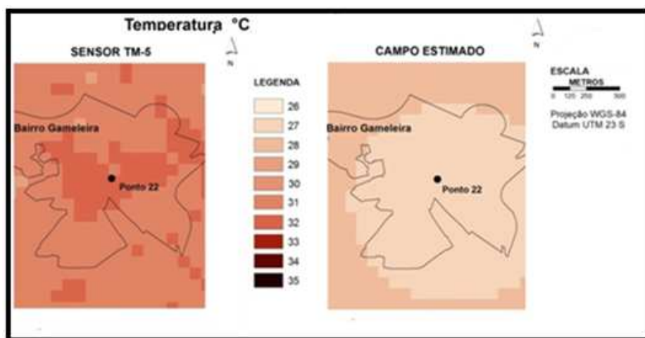
Figura 5. Comparativo em C° para o bairro Nova Gameleira Sensor TM/Landsat-5 e CampoEstimado
