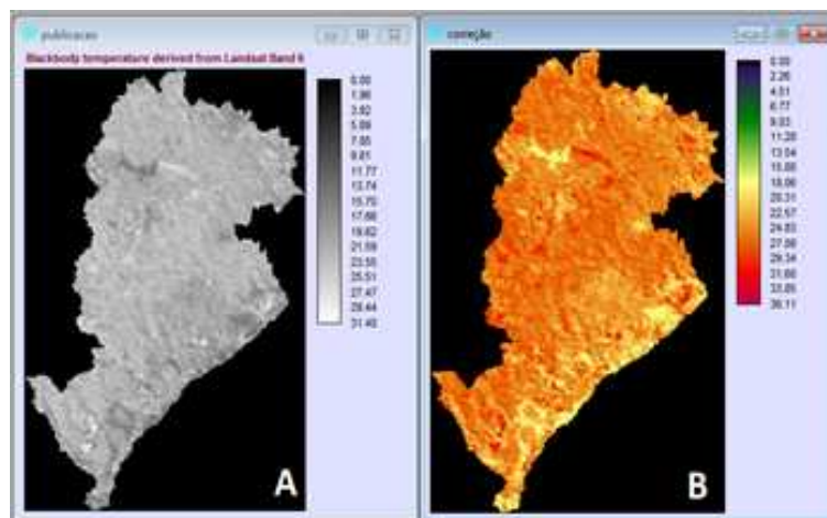
Figura 2. Imagens termais, com resolução de 120 m.: a) Thermal b) Thermal + Reclass
