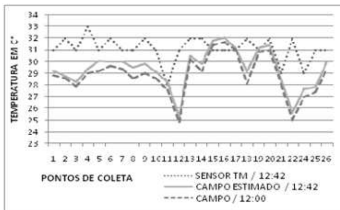
Figura 4. Comparativo da temperatura em C° entre os métodos de coleta
