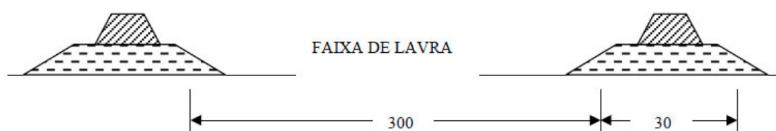
Figura 3.34 – Esquema para retomada de rejeitos – Mineração Caraíba (PIGNATON, 2010).
