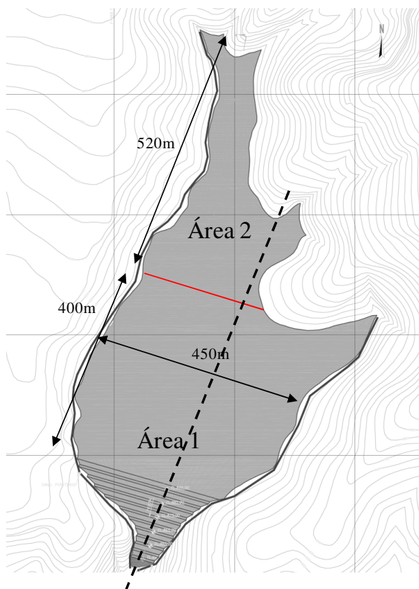
Figura 5.4 – Divisão do reservatório.
