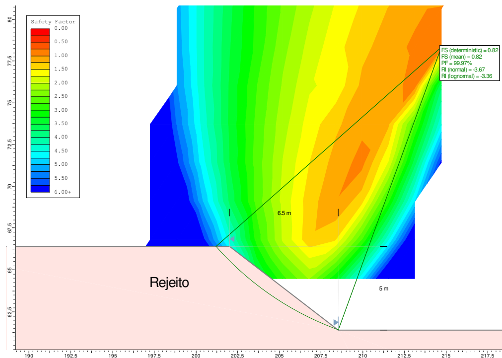
Figura A.36 - Análise de Estabilidade – Desmonte Hidráulico – Inclinação 1,3H:1V – Fator Ru = 0,15.
