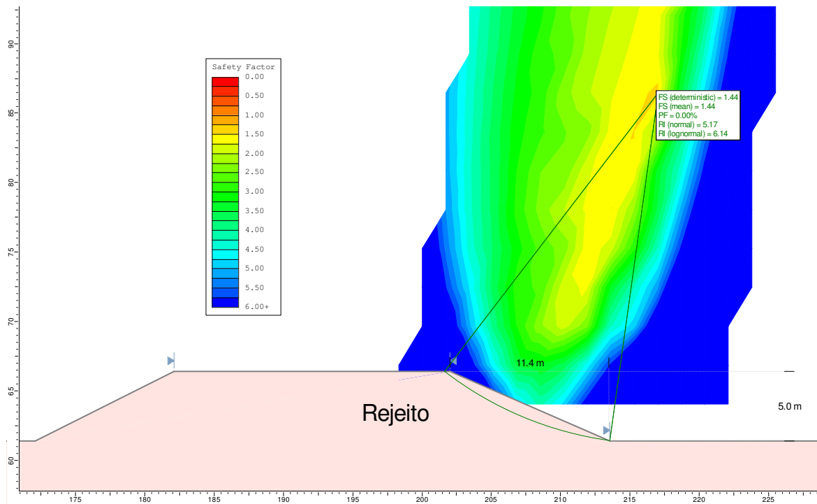
Figura A.40 - Análise de Estabilidade – Desmonte Hidráulico – Inclinação 2,3H:1V – Fator Ru = 0,15.
