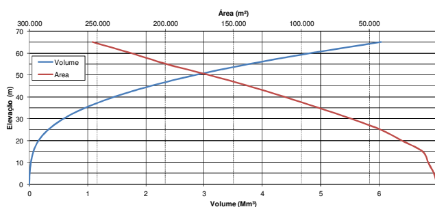
Figura 4.3 – Curva cota área volume do Empilhamento Drenado.
