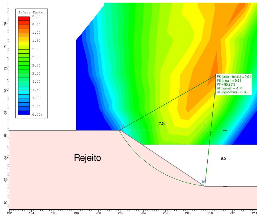
Figura A.46 - Análise de Estabilidade – Desmonte Hidráulico – Inclinação 1,5H:1V – Fator Ru = 0,20.
