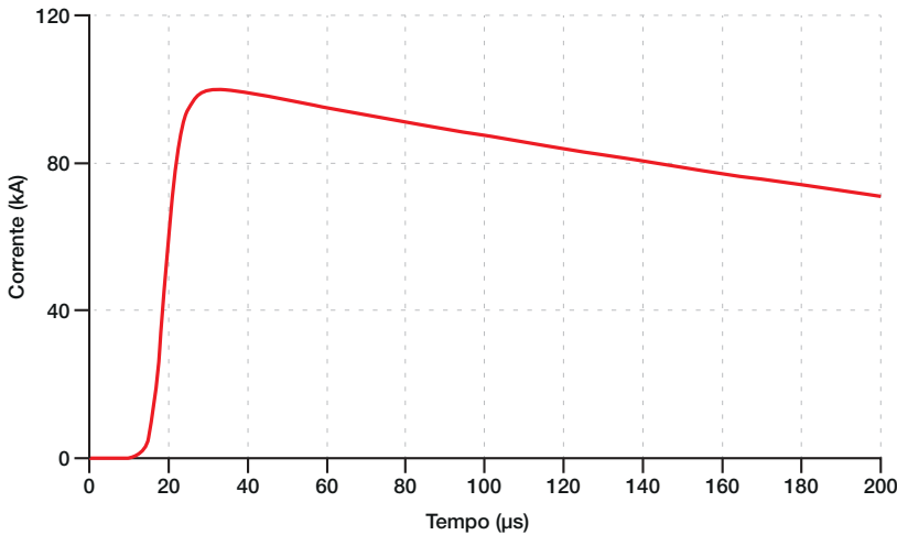
Fig. 6.3 – Onda de corrente utilizada nas simulações. Descarga principal positiva, forma de onda 10/350 \mu\text{s} e valor de pico de 100kA [6].
