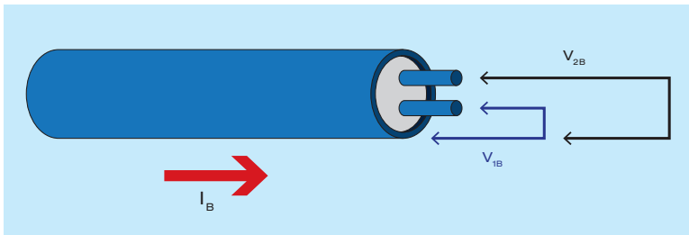
Fig.5.19 – Tensões induzidas entre os condutores internos e a blindagem.
