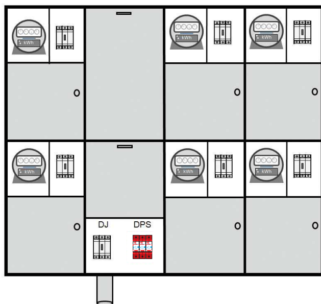
Fig.8.11 – Exemplo de instalação de DPS Classe I dentro da caixa de medição em rede 220/127V.
