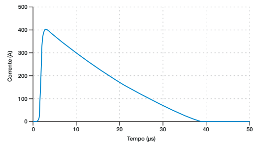
Fig. 3.25 - Corrente através dos DPS baseados em tecnologia MOV ou semiconductor instalado nas portas LAN dos equipamentos da Fig. 3.17.
