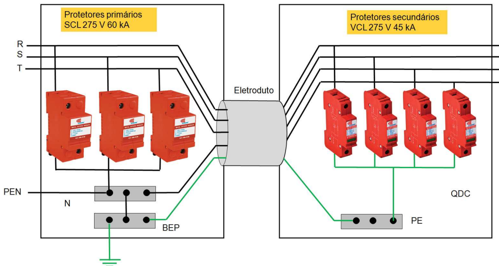
Fig. 9.8 – Exemplo de aplicação de DPS na entrada de energia elétrica da Estação de Telecomunicações.
