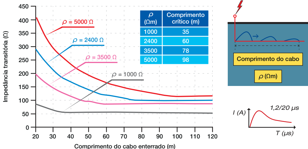
Fig. 4.26 – Comprimento crítico de malha de aterramento constituída de um cabo horizontal enterrado em solos de 1000, 2400, 3500 e 5000 \Omega m . Adaptado de [7].
