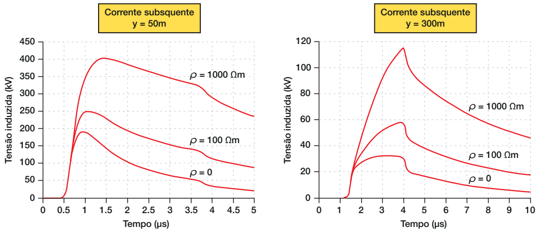
Fig. 3.34 - Tensões induzidas em um condutor a h = 5\text{m} de altura; Descarga subsequente (50kA) incidindo a 50m e 300m, para diferentes valores de resistividade do solo.
