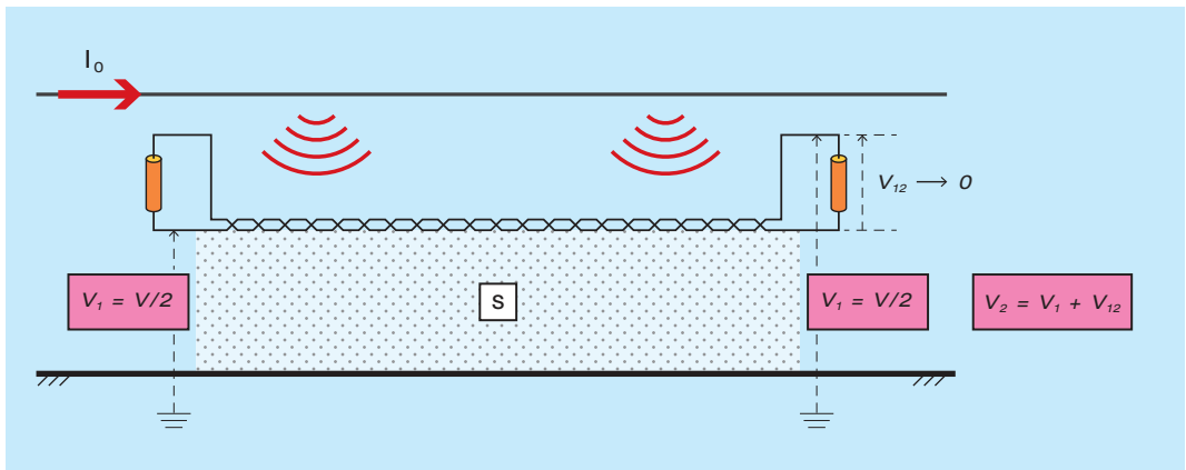
Fig.5.17 – Tensões de modo comum em um cabo de par trançado.
