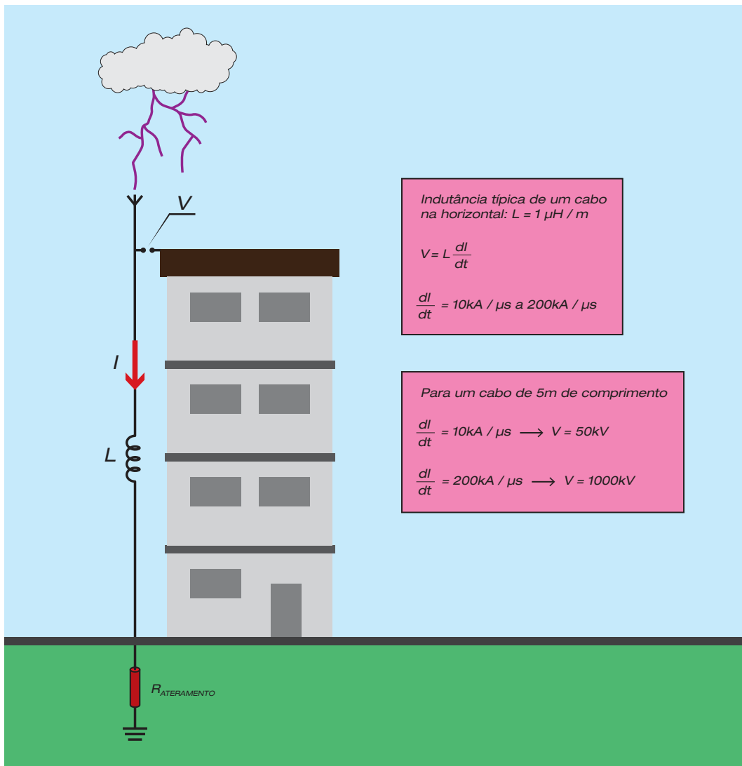
Fig. 4.30 – Tensões desenvolvidas em um condutor de descida de um SPDA.
