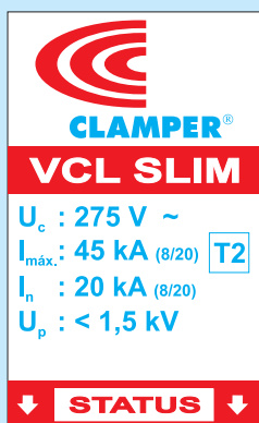
Fig. 8.1 – Identificação dos principais parâmetros de um DPS CLAMPER para redes elétricas. (A) DPS Classe I/II; (B) DPS Classe II.
