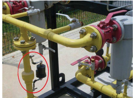
Fig. 10.16 - Proteção de junta isolante no citygate. DPS modelo GCL EC EX
