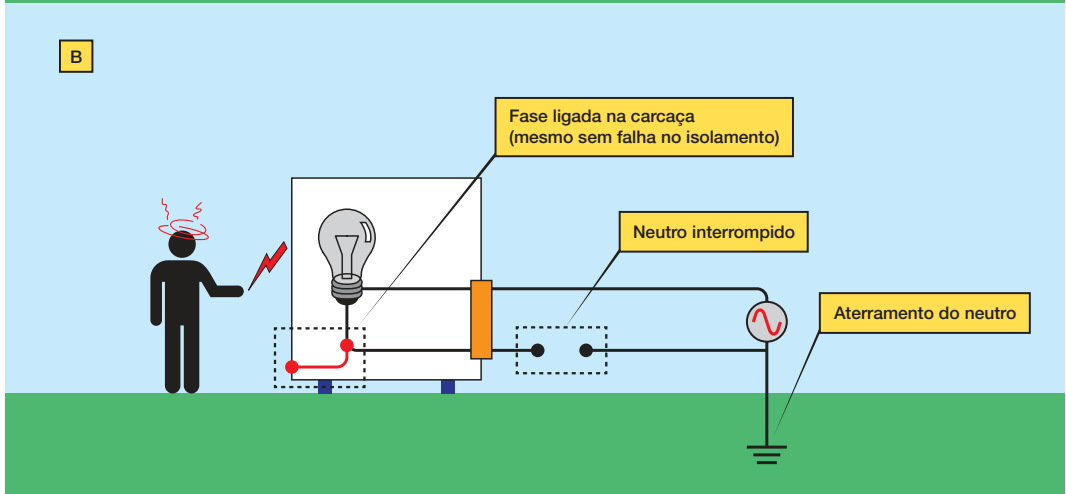
Fig. 4.2 – Utilização do neutro como cabo de proteção. Se o cabo neutro for interrompido, a carça fica energizada, mesmo se não houver contato acidental.
