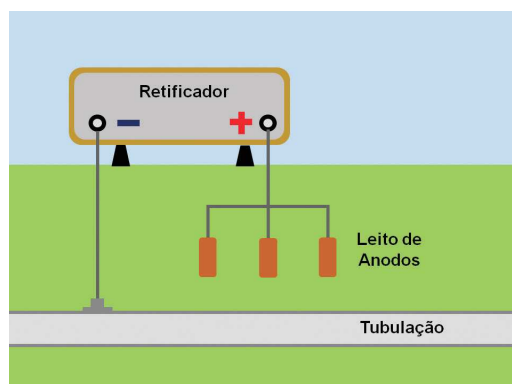
Fig. 10.8 - Sistema de proteção catódica contra corrosão acelerada.
