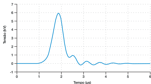
Fig. 3.19 - Tensão desenvolvida na porta LAN do roteador da Fig. 3.14.
