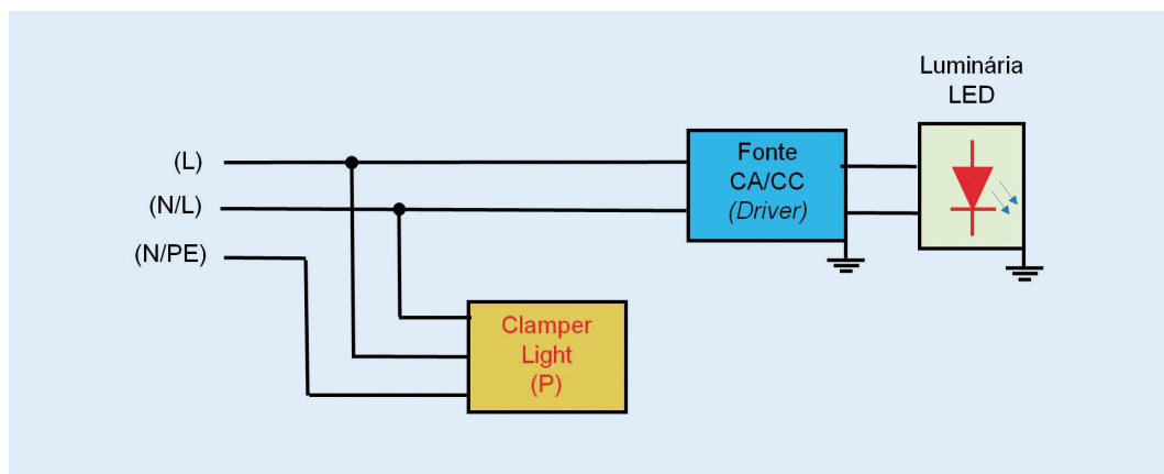
Fig.10.7 – Detalhe conexão em paralelo com a luminária.
