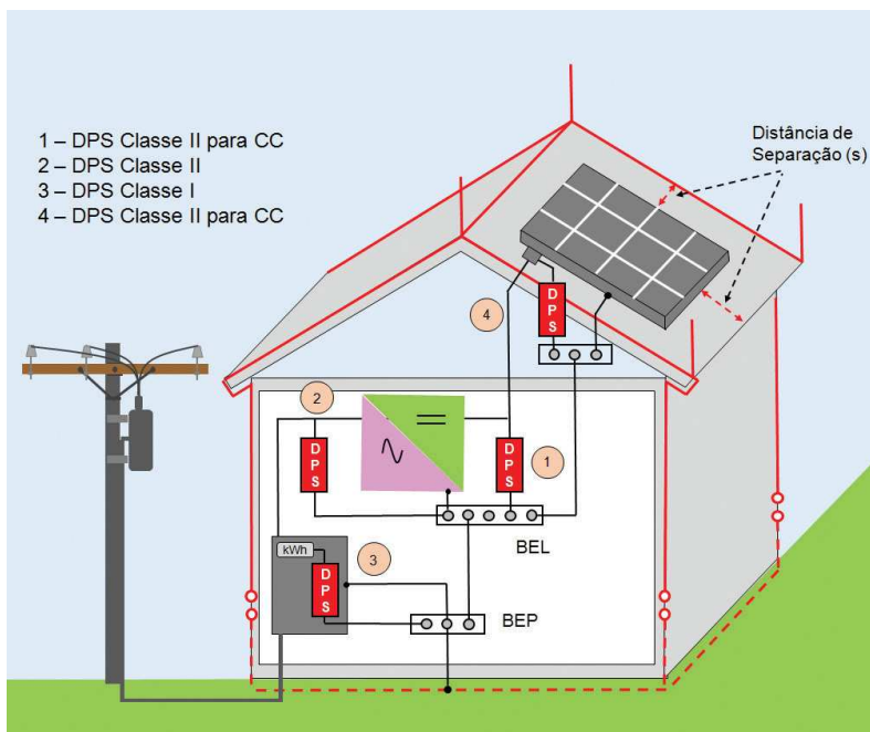
Fig.9.26 – Localização dos DPS no caso de painéis isolados do SPDA. Adaptado de [4].
