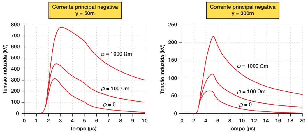
Fig. 3.33 - Tensões induzidas em um condutor a h = 5\text{m} de altura; Descarga principal negativa (110kA) incidindo a 50m e 300m, para diferentes valores de resistividade do solo.
