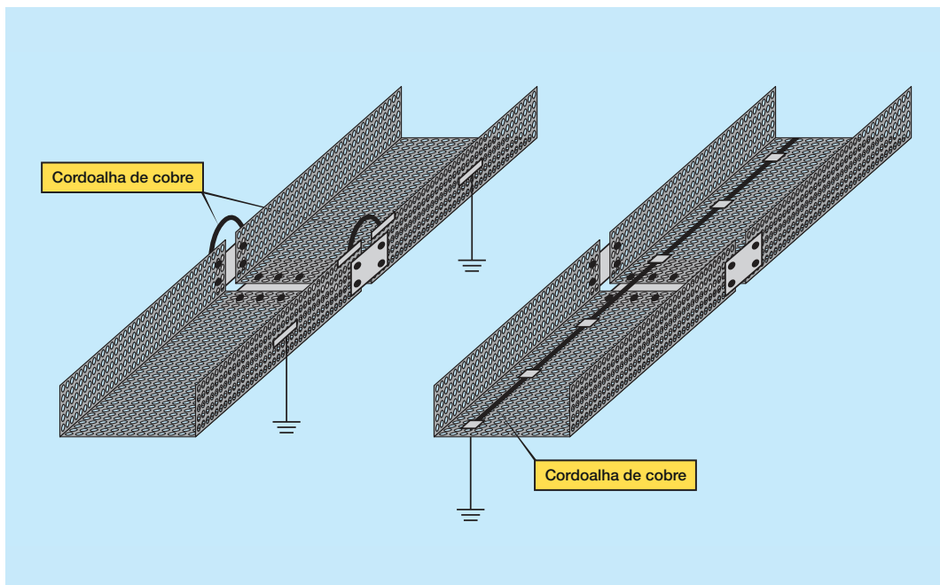
Fig. 4.43 – Bandejas eletricamente bem conectadas que podem integrar o sistema de equalização interno.
