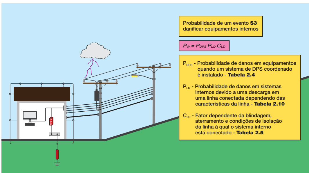
Fig. 2.38 Probabilidade de um evento S3 danificar equipamentos internos ( P_W ).
