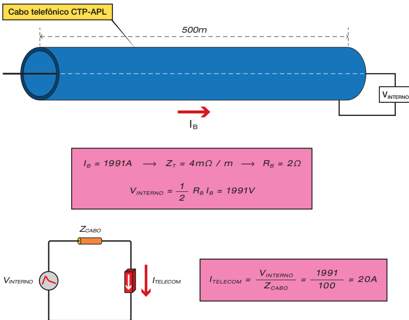
Fig. 6.37 - Cálculo da corrente que circula pelo DPS instalado entre um dos condutores internos e a barra de equalização da edificação. Foi considerado um cabo telefônico blindado, tipo CTP-APL, com resistência da blindagem igual a 4\text{m}\Omega/\text{m} . A impedância de surto interna do cabo ( Z_{\text{cabo}} ) foi considerada como sendo igual a 100\Omega .
