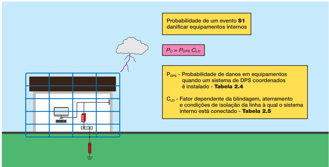
Fig. 2.28 - Probabilidade de um evento S1 danificar equipamentos internos ( P_c ).
