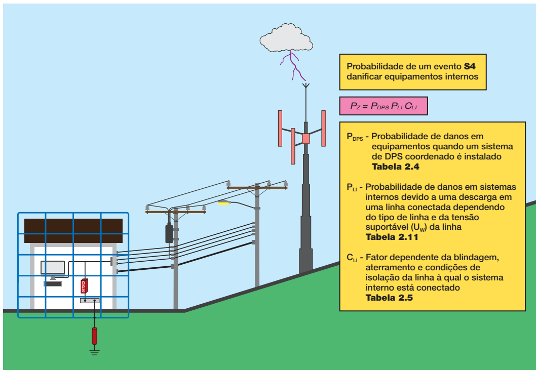
Fig. 2.42 - Probabilidade de um evento S4 danificar equipamentos internos ( P_Z ).
