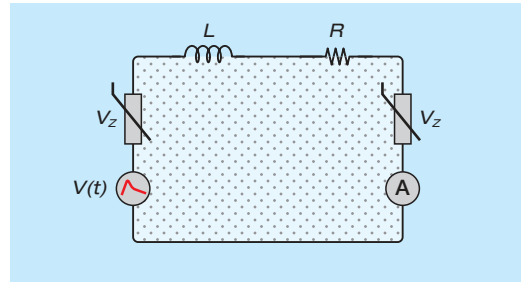
Fig. 3.24 - Circuito equivalente da situação apresentada na Fig. 3.17, supondo instalação de DPS do tipo MOV ou semiconductor nas portas LAN do computador e do roteador.
