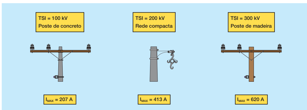
Fig.6.26 – Valores típicos das TSI de estruturas de redes de distribuição de 13,8kV e valores máximos da corrente que se propaga pela rede sem provocar disrupções.
