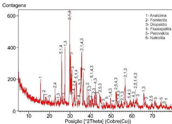
Figura 7. Difratograma de raios-x do kamafugito.
