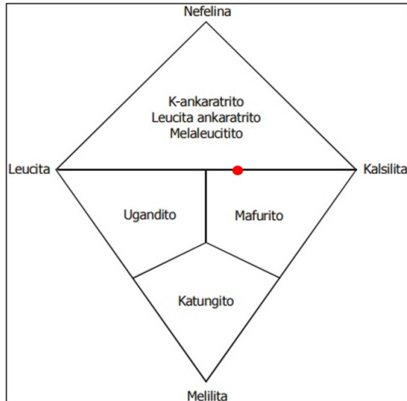
Figura 10. Diagrama de classificação das rochas kamafugíticas ou ankartriticas. Ponto vermelho representa a classificação do kamafugito estudado. Retirado de Silva (2006) e adaptado de Sahama (1974).
