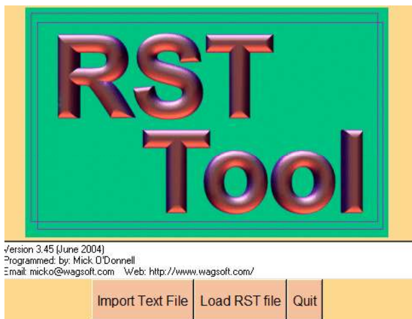
Figura 14 – Programa RSTTool
