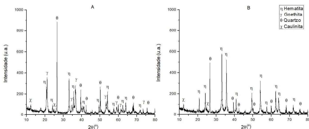
Figura 1: Difratogramas das amostras de RMF in natura (A) e calcinadas (B)
