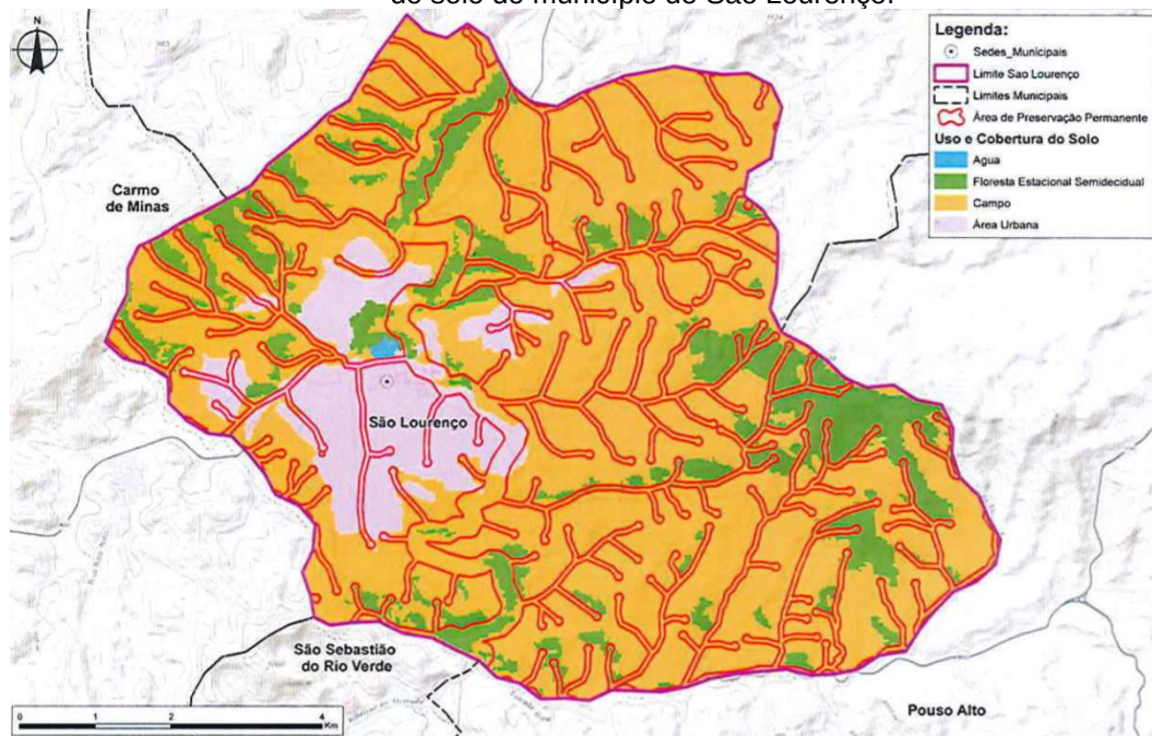
Figura 3 – Mapa de áreas de preservação permanente e uso e cobertura do solo do município de São Lourenço.
