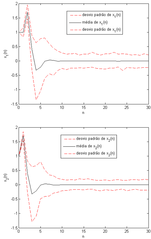
Figura 11: Estados x_1(n) e x_2(n) . As linhas contínuas indicam as média das trajetórias dos estados controlados usando ações obtidas via aplicação do Teorema 4.1, e as linhas tracejadas indicam o desvio padrão de cada estado do sistema.
