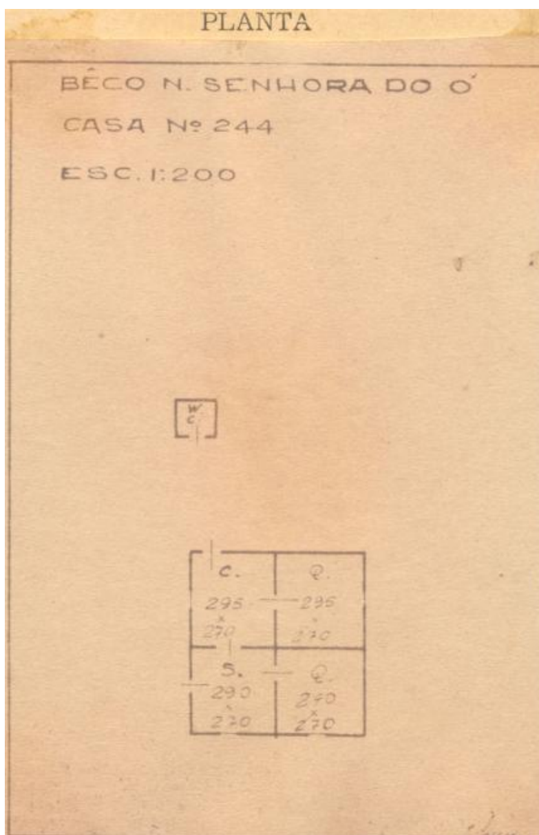
Figura 29: Planta da casa 140 - Em 1956
