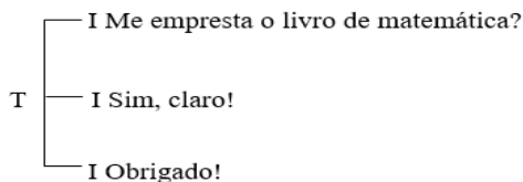
Figura 1: Estrutura hierárquica 1.
