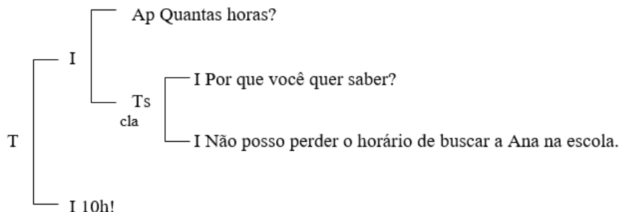
Figura 4: Estrutura hierárquica 4.
