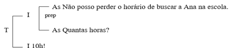
Figura 3: Estrutura hierárquica 3.
