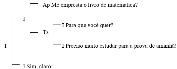
Figura 2: Estrutura hierárquica 2.
