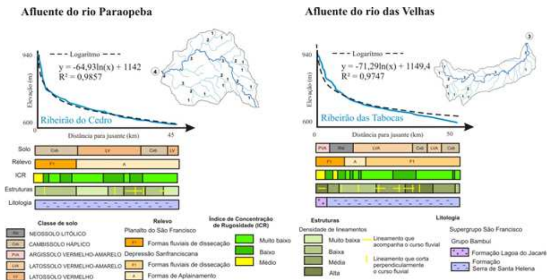
Figura 9: Perfis longitudinais cuja geometria se aproxima das condições de modelo ideal. Suas variáveis condicionantes, por sua vez, apresentam diferentes comportamentos
