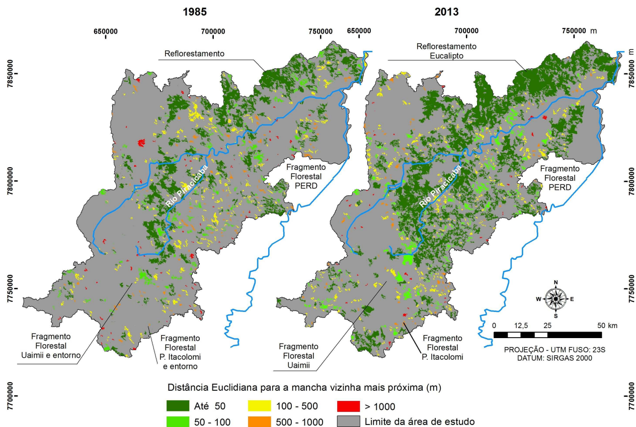
Figura 9 Mapas da distância euclidiana para o vizinho mais próximo – classe Reflorestamento: 1985 e 2013.
