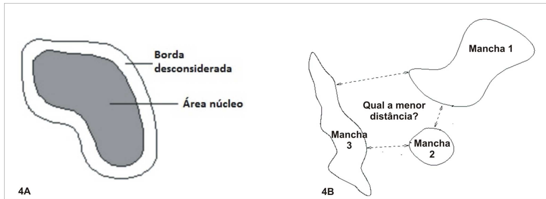
Figura 4 Esquema para cálculo das métricas no V-late: A) métrica da área núcleo; B) métrica do grau de isolamento.
