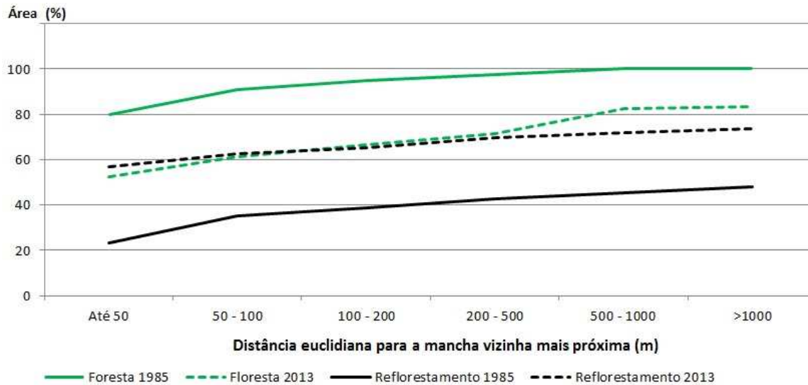
Figura 10 Porcentagem de área de manchas das classes Floresta e Reflorestamento por faixas de distância: 1985 e 2013
