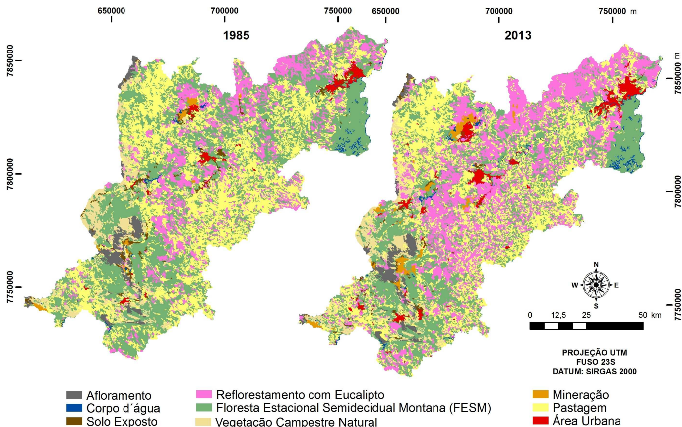
Figura 5 Mapeamentos da cobertura da terra: 1985 e 2013.
