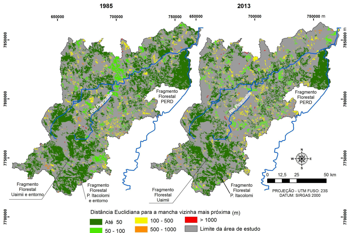
Figura 8 Mapas da distância euclidiana para o vizinho mais próximo – classe Floresta: 1985 e 2013.
