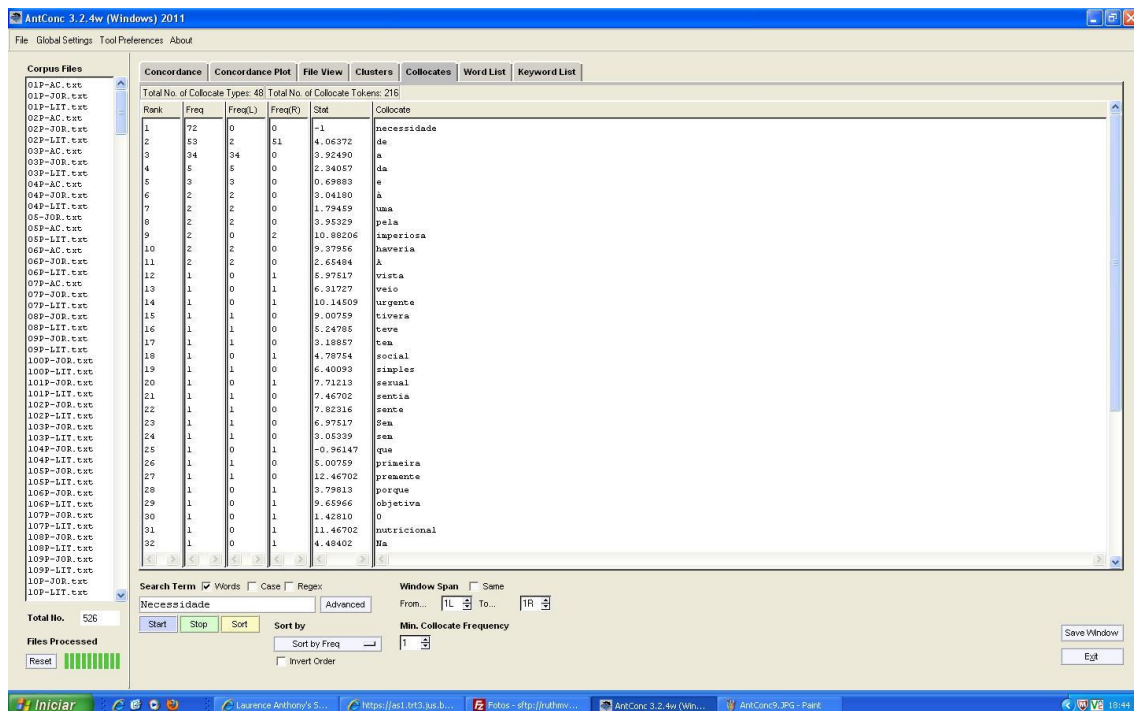
Figura 10: Tela do AntConc exibindo a palavra de busca e a lista de frequência de todos os itens lexicais que acompanham essa palavra à direita e à esquerda
