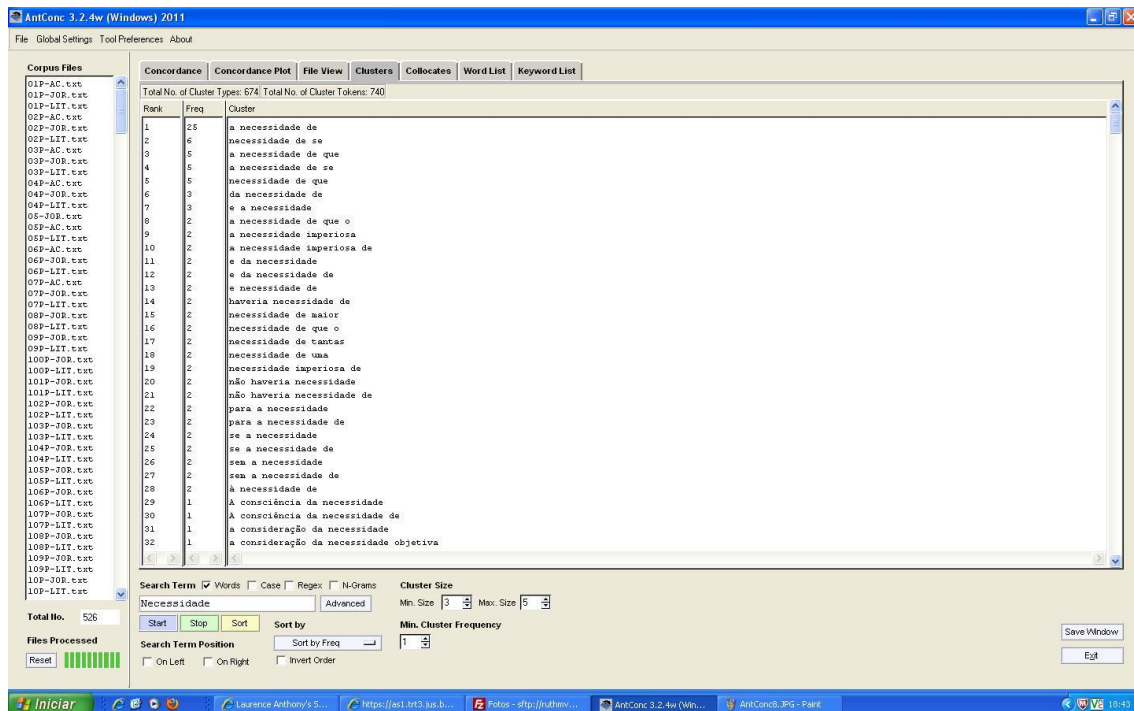
Figura 9: Tela do AntConc exibindo todos os agrupamentos de palavras em que a palavra de busca pode ser encontrada
