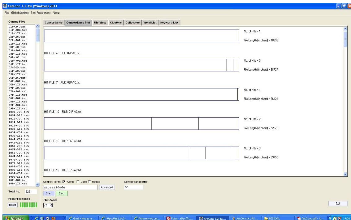
Figura 7: Tela do AntConc exibindo o número de vezes que a palavra de busca aparece em cada arquivo que compõe o corpus e em que parte do corpus ela está
