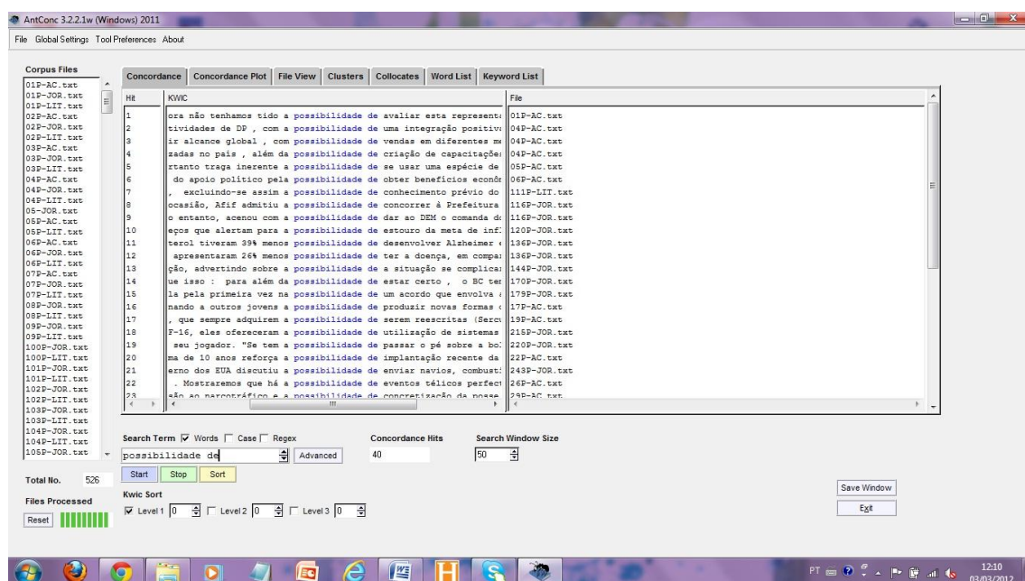
Figura 18: Tela do AntConc mostrando as linhas de concordância para a busca do lema Possibilidade + preposição de
