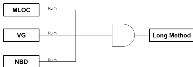
Figura 4.5. Estratégia de detecção para Long Method extraída de Souza [2016].
