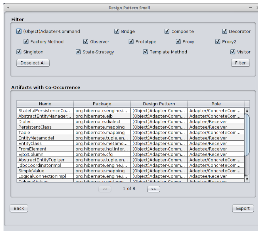
Figura 5.6. Tela para visualização dos artefatos afetados pelas coocorrências.
