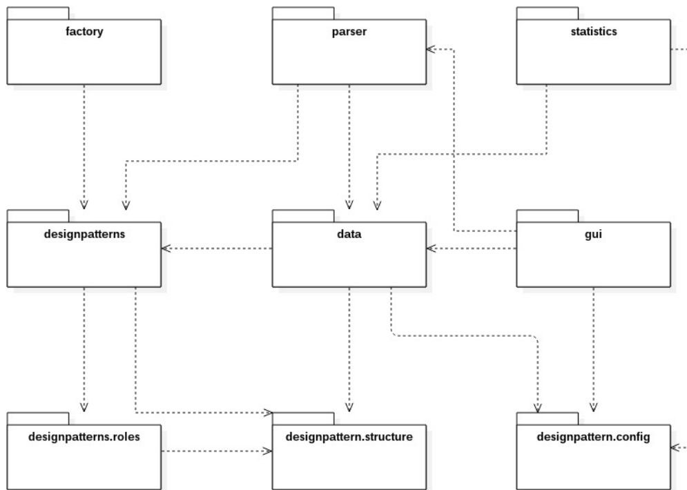
Figura 5.2. Diagrama de pacotes da ferramenta Design Pattern Smell .
