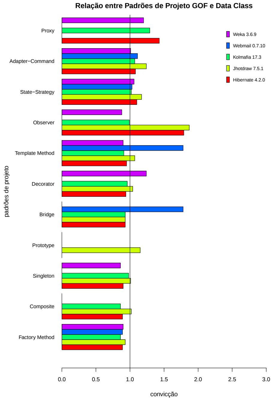
Figura 6.1. Resultado da associação (Padrão de Projeto \Rightarrow Data Class ).
