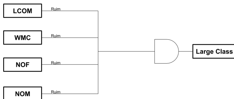
Figura 4.4. Estratégia de detecção para Large Class extraída de Souza [2016].
