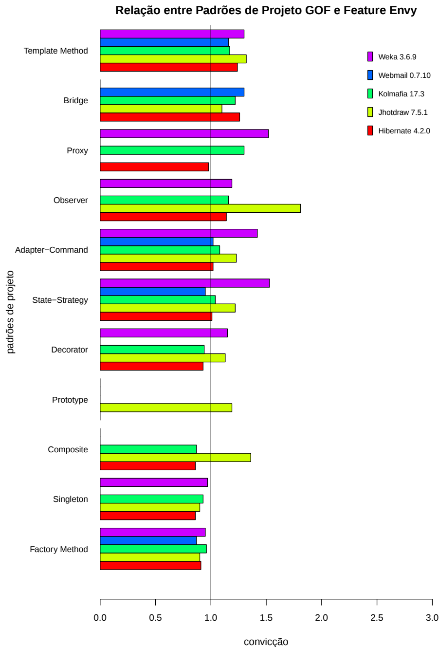
Figura 6.2. Resultado da associação (Padrão de Projeto \Rightarrow Feature Envy ).
