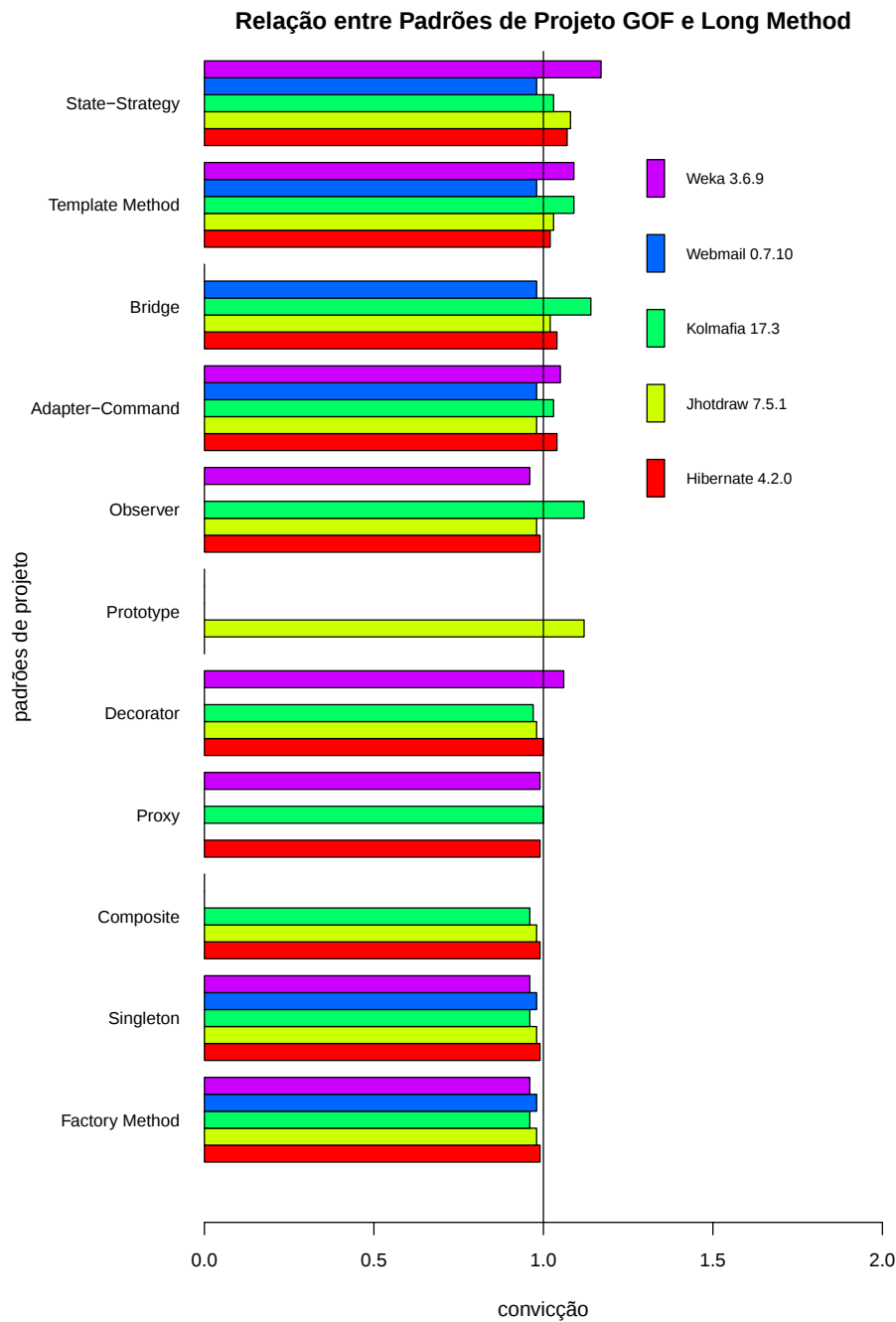
Figura 6.4. Resultado da associação (Padrão de Projeto \Rightarrow Long Method).
