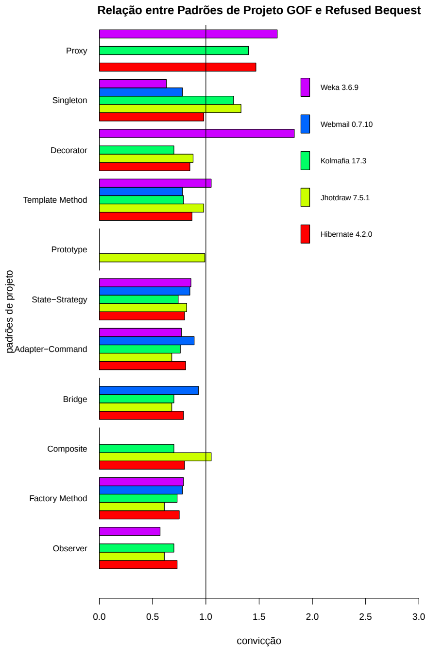
Figura 6.5. Resultado da associação (Padrão de Projeto \Rightarrow Refused Bequest ).
