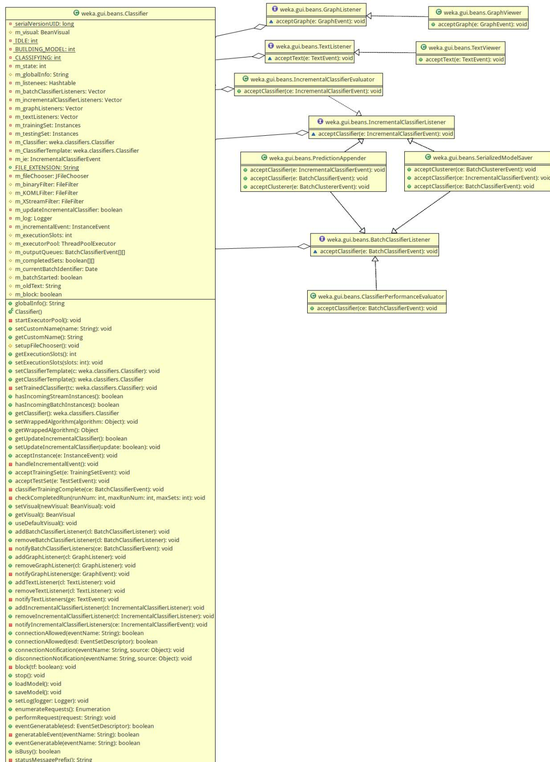
Figura 6.8. Diagrama de Classes que representa a relação Observer \Rightarrow Large Class .
