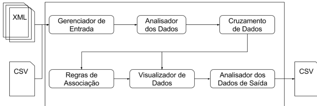
Figura 5.1. Arquitetura da Design Pattern Smell Architecture .
