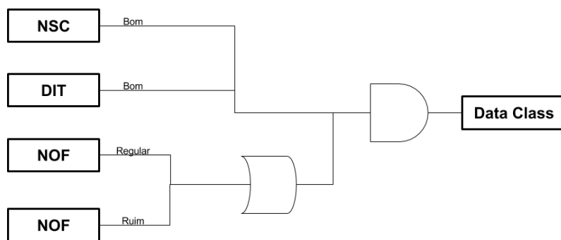
Figura 4.2. Estratégia de detecção para Data Class extraída de Souza [2016].
