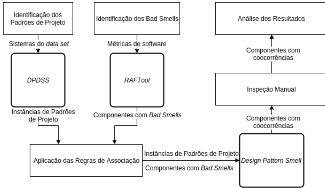
Figura 4.7. Método de análise dos resultados.
