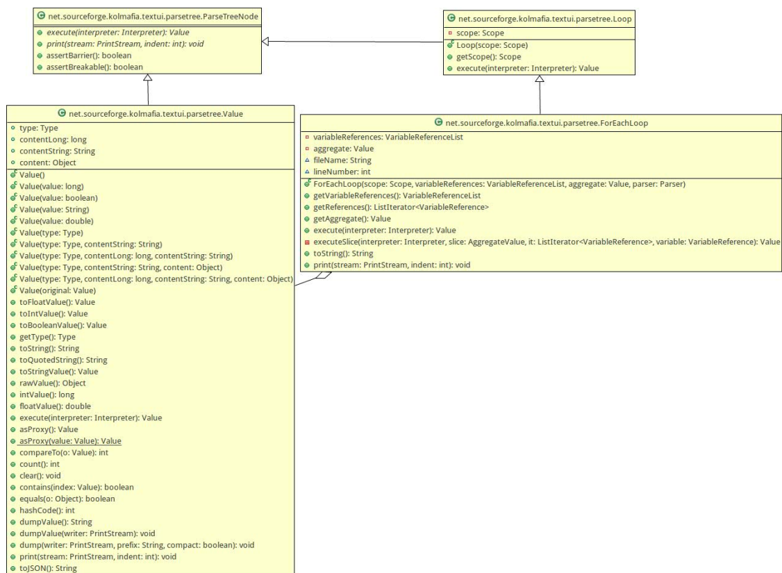
Figura 6.10. Diagrama de Classes que representa a relação Proxy \Rightarrow Refused Bequest .
