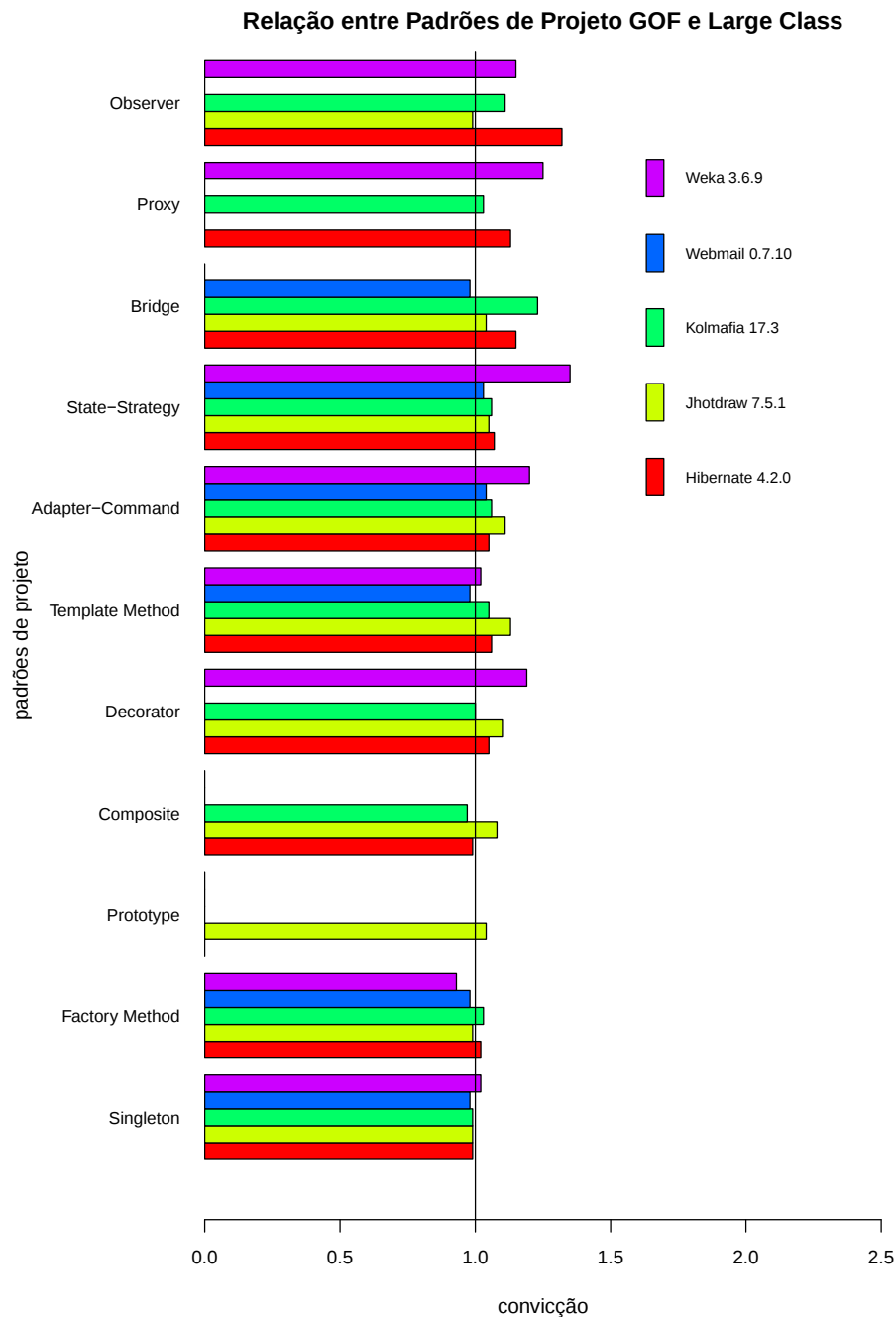
Figura 6.3. Resultado da associação (Padrão de Projeto \Rightarrow Large Class ).
