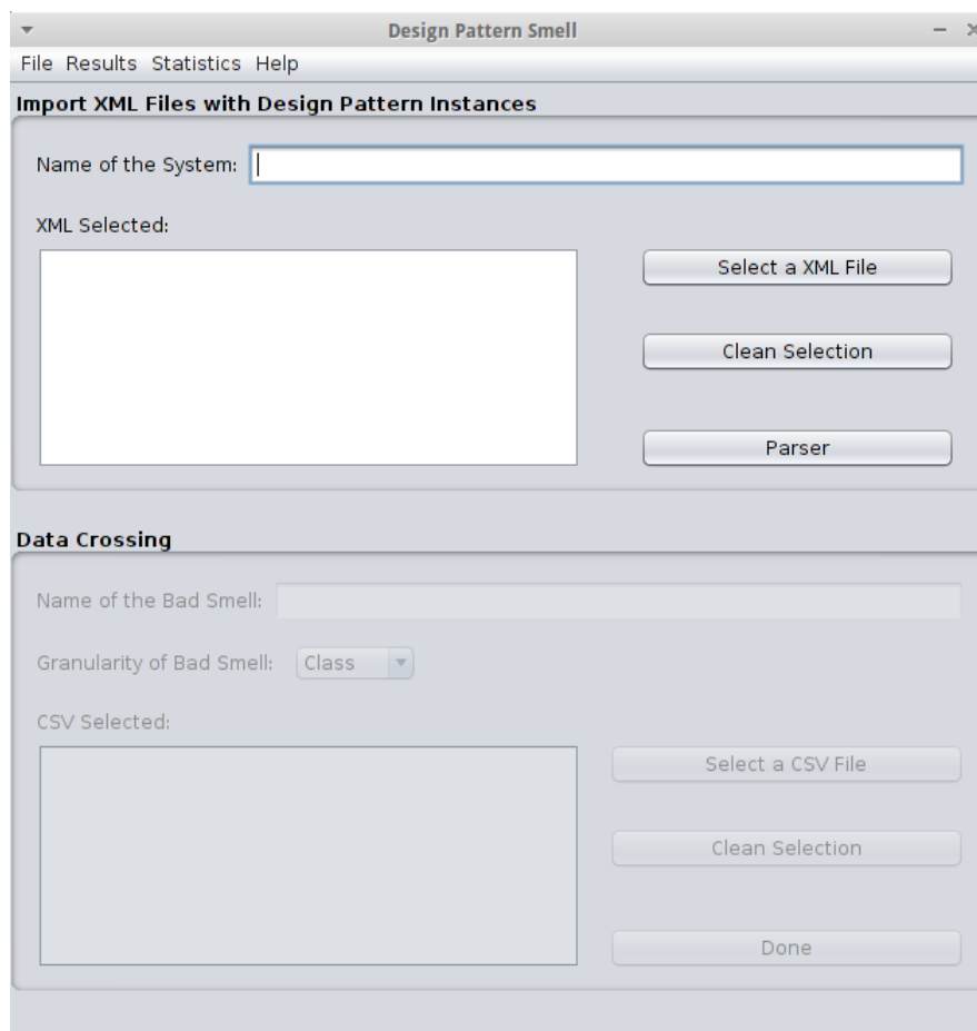
Figura 5.3. Tela principal para importação dos arquivos XML e CSV.
