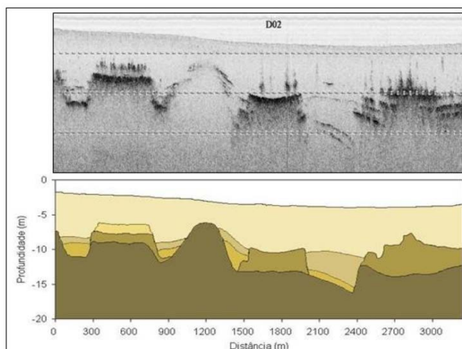
Figura 2. Perfil sísmico
