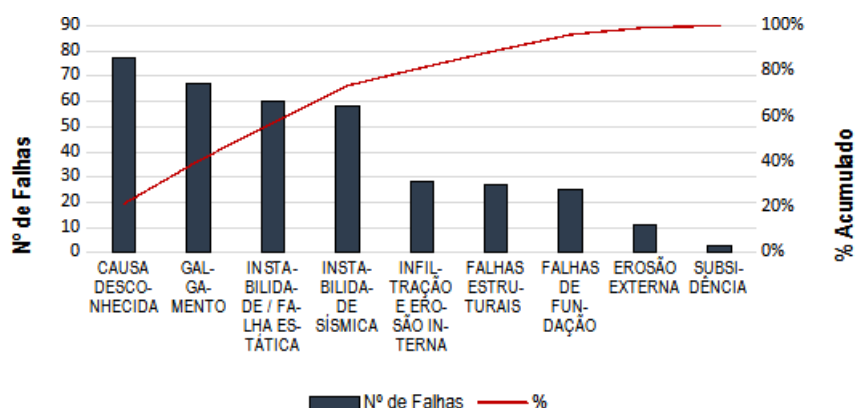
Gráfico 7 - Diagrama de Pareto para os tipos de causas relativos ao número de rompimento, baseado nos 356 registros na base WMTF, normatizados com descrições para causas do evento
