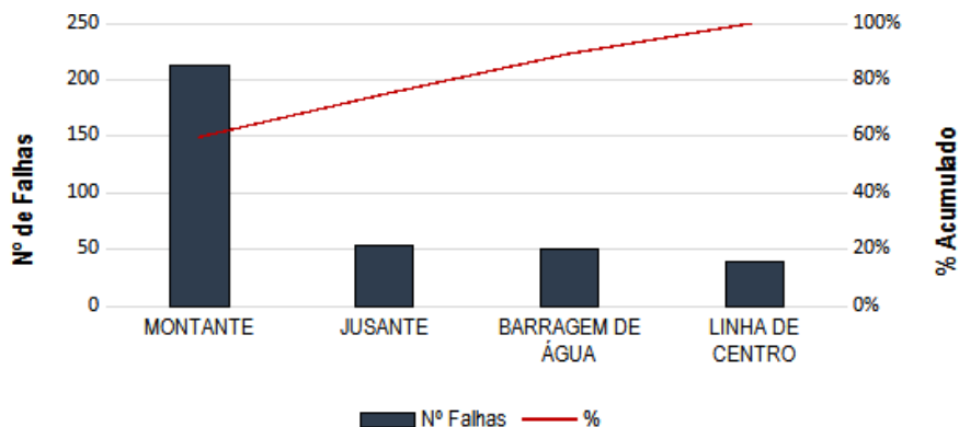
Gráfico 8 - Diagrama de Pareto para os tipos de alteamento relativos ao número de rompimento, baseado nos 356 registros na base WMTF, normatizados com descrições para causas do evento
