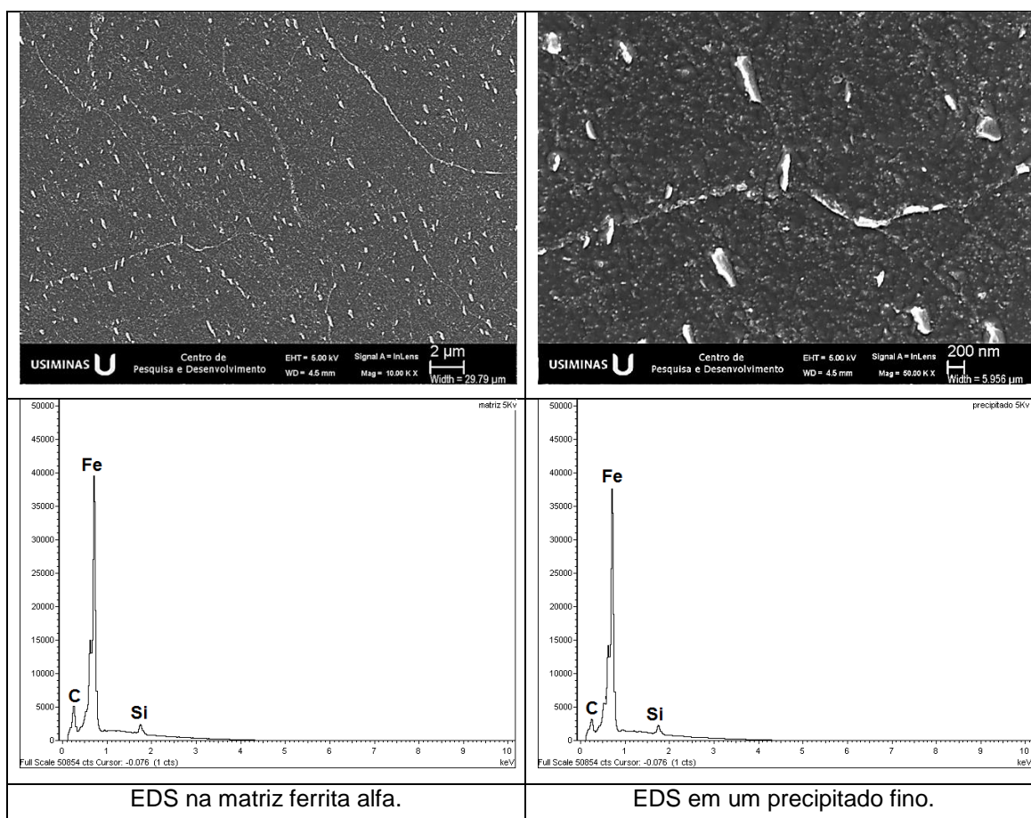
FIGURA V.23 – MEV e EDS realizados na GGZAC do aço SAC 2, para análise dos precipitados finos – pf.
