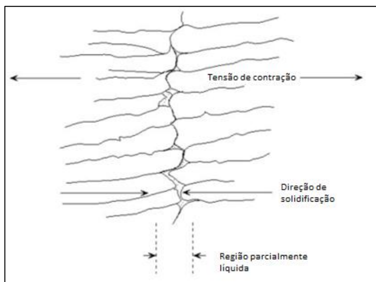
FIGURA III.8 – Trinca de solidificação (25) .
