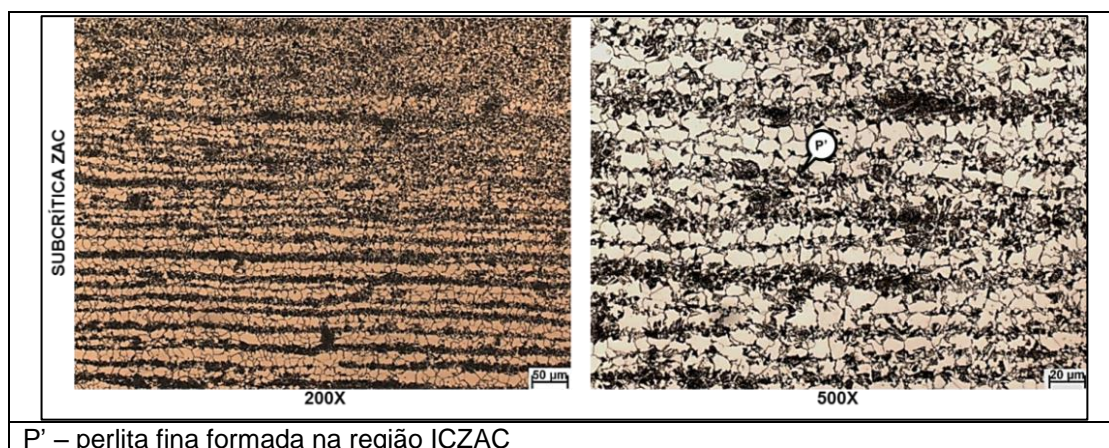
FIGURA V.18 – Região ICZAC do aço SAC 1 com baixo aporte de calor.
