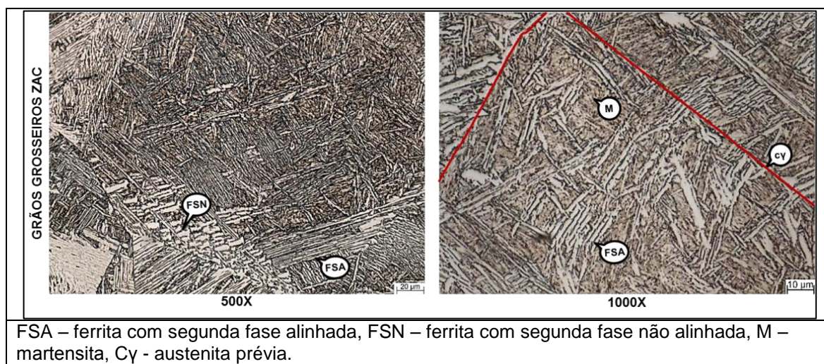
FIGURA V.15 – Região GGZAC do aço SAC 1 com alto aporte de calor.
