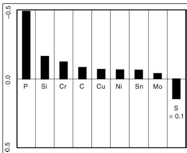
FIGURA III.2 – Efeito dos elementos químicos na taxa de corrosão atmosférica (7) .
