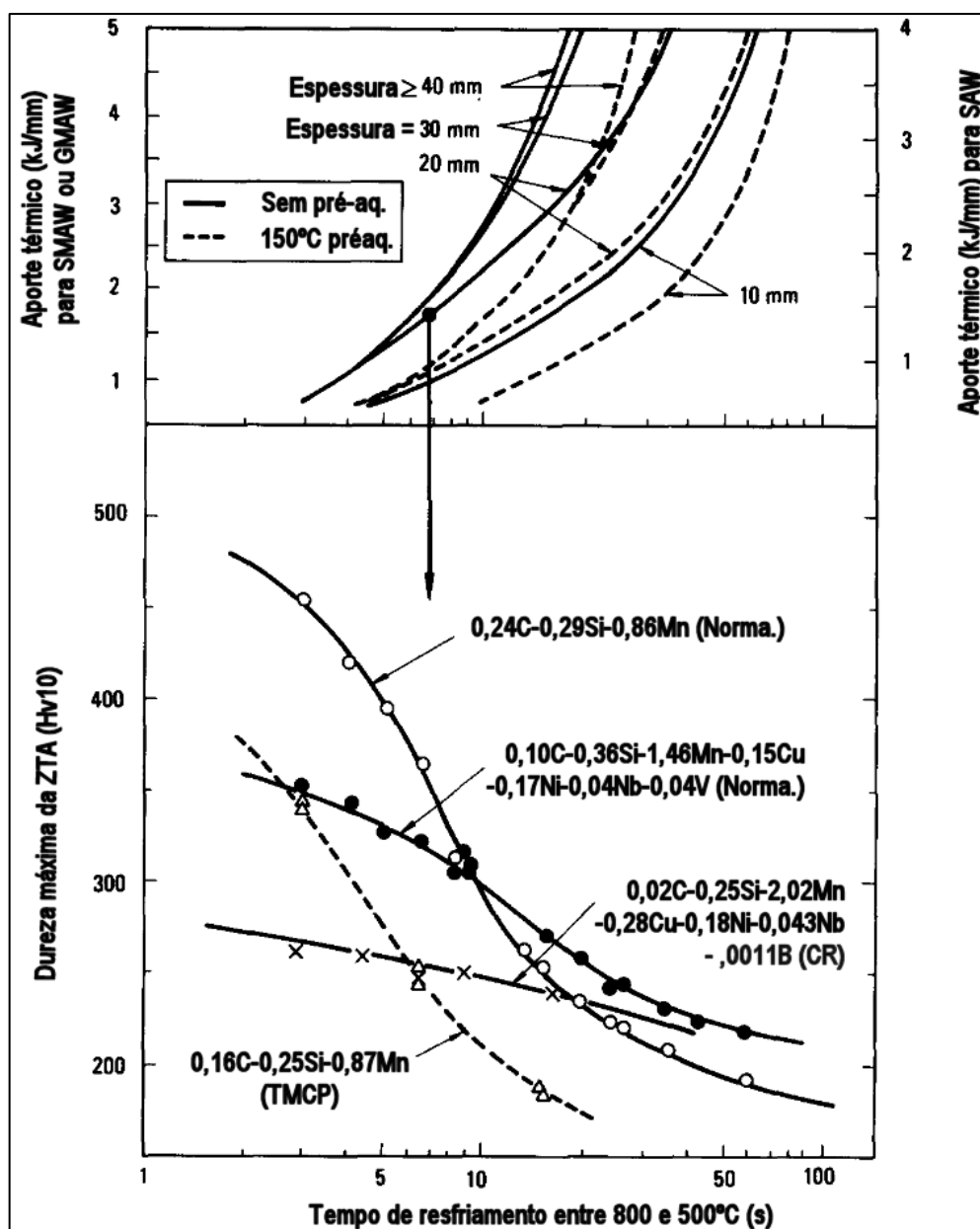
FIGURA III.7 – Mudança nos valores de dureza de vários tipos de aço com respeito ao tempo de resfriamento da solda. Adaptado de Yurioka (24) .
