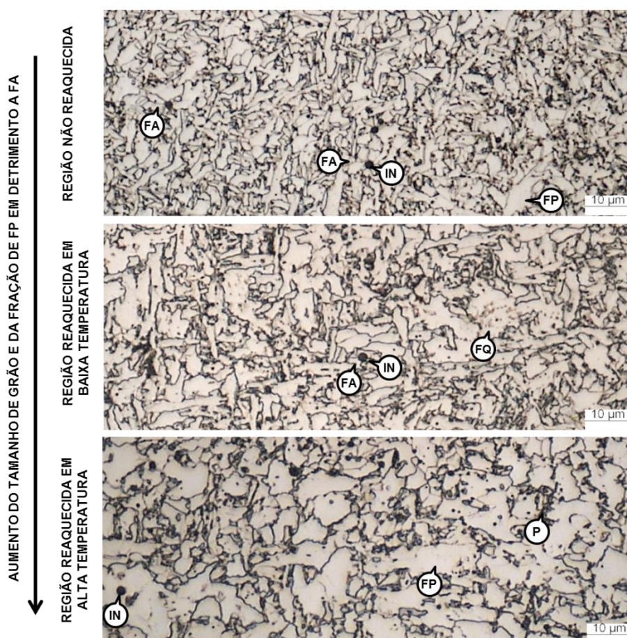
FIGURA V.13 – Diferentes regiões do metal de solda evidenciando os microconstituintes FA, FP, FQ e IN.
