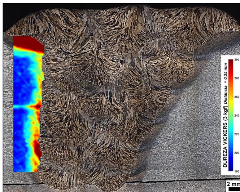
FIGURA V.39 – Mapeamento de dureza da ZAC do aço SAC 1 com AAC.
