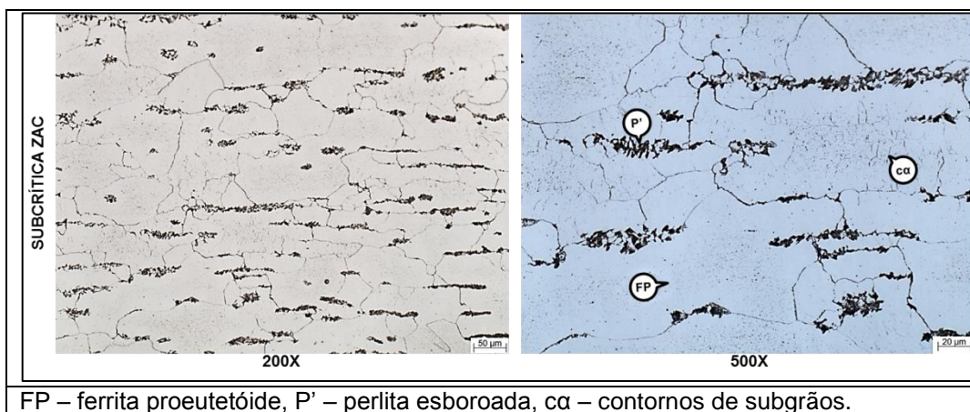
FIGURA V.31 – Região SCZAC do aço SAC 2 com alto aporte de calor.
