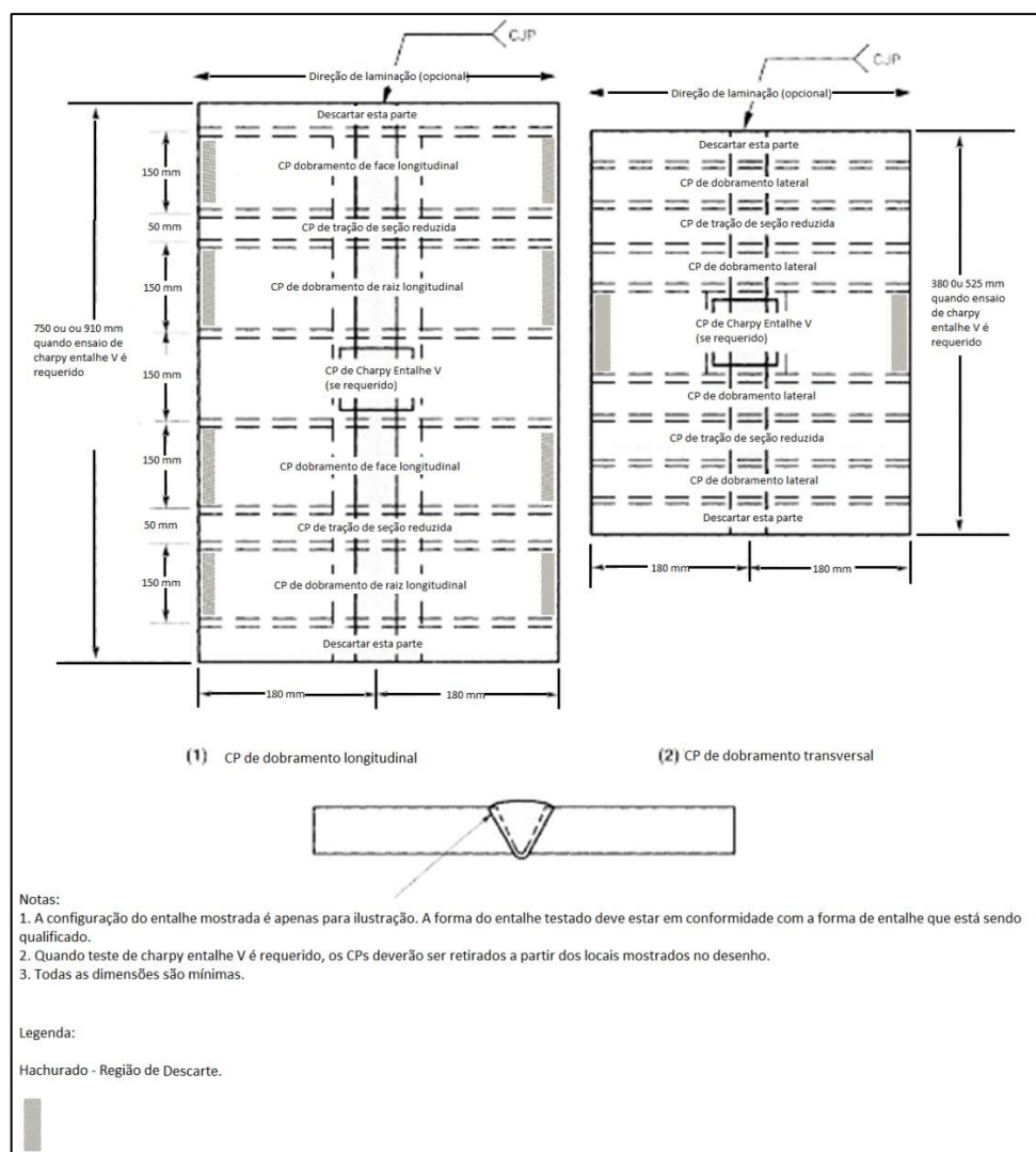
FIGURA IV.3 – Desenho esquemático para retirada dos CPs para os ensaios mecânicos das juntas soldadas. Adaptado de AWS (14) .
