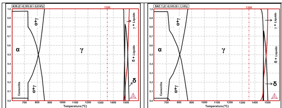
FIGURA V.6 – Fração molar das diferentes fases formadas durante o resfriamento dos aços ASTM A36 e SAC 1.
