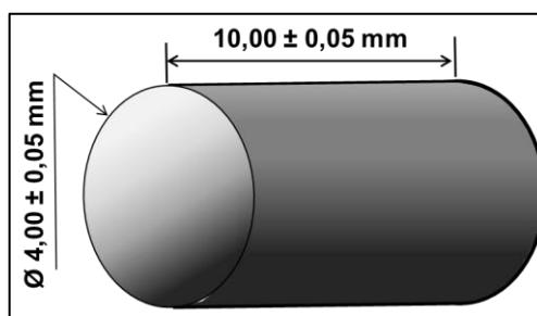
FIGURA IV.8 – Desenho esquemático do CP para ensaio de simulação dilatométrica.
