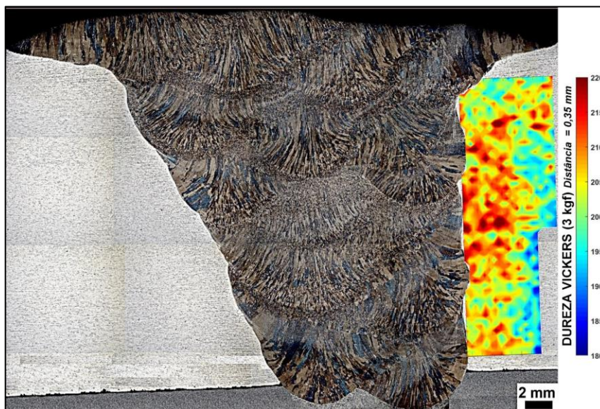
FIGURA V.38 – Mapeamento de dureza da ZAC do aço SAC2 com BAC.
