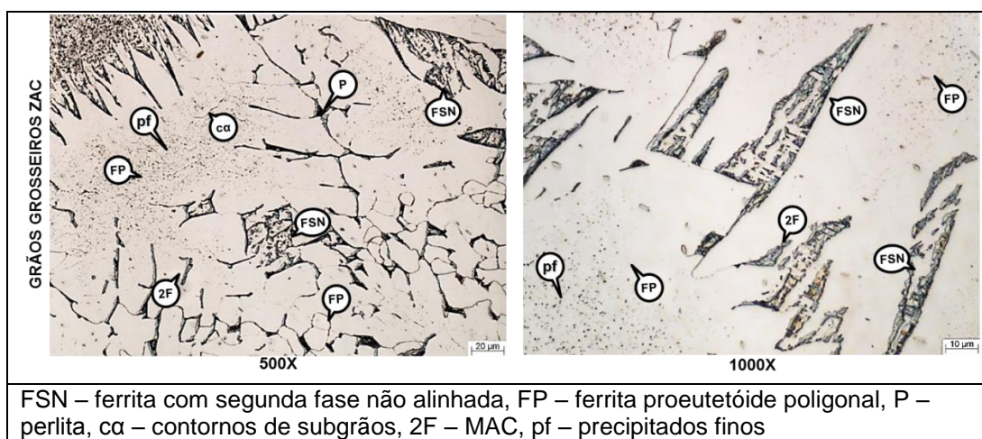
FIGURA V.21 – Região GGZAC do aço SAC 2 com baixo aporte de calor.
