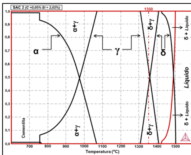
FIGURA V.5 – Fração molar das diferentes fases formadas durante o resfriamento do aço SAC 2 no equilíbrio e diagrama de equilíbrio evidenciando a região de formação de ferrita delta.
