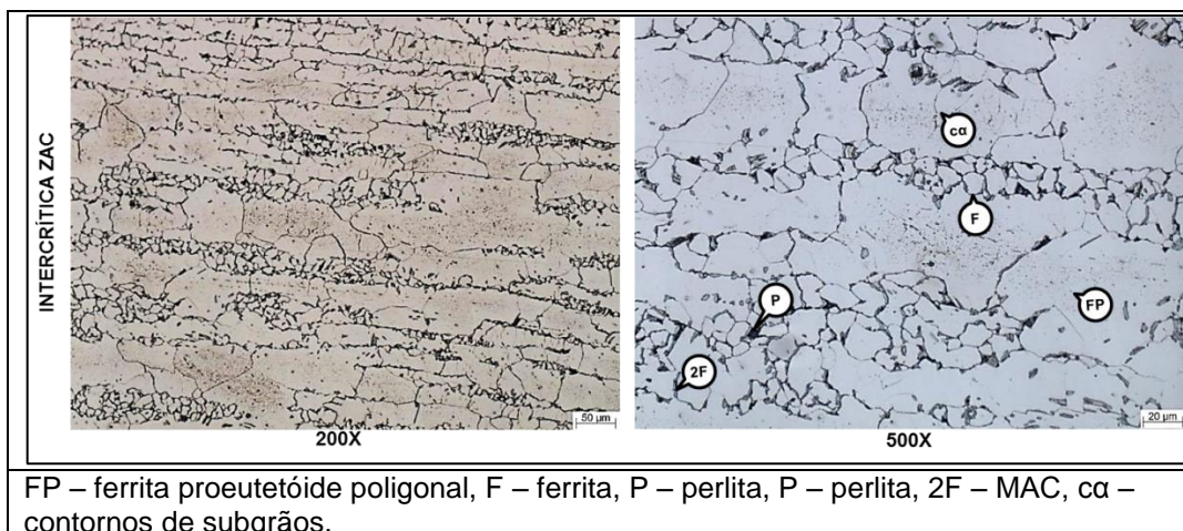
FIGURA V.28 – Região ICZAC do aço SAC 2 com baixo aporte de calor.
