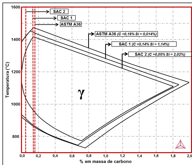
FIGURA V.7 – Influência do silício (SAC 2) na extensão do campo austenítico ( \gamma ).
