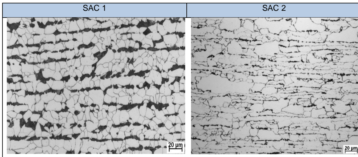
FIGURA V.1 – Microestrutura dos aços SAC 1 e SAC 2.
