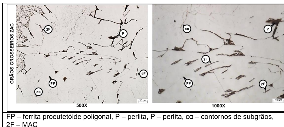
FIGURA V.22 – Região GGZAC do aço SAC 2 com alto aporte de calor.
