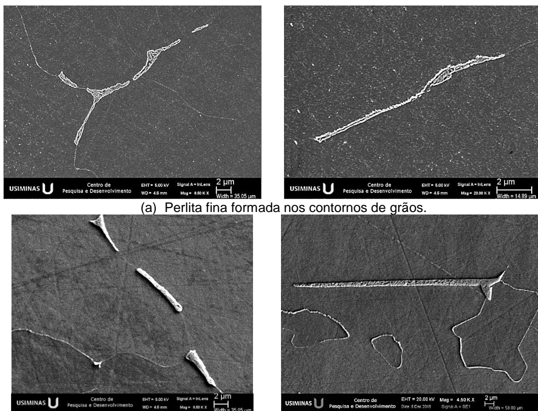
(b) Segunda fase nos contornos da austenita previa possivelmente ferrita delta.
