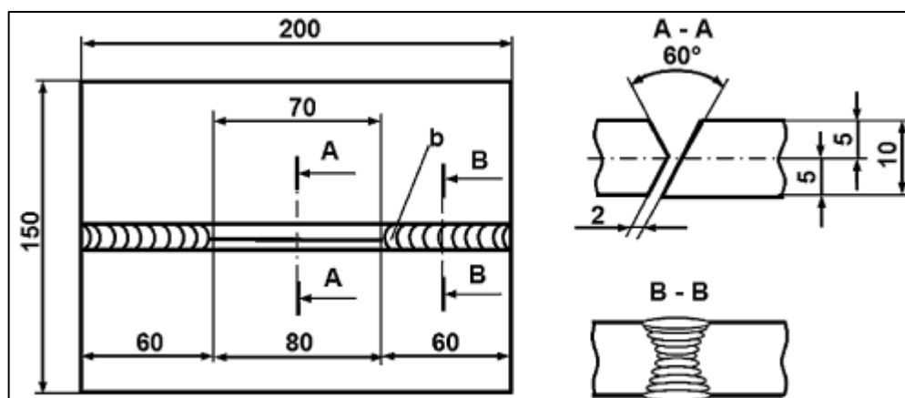
FIGURA IV.1 – Desenho esquemático do corpo de prova para o ensaio Tekken (33) .
