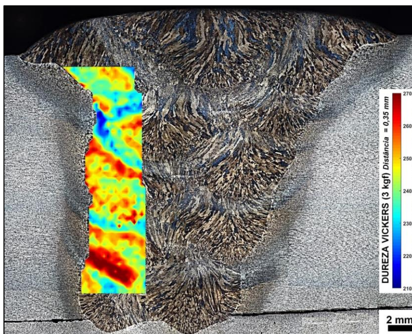
FIGURA V.35 – Mapeamento de dureza do metal de solda do aço SAC 1 com AAC.
