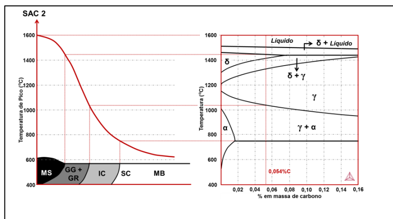
FIGURA V.8 – Regiões da ZAC em função do diagrama de equilíbrio do aço SAC 2.
