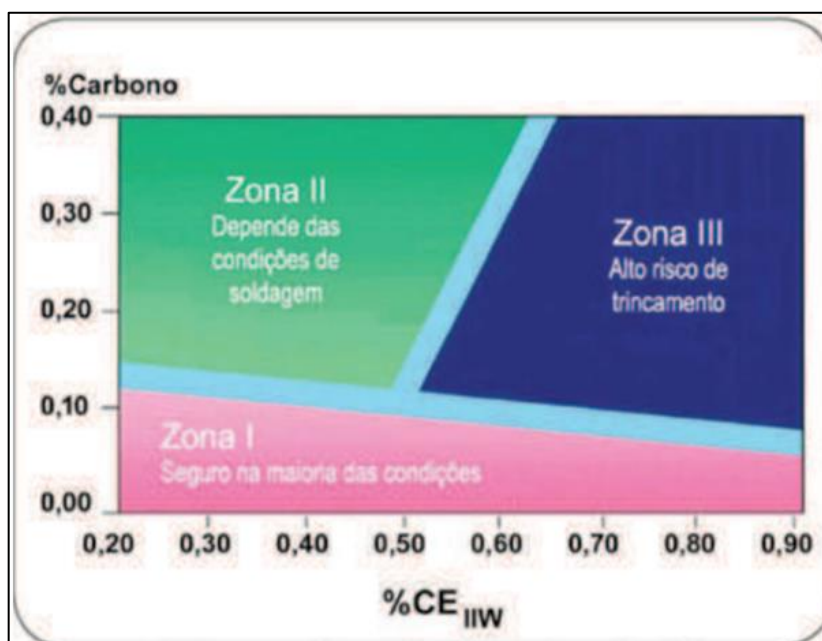
FIGURA III.4 - Diagrama de Graville ilustrando o vínculo entre a soldabilidade de um aço com sua composição química. Adaptado de Graville (17) .
