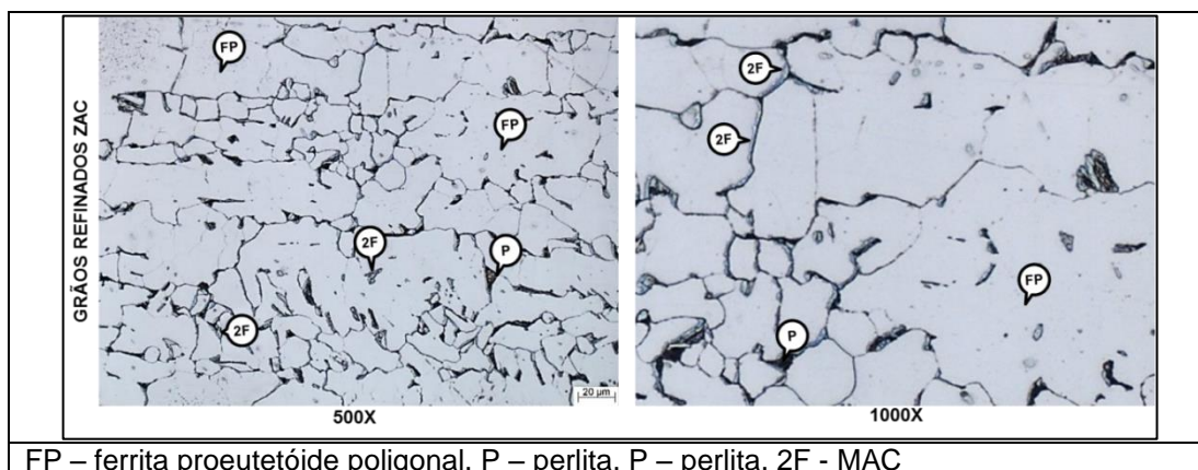
FIGURA V.26 – Região GRZAC do aço SAC 2 com baixo aporte de calor.
