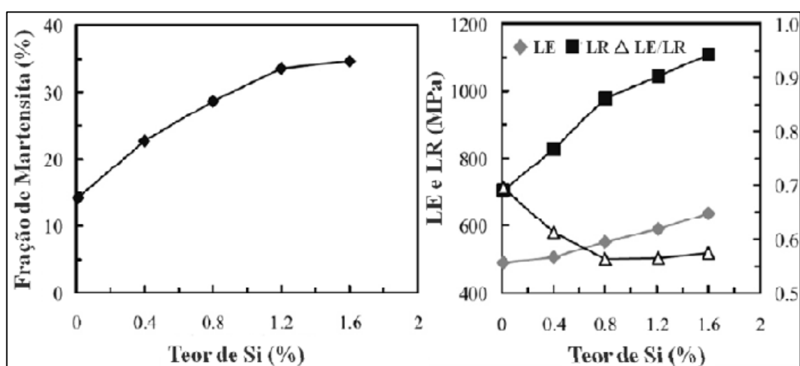
FIGURA III.5 – Efeito do teor de Si na fração volumétrica de martensita e nas propriedades mecânicas de um aço C-Mn (21) .
