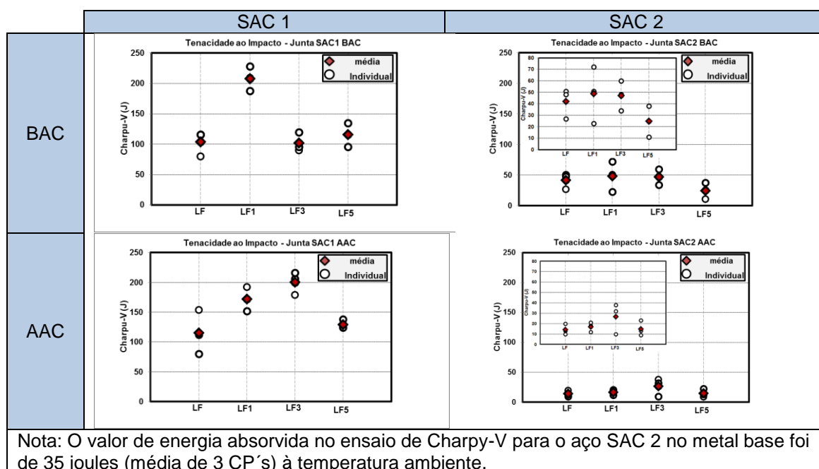
FIGURA V.41 – Resultados de tenacidade ao impacto dos aços SAC 1 e SAC 2, com BAC e AAC.
