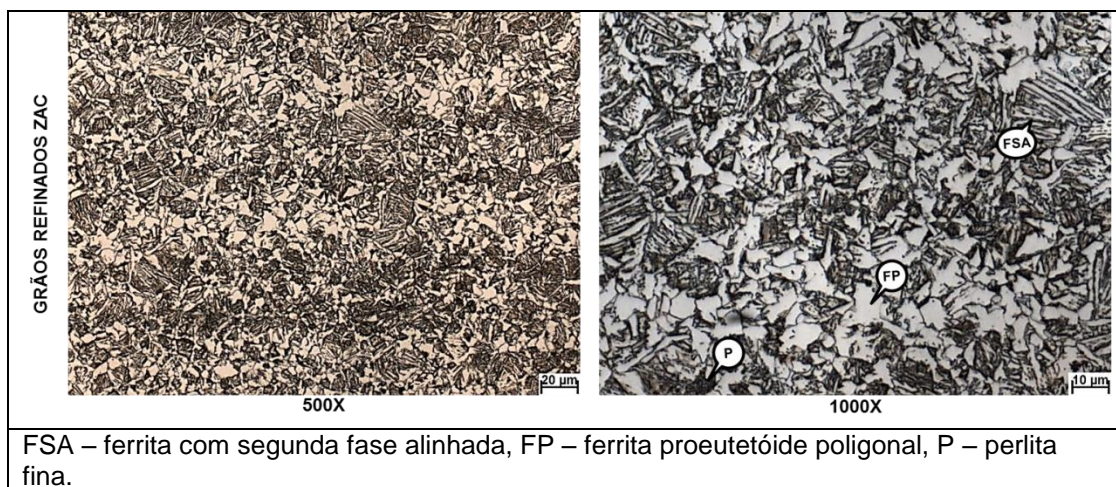
FIGURA V.16 – Região GRZAC do aço SAC 1 com baixo aporte de calor.
