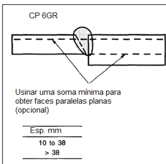
FIGURA IV.7 – Desenho esquemático do CP de dobramento lateral. Adaptado de AWS (14) .
