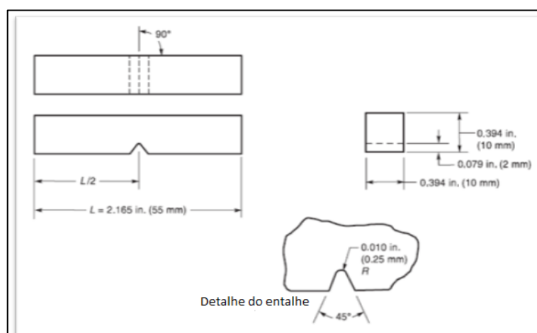
FIGURA IV.6– Desenho esquemático do dimensional dos corpos de prova de Charpy. Adaptado de AWS (13) .
