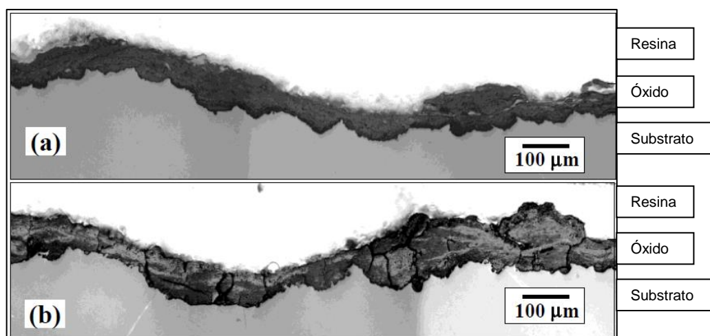
FIGURA III.3 – (a) Seção transversal de uma camada de óxido formada em um aço patinável por 32 anos e (b) de um aço baixo carbono exposto por 15 anos, por luz polarizada (11) .
