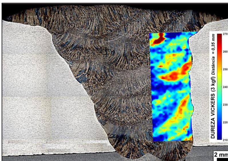
FIGURA V.34 – Mapeamento de dureza do metal de solda do aço SAC 2 com BAC.
