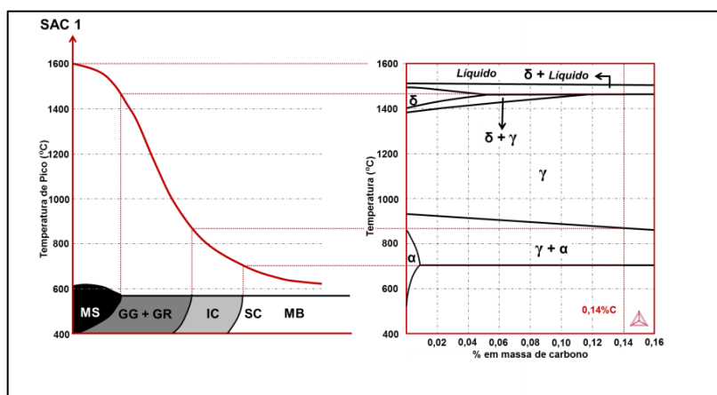
FIGURA V.9 – Regiões da ZAC em função do diagrama de equilíbrio do aço SAC 1.
