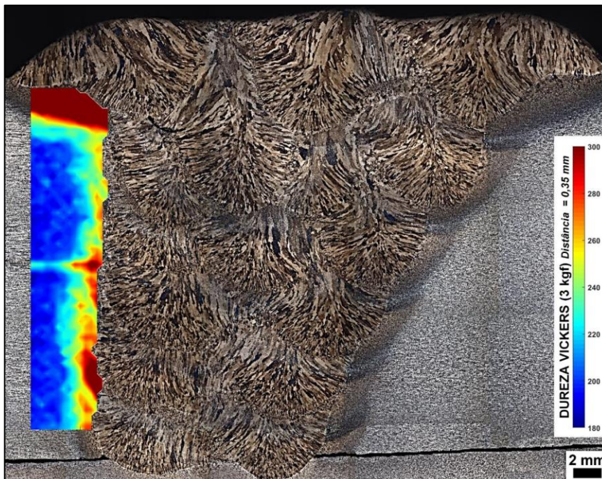
FIGURA V.37 – Mapeamento de dureza da ZAC do aço SAC 1 com BAC.
