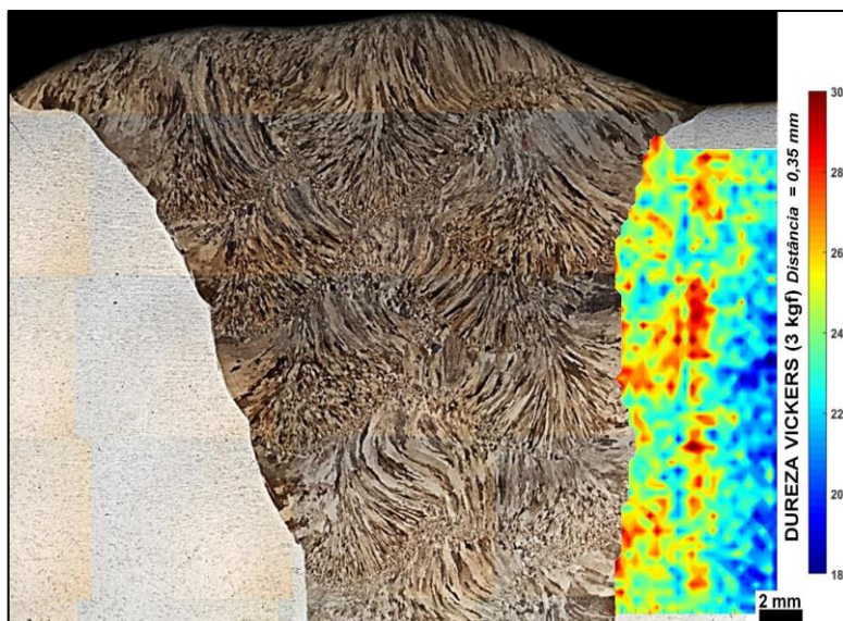
FIGURA V.40 – Mapeamento de dureza da ZAC do aço SAC 2 com AAC.
