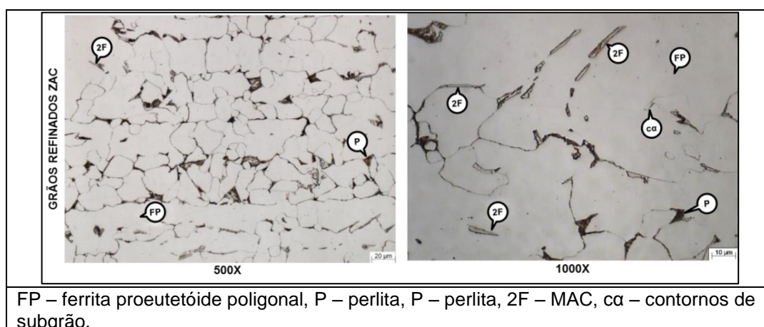
FIGURA V.27 – Região GRZAC do aço SAC 2 com alto aporte de calor.
