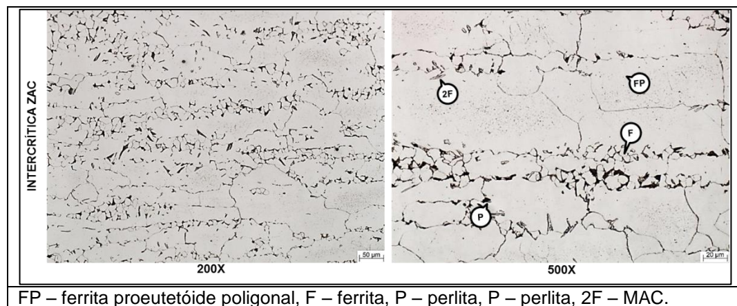
FIGURA V.29 – Região ICZAC do aço SAC 2 com alto aporte de calor.
