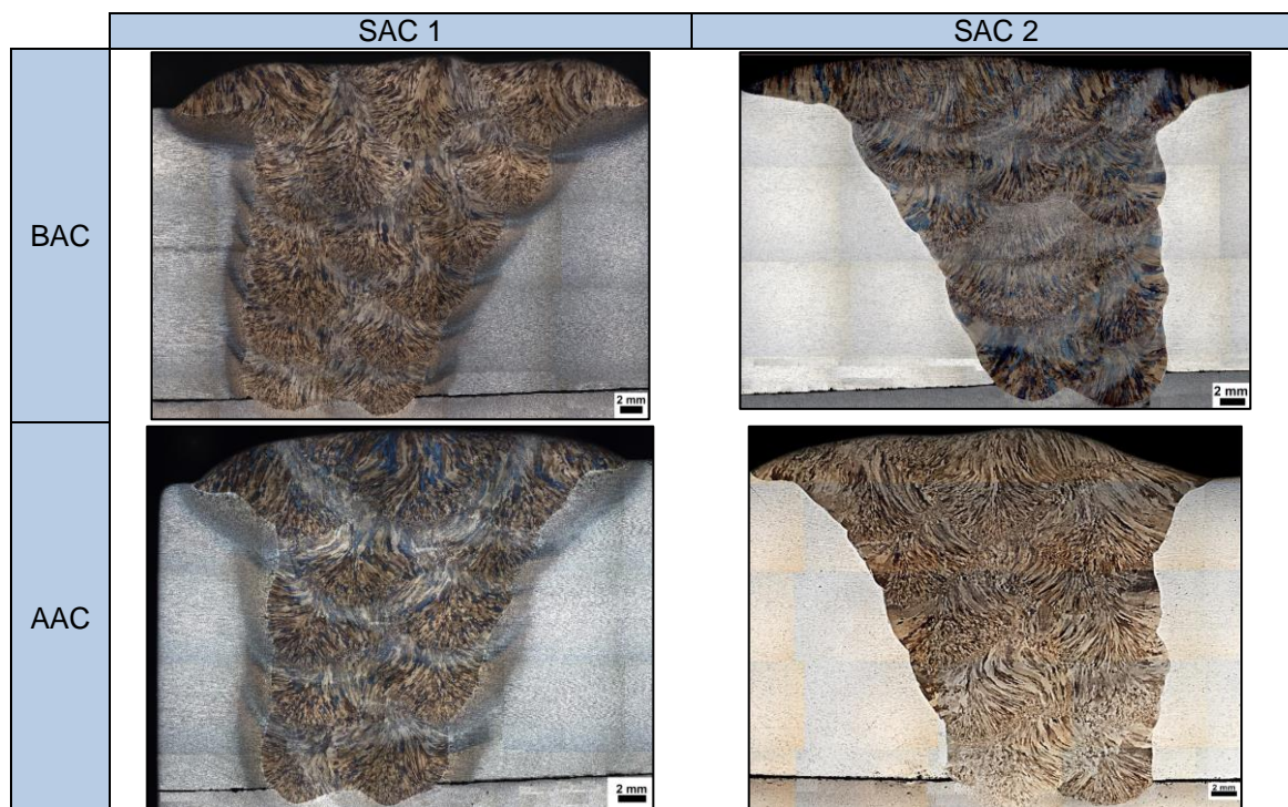
FIGURA V.12 – Aspecto macroestrutural da junta soldada dos aços SAC 1 e SAC 2 com BAC e AAC.
