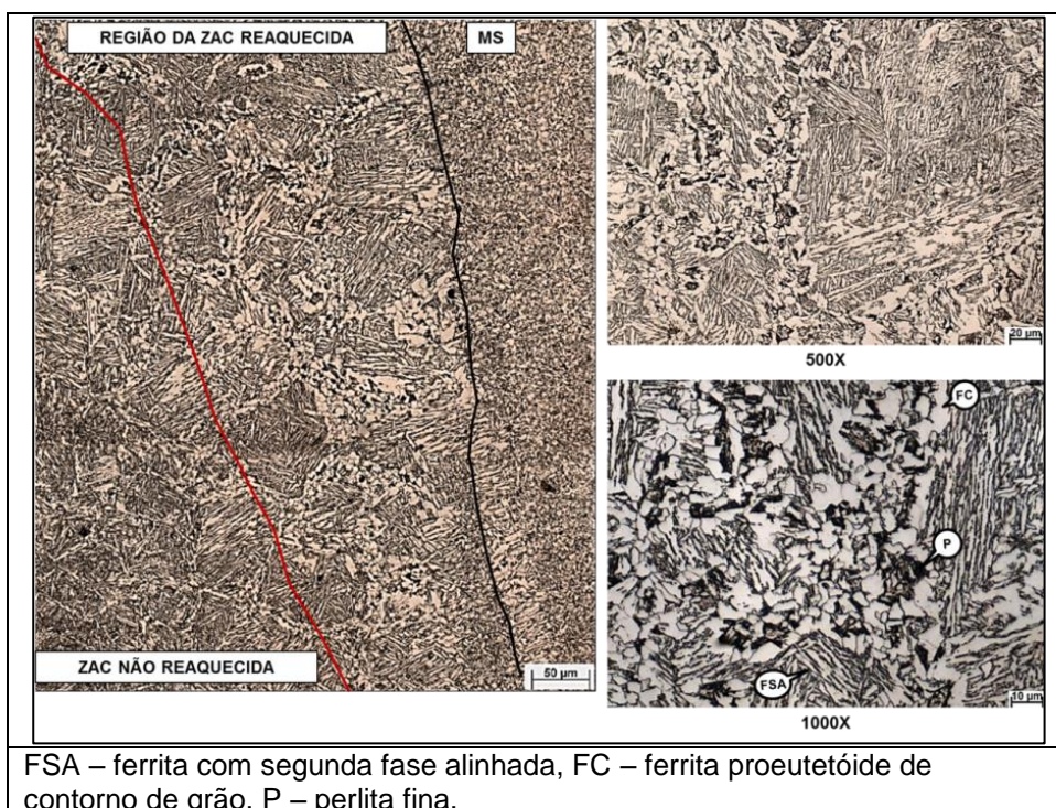
FIGURA V.20 – Região reaquescida da ZAC do aço SAC 1 com baixo aporte de calor.
