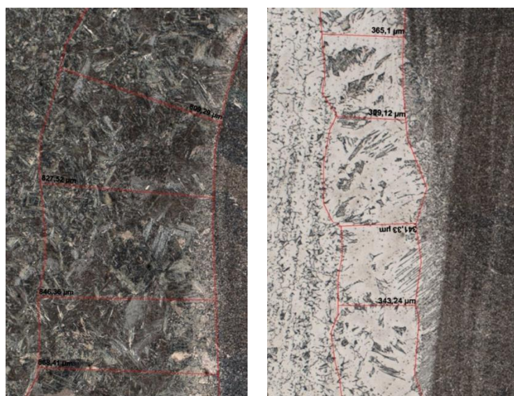
FIGURA V.32 – Medição da região GGZAC dos aços SAC 1 e SAC 2.
