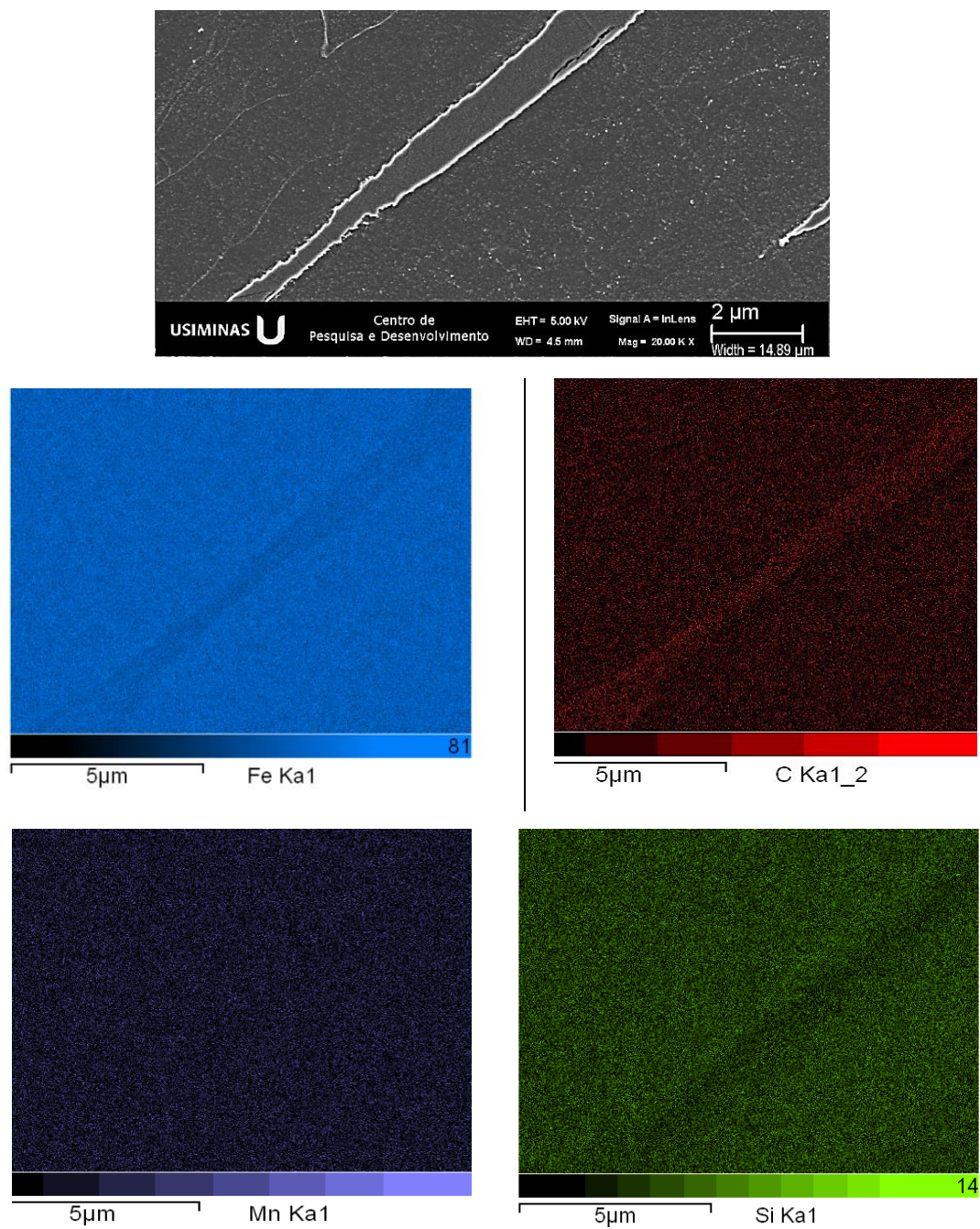
FIGURA V.25 – Mapeamento de EDS em uma segunda fase na forma de agulha.
