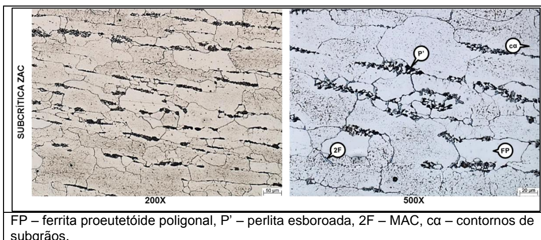
FIGURA V.30 – Região SCZAC do aço SAC 2 com baixo aporte de calor.
