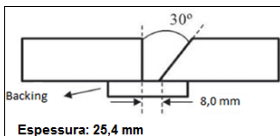
FIGURA IV.2 – Desenho esquemático para chanfro de soldagem.
