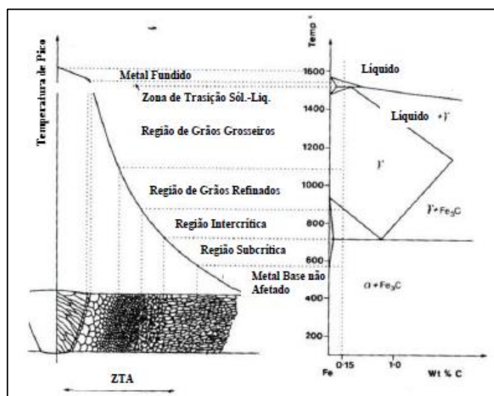
FIGURA III.6 – Diagrama esquemático das várias regiões da ZAC. Adaptado de Lippold (16) .
