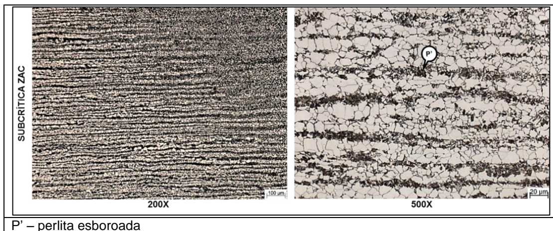
FIGURA V.19 – Região ICZAC do aço SAC 1 com alto aporte de calor.
