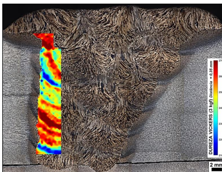
FIGURA V.33 – Mapeamento de dureza do metal de solda do aço SAC 1 com BAC.
