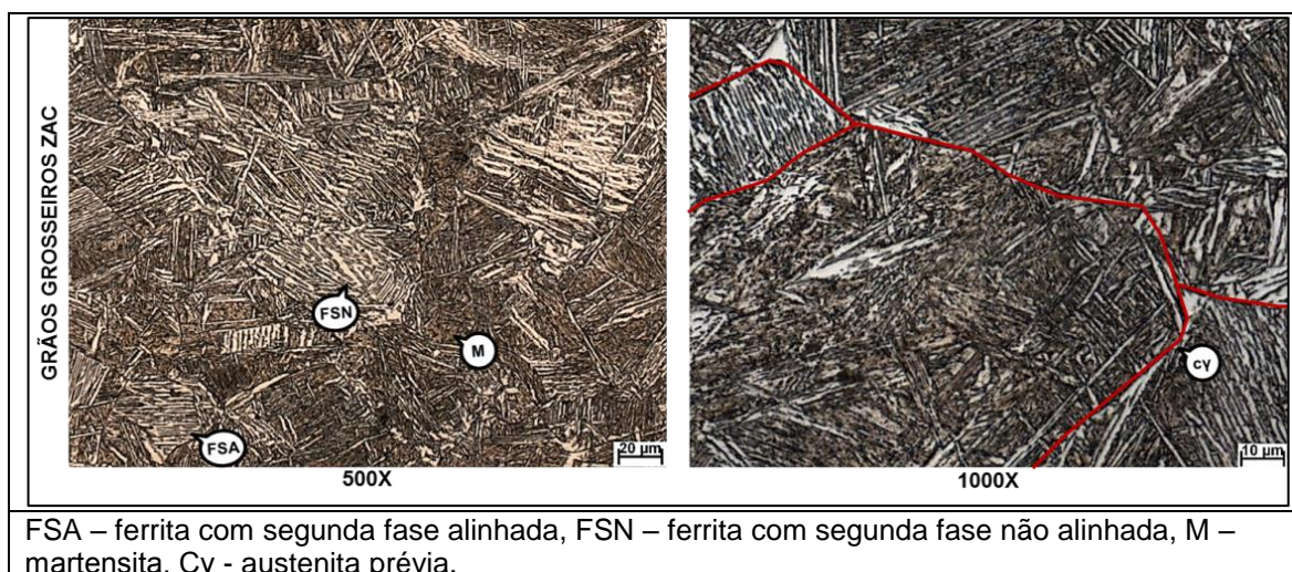
FIGURA V.14 – Região GGZAC do aço SAC 1 com baixo aporte de calor.
