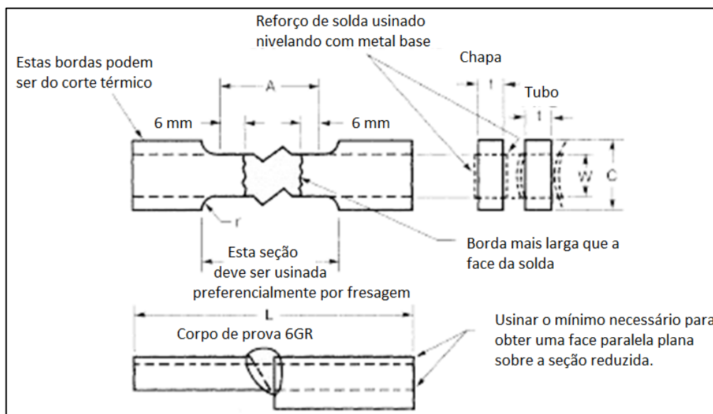
FIGURA IV.4 – Corpo de prova retangular para ensaio de tração (14) .
