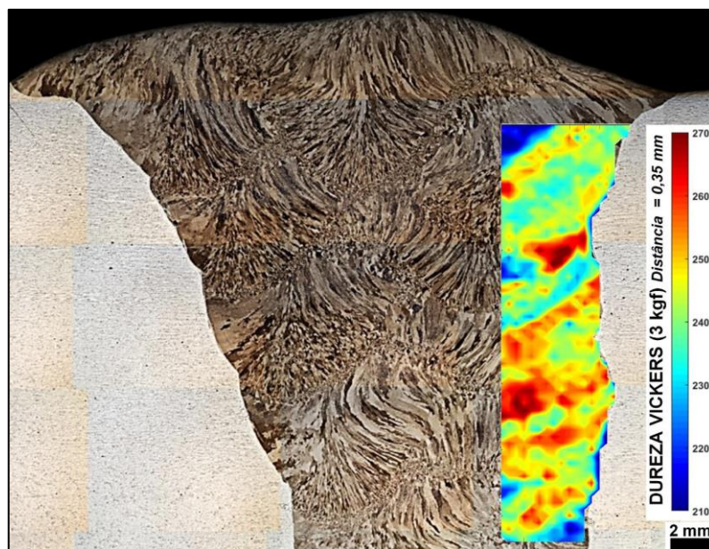
FIGURA V.36 – Mapeamento de dureza do metal de solda do aço SAC 2 AAC.
