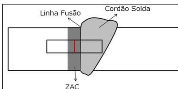
FIGURA IV.5 – Desenho esquemático do corpo de prova de Charpy na junta soldada (41) .
