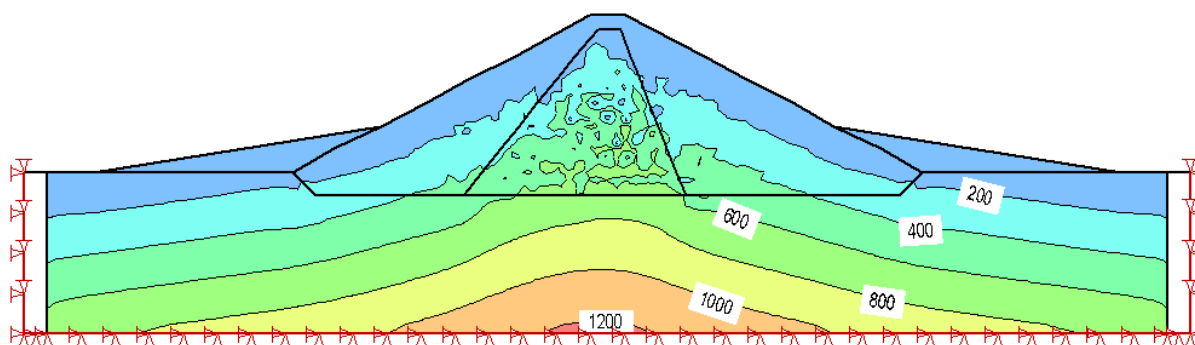
Figura 4.12: Tensões verticais 2 – margem esquerda (valores em kPa)
