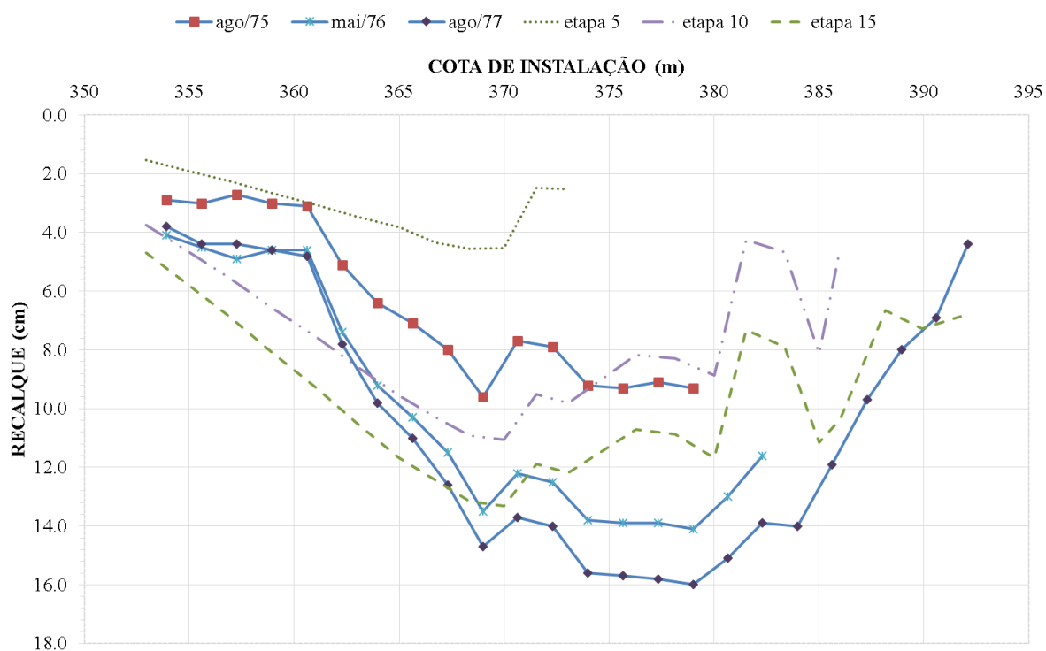
Figura 4.40: Comparação 3 entre os recalques do modelo com o instrumento SSMDIR300
