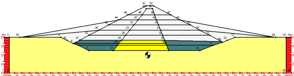
Figura 3.17: Etapa 4 da barragem da margem direita
