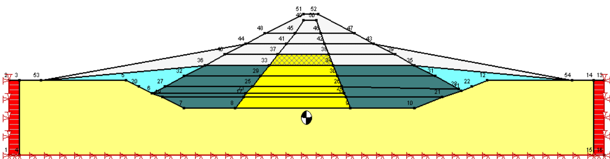
Figura 3.22: Etapa 9 da barragem da margem direita
