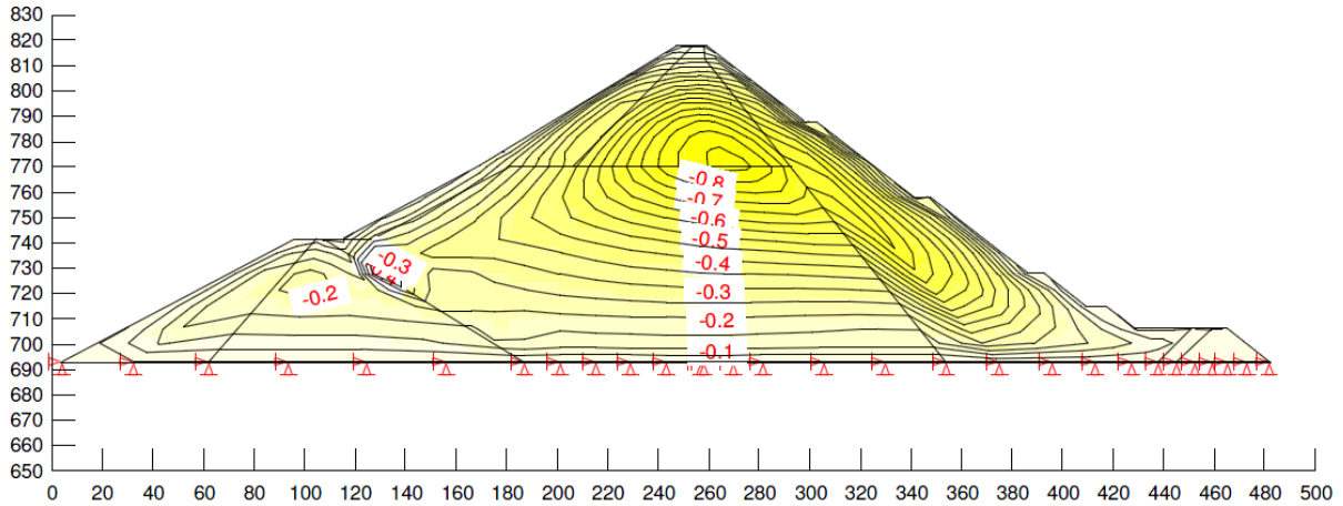
Figura 2.19: Deslocamentos verticais para UHE Nova Ponte – Caso 1 (MUSMAM, 2002)
