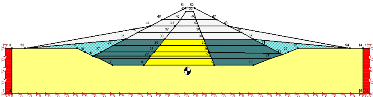
Figura 3.21: Etapa 8 da barragem da margem direita
