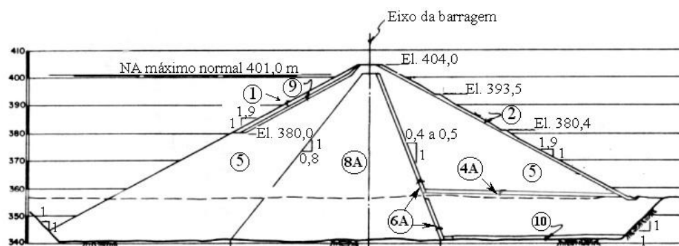
Figura 3.4: Barragem de terra da margem direita da UHE de São Simão (FONSECA, 2003)
