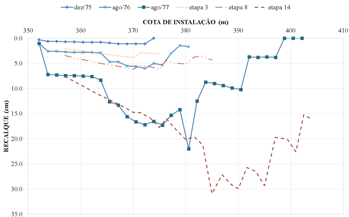
Figura 4.13: Comparação 2 entre os recalques do modelo com o instrumento SSMEIR100
