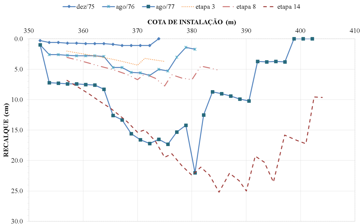
Figura 4.27: Comparação 3 entre os recalques do modelo com o instrumento SSMEIR100
