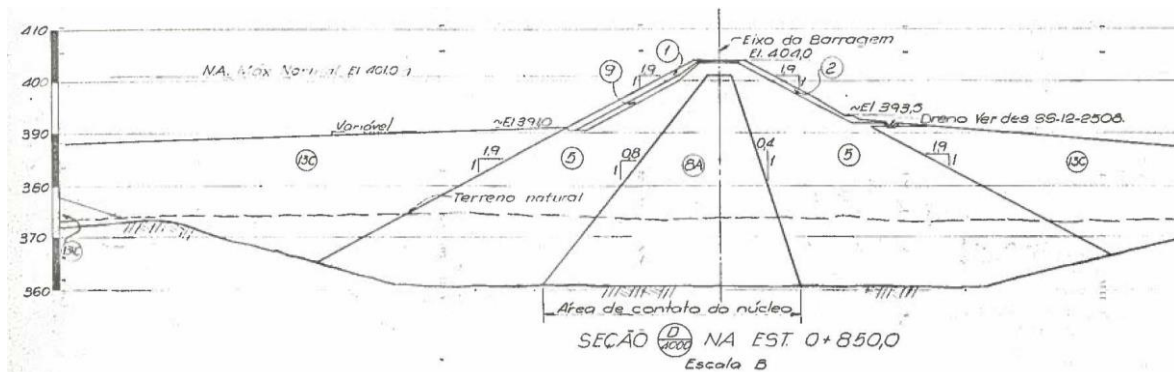
Figura 3.10: Seção de estudo da margem direita (CEMIG, 1973b)
