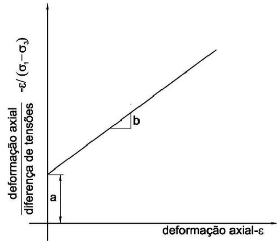
Figura 2.4: Curva tensão deformação hiperbólica transformada
