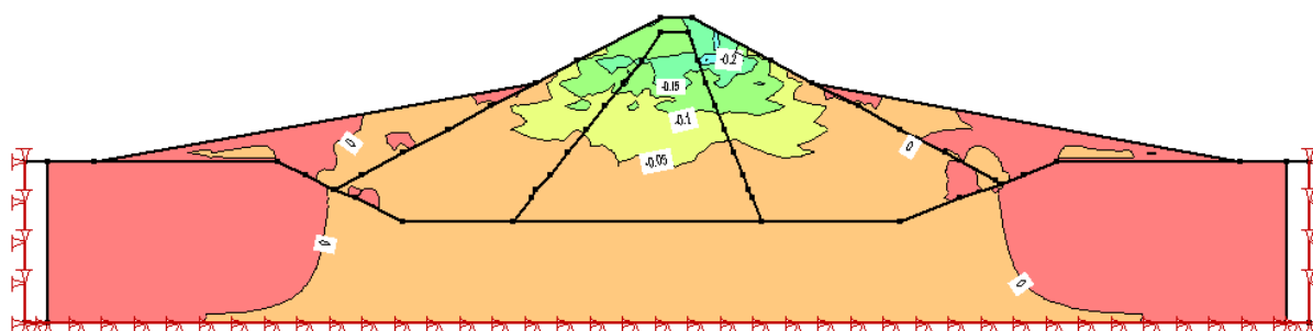
Figura 4.7: Deslocamentos verticais – margem direita (valores em m)
