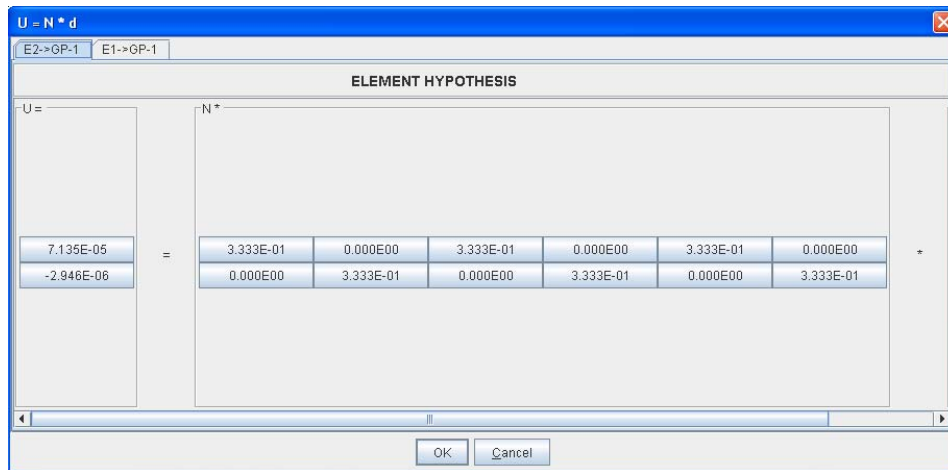
Figura 5.7: Deslocamentos nos pontos de Gauss selecionados.
