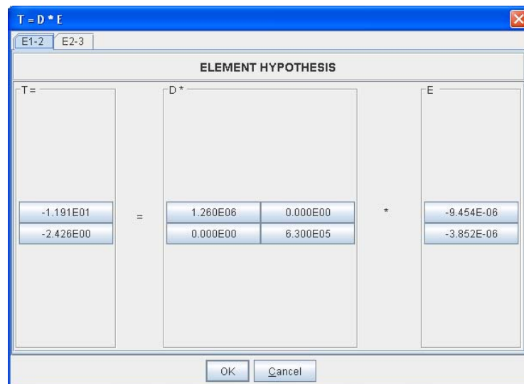
Figura 6.51: Esforços em um ponto qualquer do elemento.
