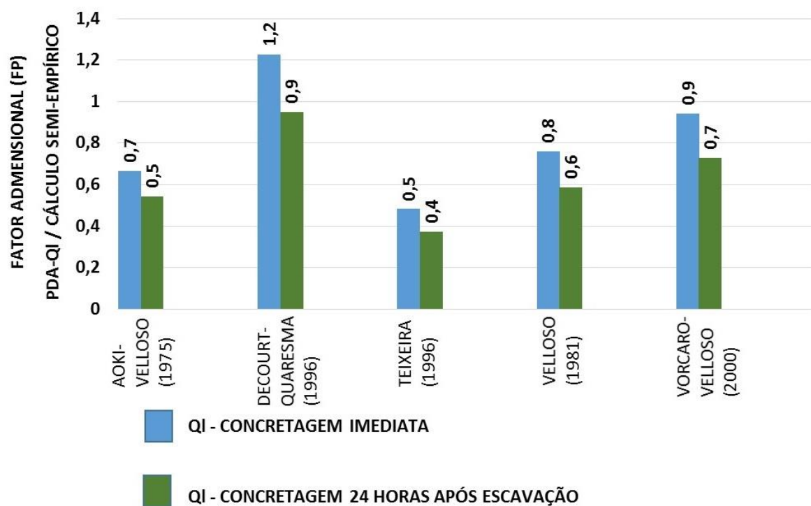
Figura 5.6: Razão entre os resultados dos ensaios de campo e os resultados dos cálculos obtidos de diferentes métodos semi-empíricos para carga lateral- campo de teste nº02
