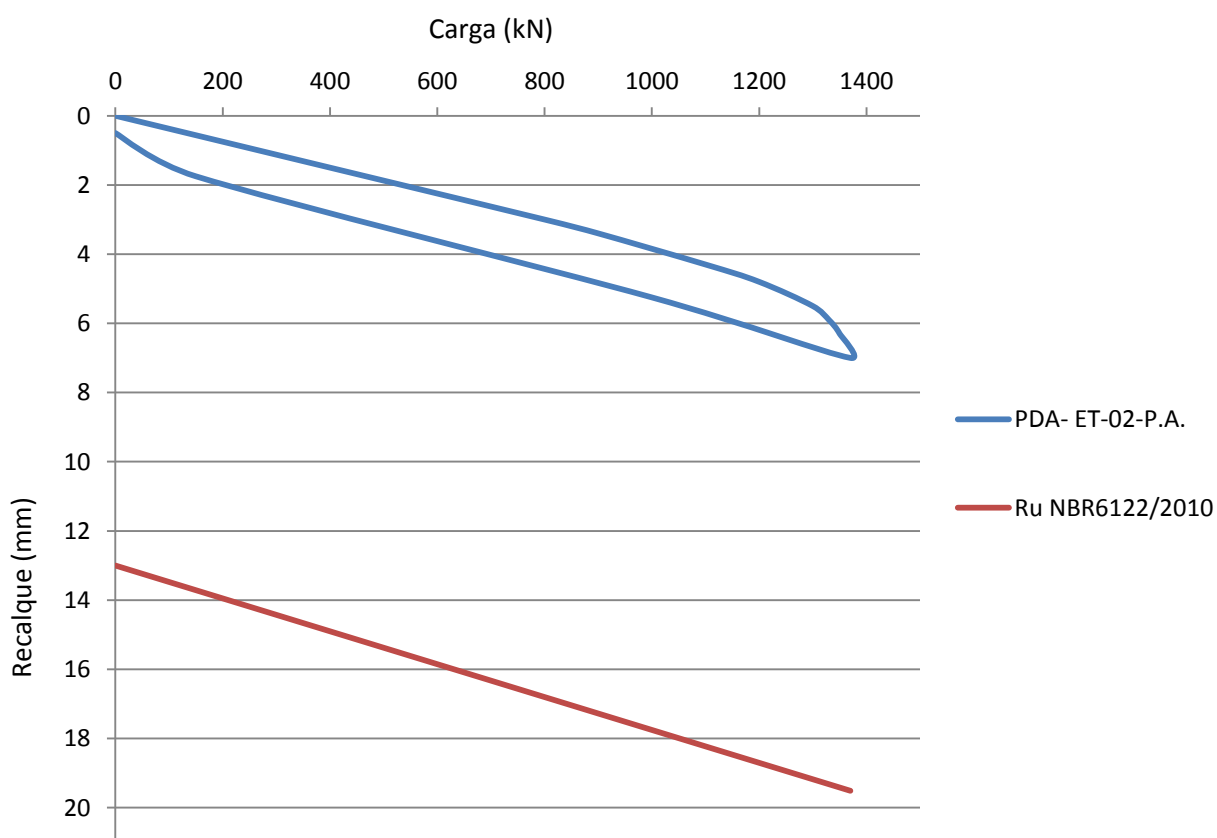
Gráfico carga x recalque – Estaca – ET-02-P.A.
