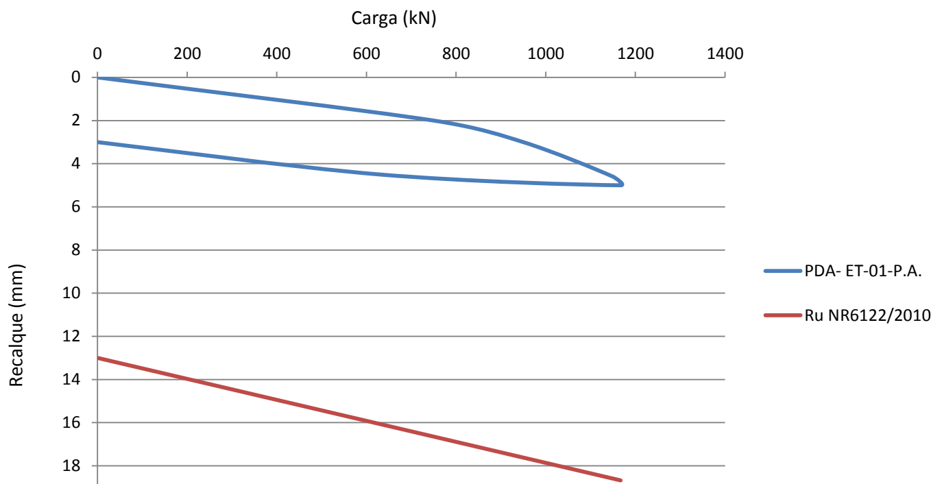
Gráfico carga x recalque – Estaca – ET-01-P.A.
