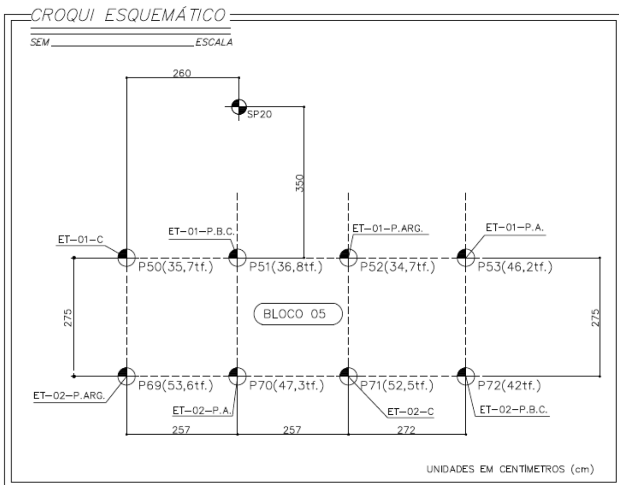
Figura 3.17: Disposição das estacas ensaiadas – campo de teste nº01
