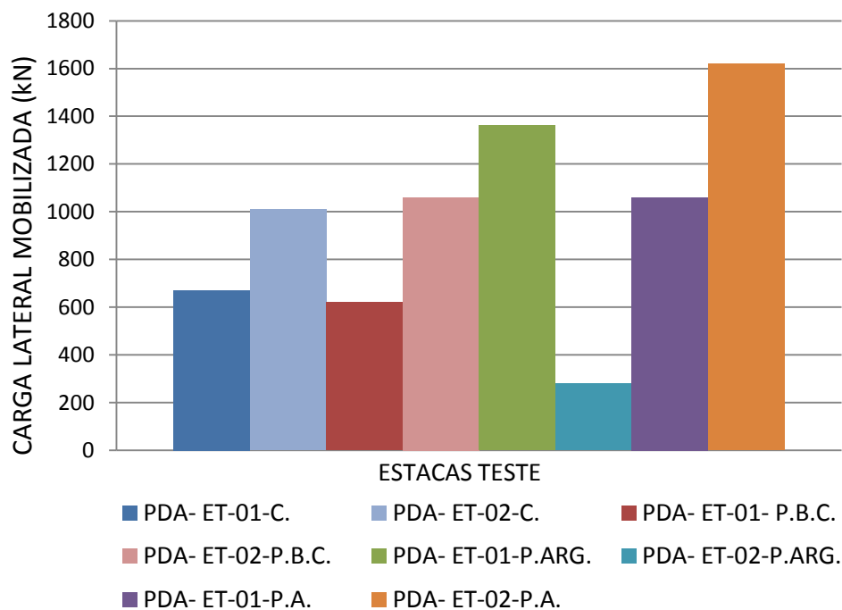
Figura 4.1: Gráfico para cargas laterais mobilizadas no campo de teste nº 01.
