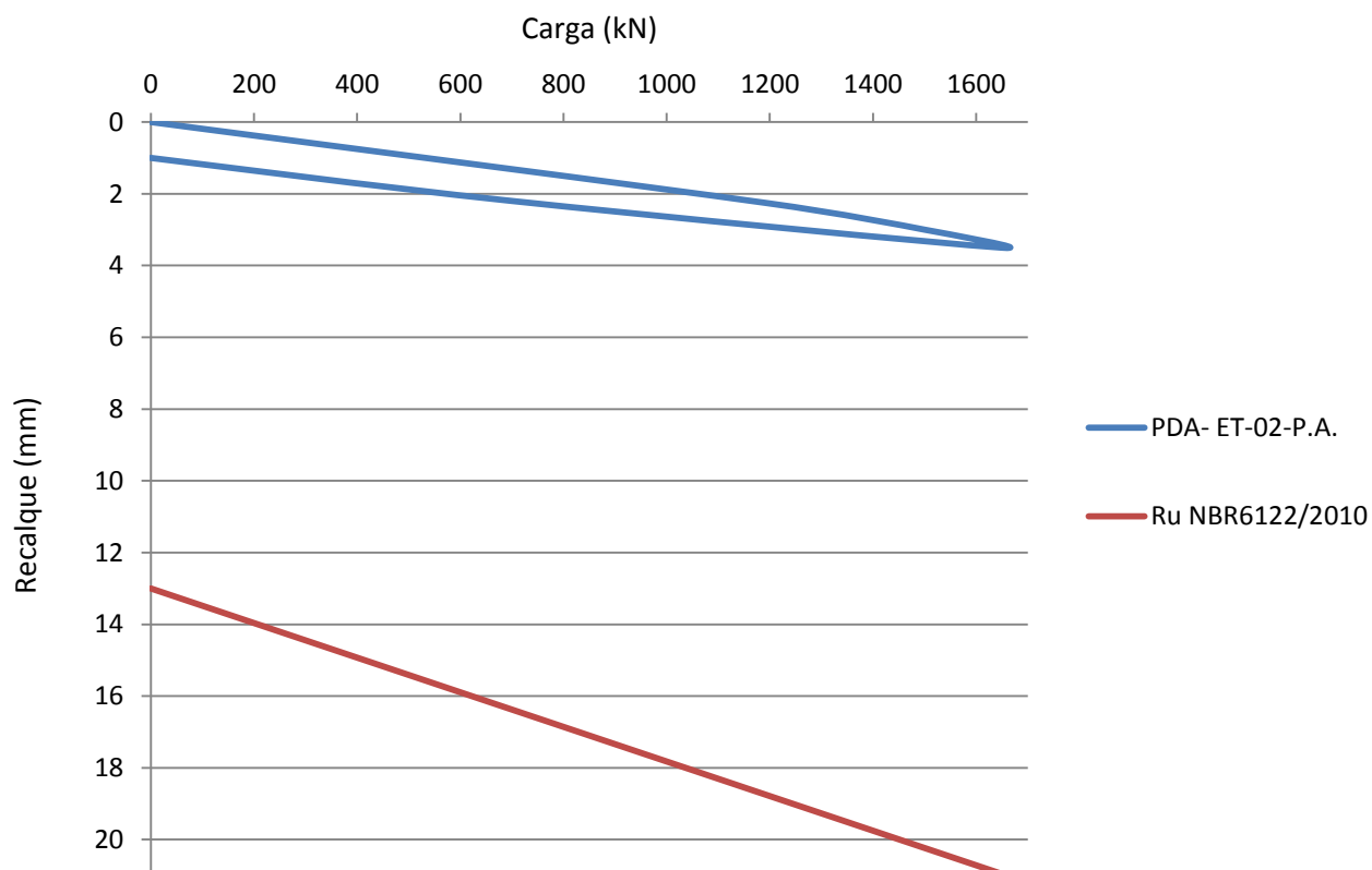
Gráfico carga x recalque – Estaca – ET-02-P.A.
