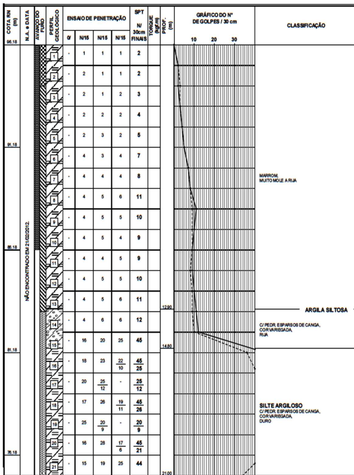
Figura 3.22: Perfil geotécnico – SP-11 de referência do campo de teste nº03
