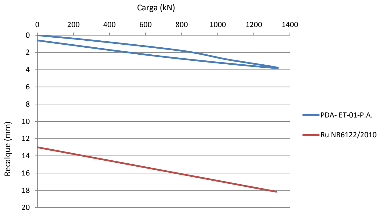
Gráfico carga x recalque – Estaca – ET-01-P.A.
