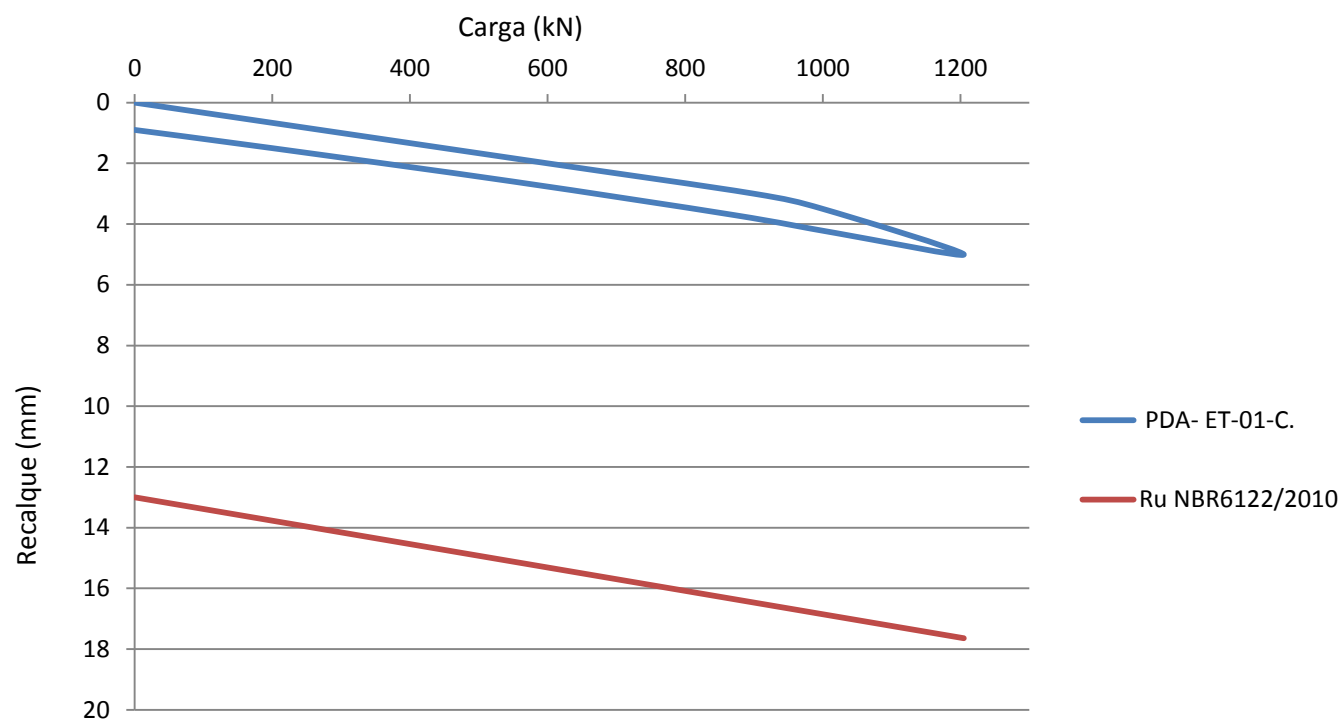
Gráfico carga x recalque – Estaca – ET-01-C.
