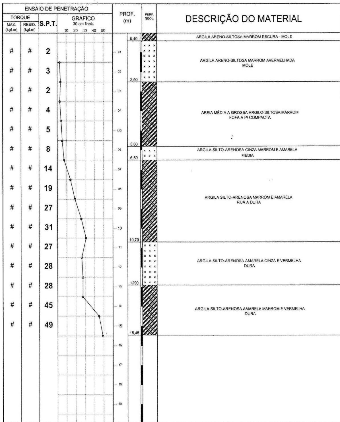
Figura 3.25: Perfil geotécnico – SP-06 de referência do campo de teste nº04
