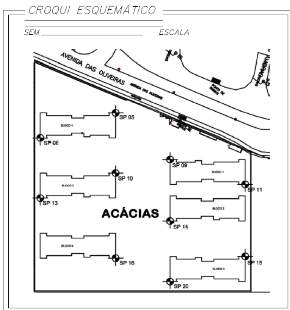
Figura 3.24: Croqui esquemático de localização do empreendimento – campo de teste nº04
