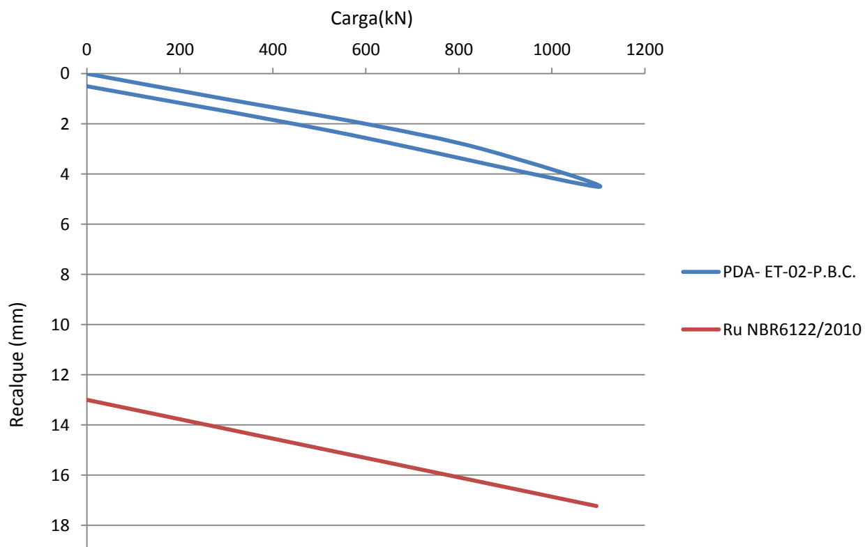
Gráfico carga x recalque – Estaca – ET-02-P.B.C.
