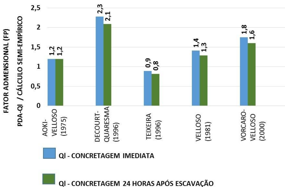
Figura 5.7: Razão entre os resultados dos ensaios de campo e os resultados dos cálculos obtidos de diferentes métodos semi-empíricos para carga lateral- campo de teste nº03
