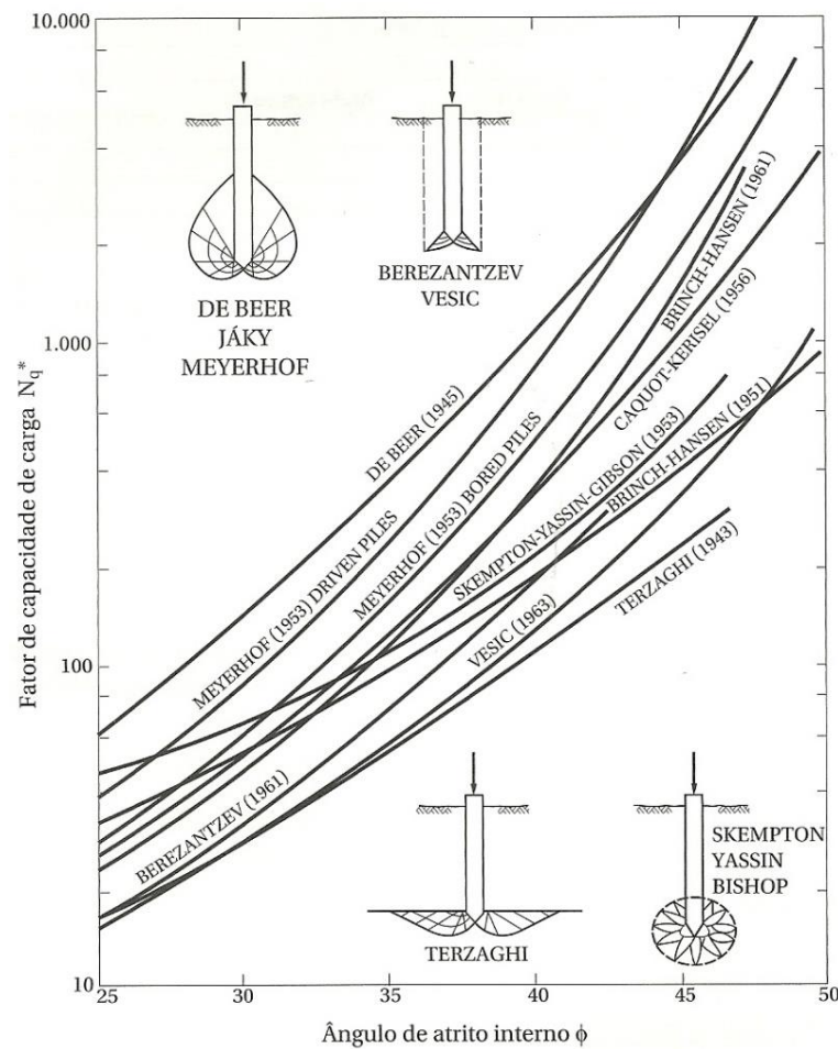
Figura 2.10: Valores de N_q^* (Vesic, 1967 apud CINTRA E AOKI, 2010)
