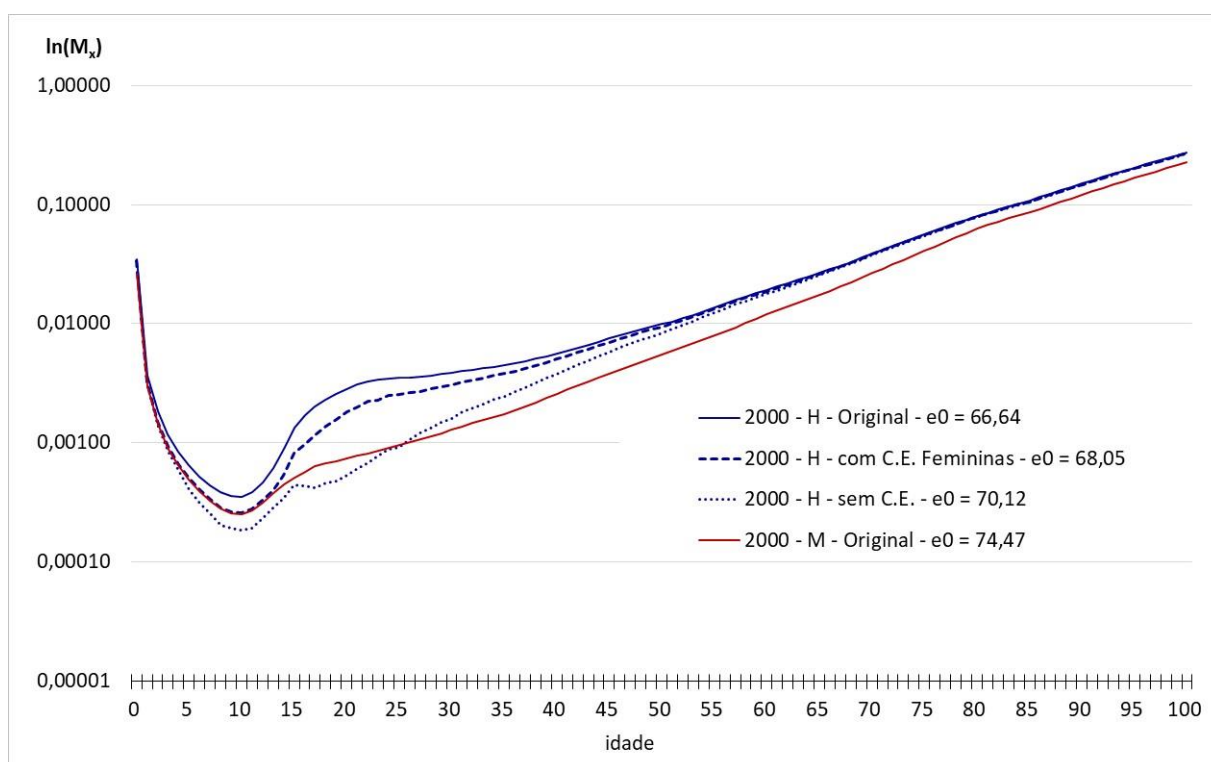
Gráfico 31 – Brasil – M_x 's Masculinas com e sem decremento de Causas Externas – 2000
