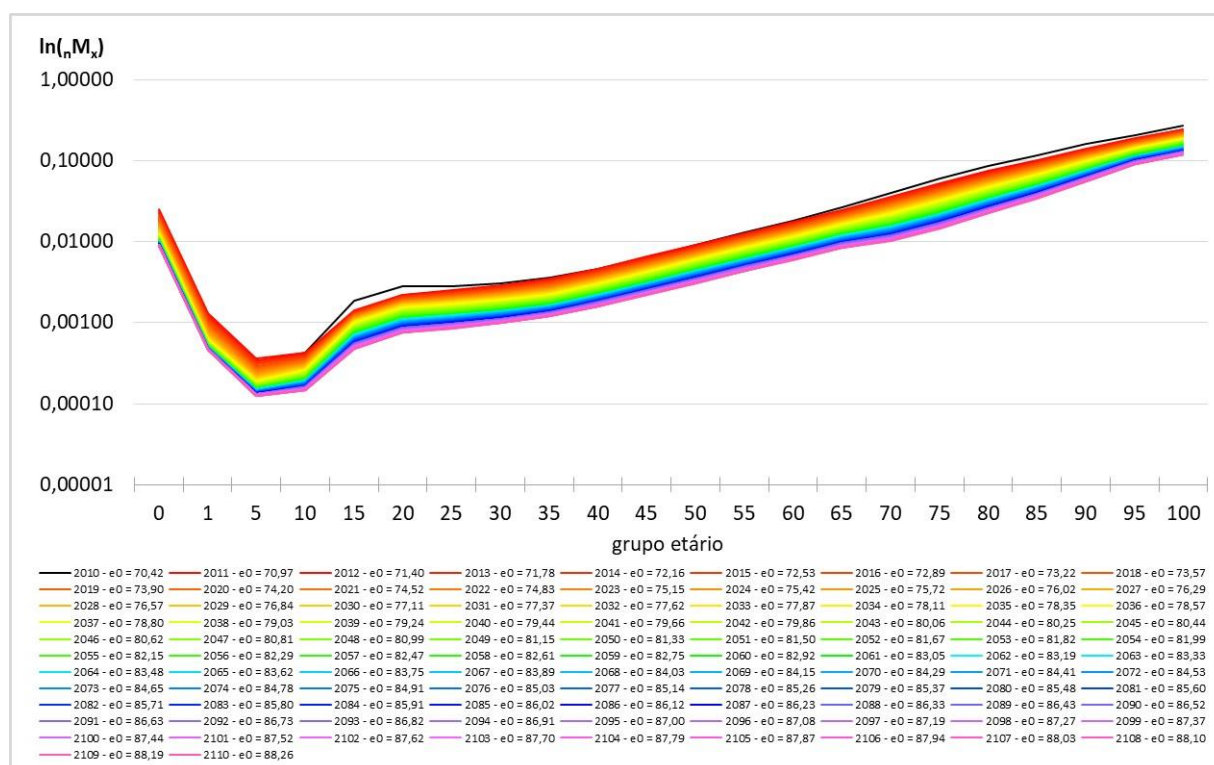
Gráfico 33 – Brasil – {}_nM_x 's Proj. método coerente de Li, Lee, & Gerland (2013) – Homem
