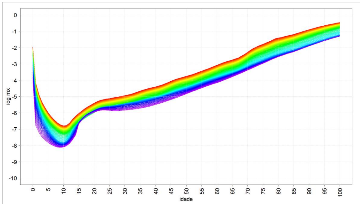
Gráfico 7 – Brasil – M_x 's interpoladas (2D) – Homem – 1950-2010
