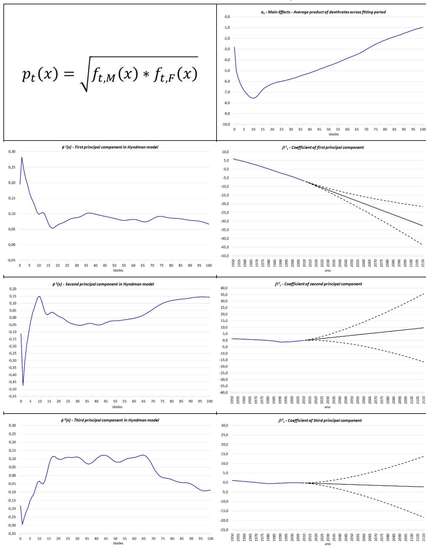
Painel 6 – Brasil – Resultados método COE – Função Produto
