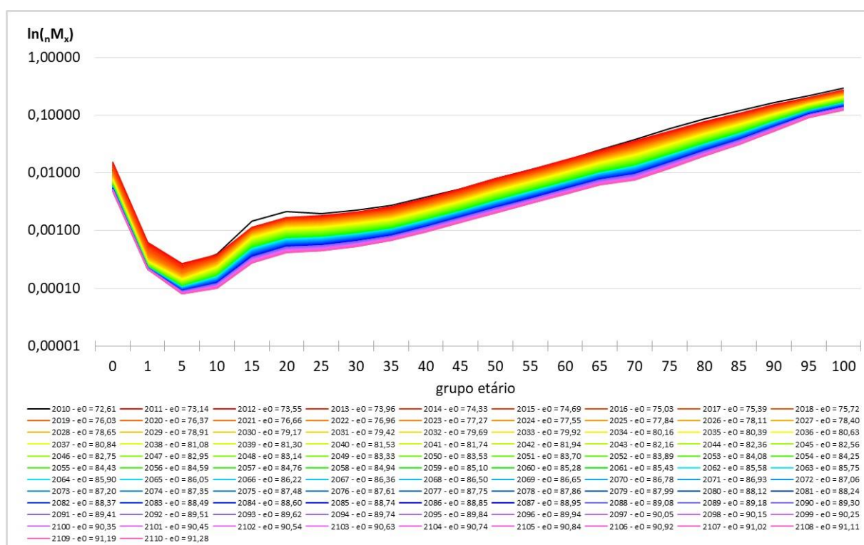
Gráfico 54 – Região Sul – {}_nM_x 's Proj. método de Li, Lee, & Gerland (2013) – Homem
