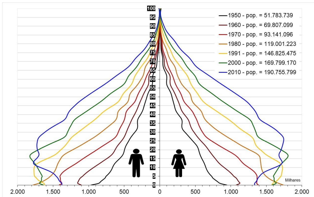
Gráfico 1 – Brasil – Pirâmides Populacionais Ajustadas Sobrepostas – 1950-2010 (números absolutos – em milhares de pessoas)
