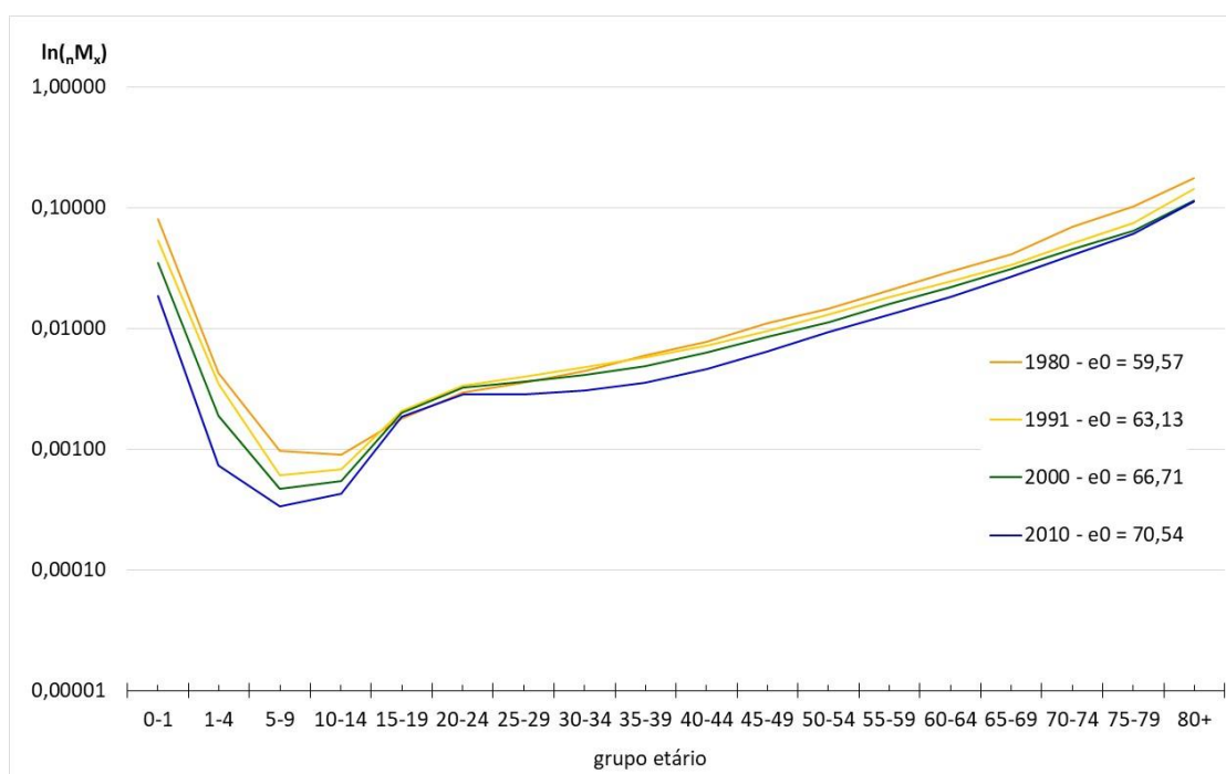
Gráfico 2 – Brasil – Taxas Centrais de Mortalidade ( {}_nM_x 's – escala ln) – Homem
