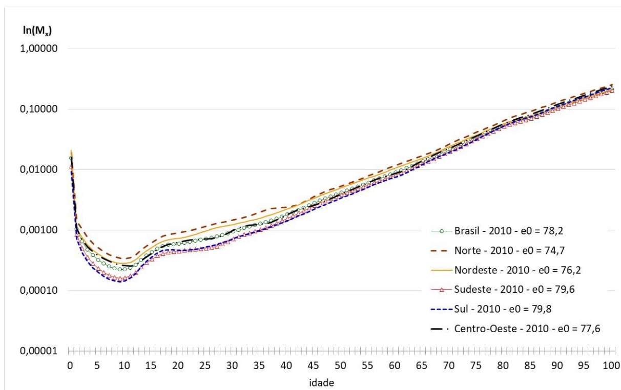
Gráfico 39 – Taxas Centrais de Mortalidade ( M_x 's) – Brasil e Grandes Regiões – 2010 – Mulher
