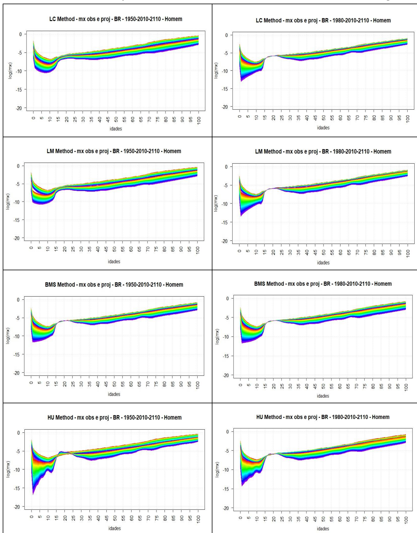
Painel 3 – Brasil – M_x 's Proj. Homem – Períodos: 1950-2010 e 1980-2010 – Diversas Metodologias
