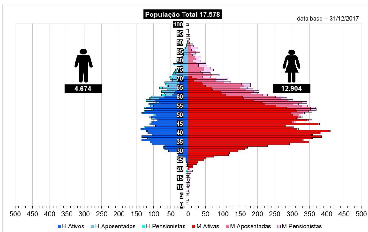
Gráfico 91 – Pirâmide Populacional da base de dados fictícia utilizada na Simulação Atuarial
