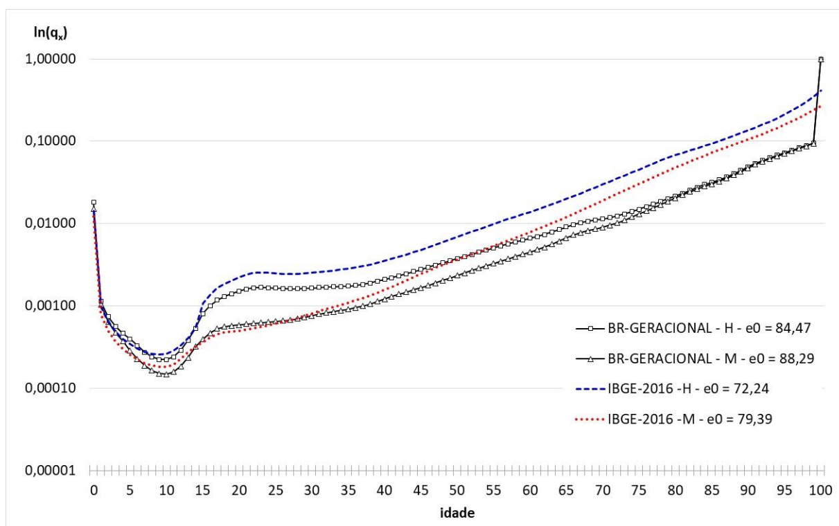
Gráfico 67 – q_x 's – Tábua BR-Geracional X Tábua IBGE-2016
