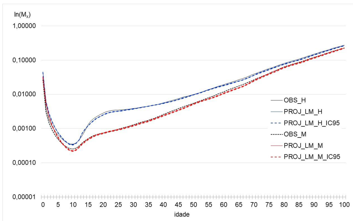
Gráfico 17 – Brasil – M_x 's Proj. X Obs. – Ano 2000 – método LM – Período 1950-1990 – H e M
