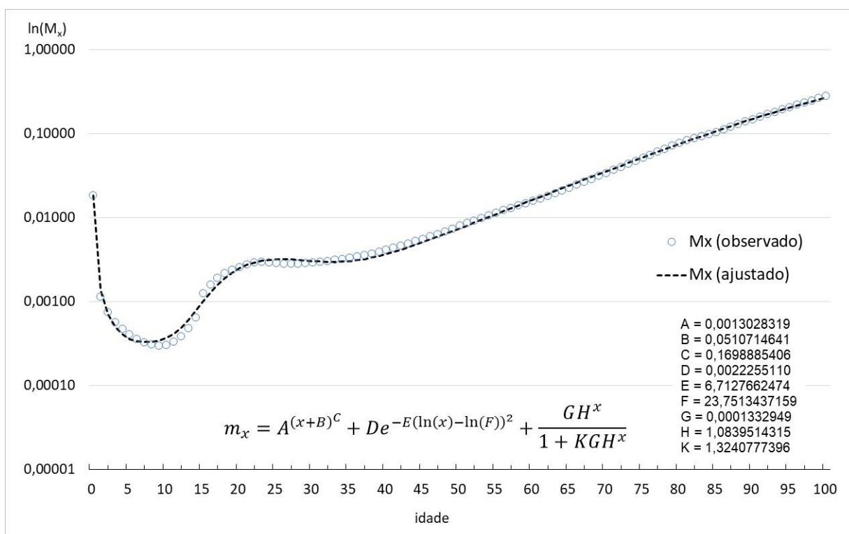
Gráfico 14 – Brasil – M_x 's – Valores Observados X Ajustados HP3 – 2010 – Homem
