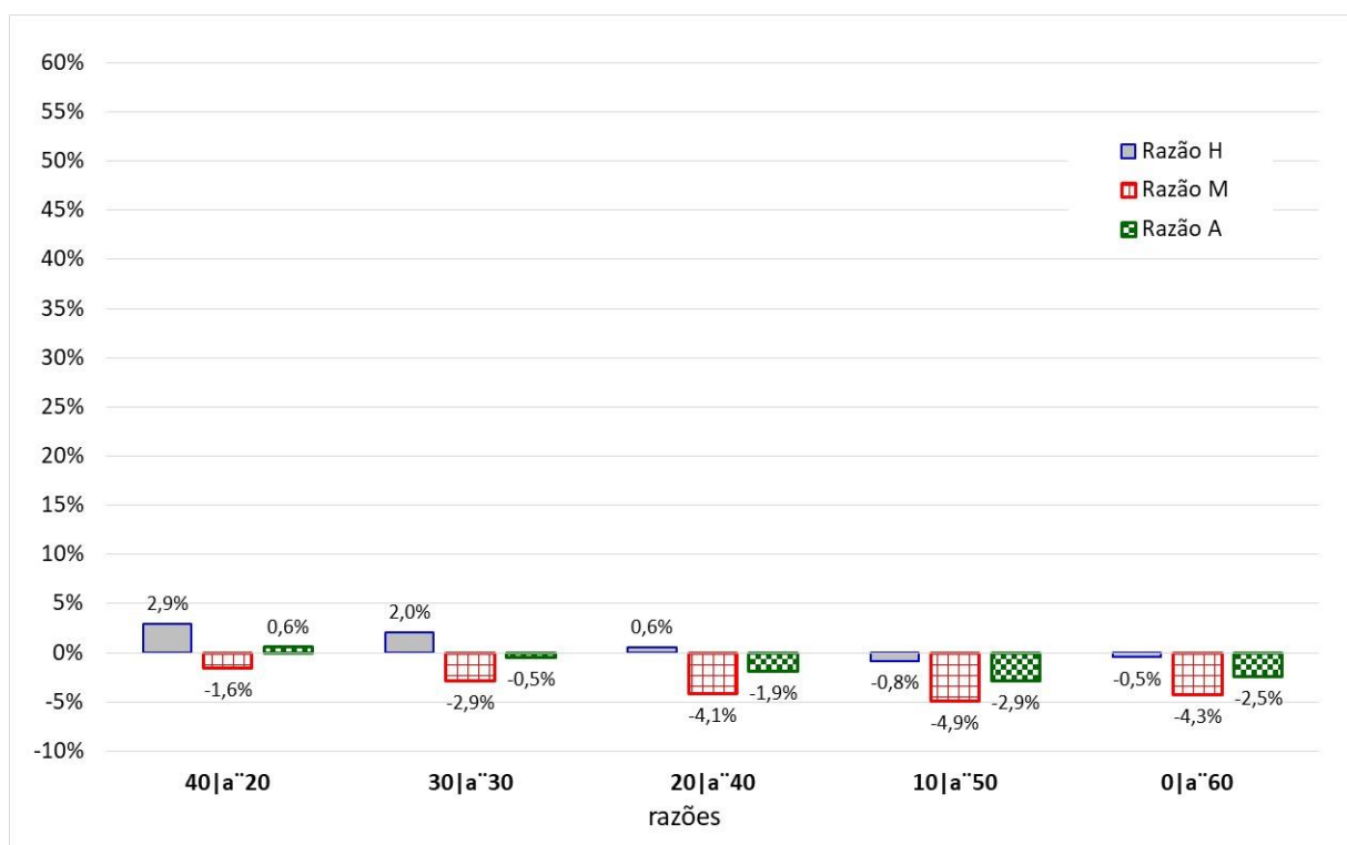
Gráfico 85 – IRL_x – benchmark Tábua EMS-sb-2015, taxa de juros de 6% a.a., BC 60 anos
