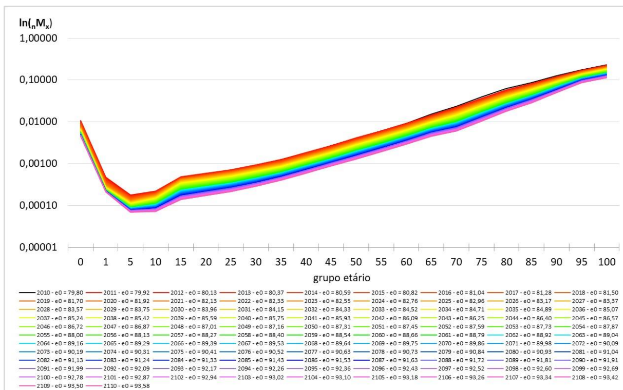
Gráfico 55 – Região Sul – nM_x 's Proj. método de Li, Lee, & Gerland (2013) – Mulher
