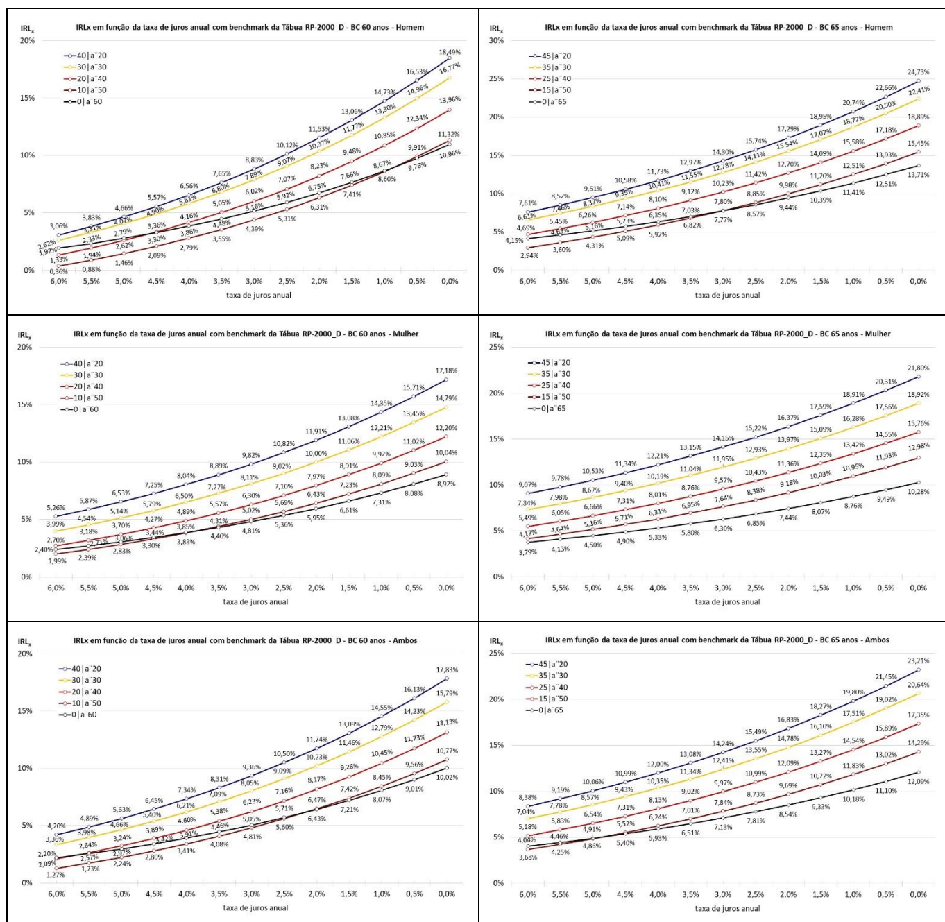
Painel 22 – Impacto do Risco de Longevidade em função da taxa de juros com benchmark na Tábua RP-2000 proj. escala AA p/ 2019 – Homem, Mulher e Ambos os Sexos
