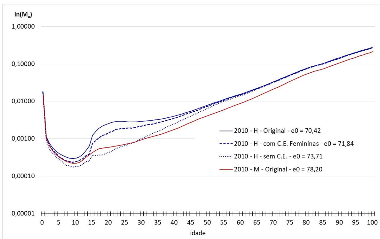
Gráfico 32 – Brasil – M_x 's Masculinas com e sem decremento de Causas Externas – 2010
