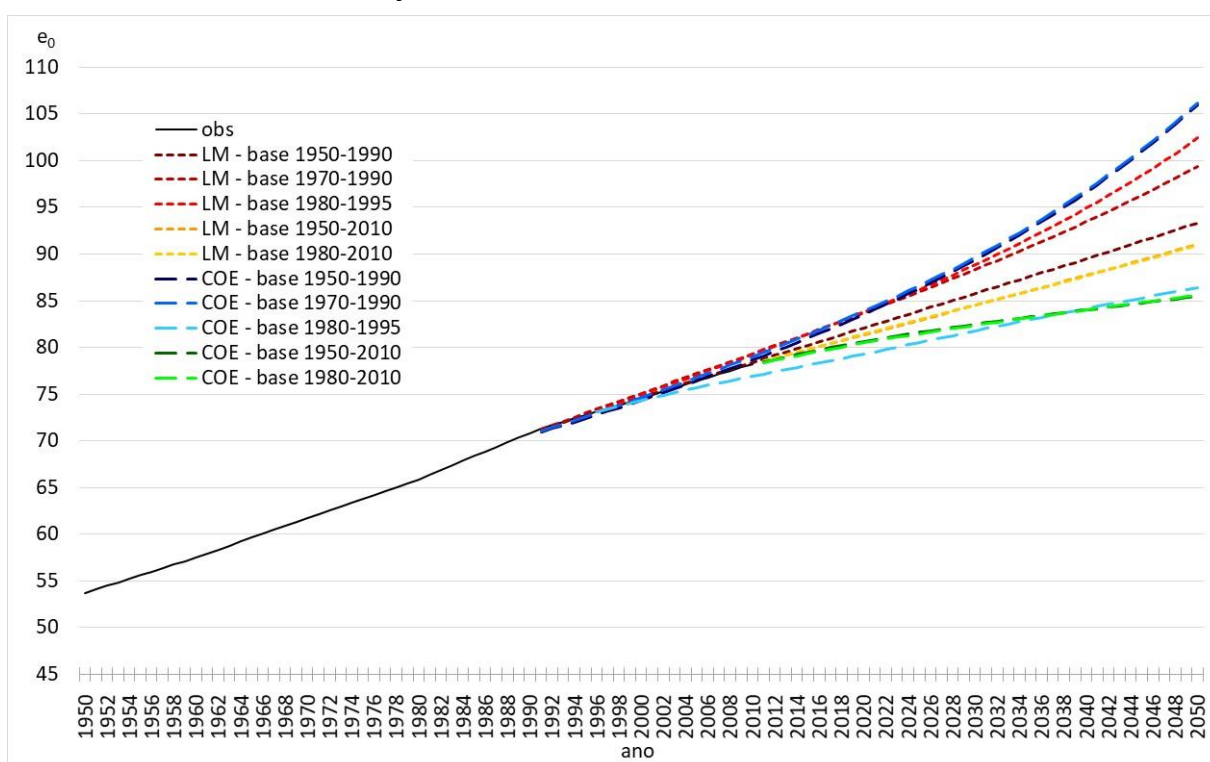
Gráfico 22 – Brasil – e_0 's Projetadas – métodos LM e COE – Vários Períodos Base – Mulher
