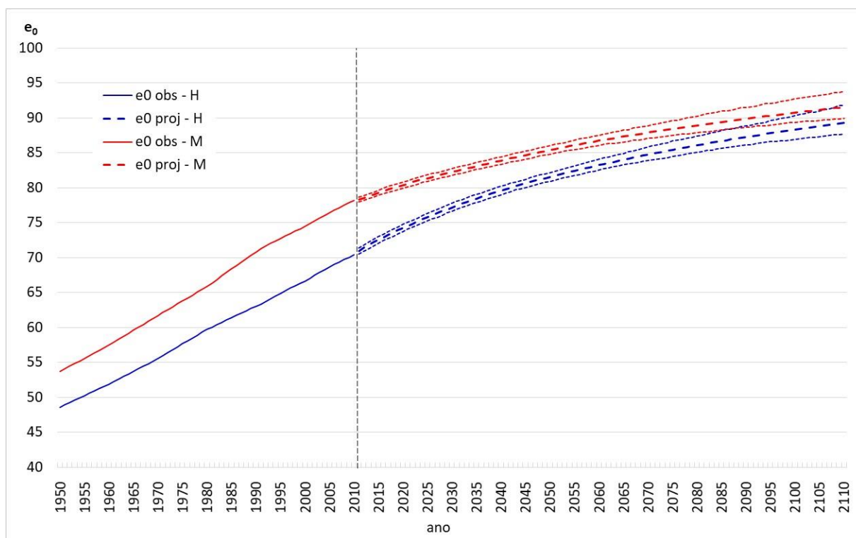
Gráfico 25 – Brasil – e_0 's Projetadas IC95 – método coerente Hyndman – Homem e Mulher
