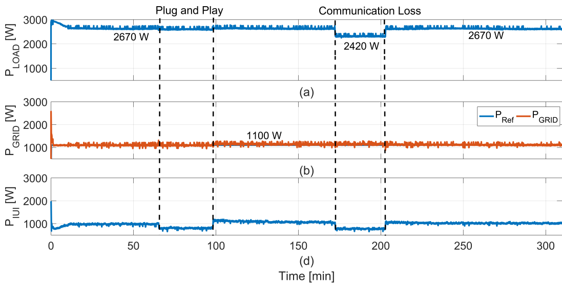
Figura 4.27: Medidas de Potência - Quinto Experimento.
