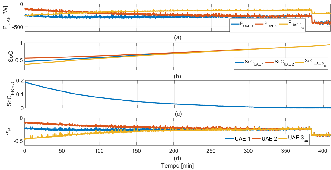
Figura 4.14: Grandezas das UAEs - Segundo Experimento.
