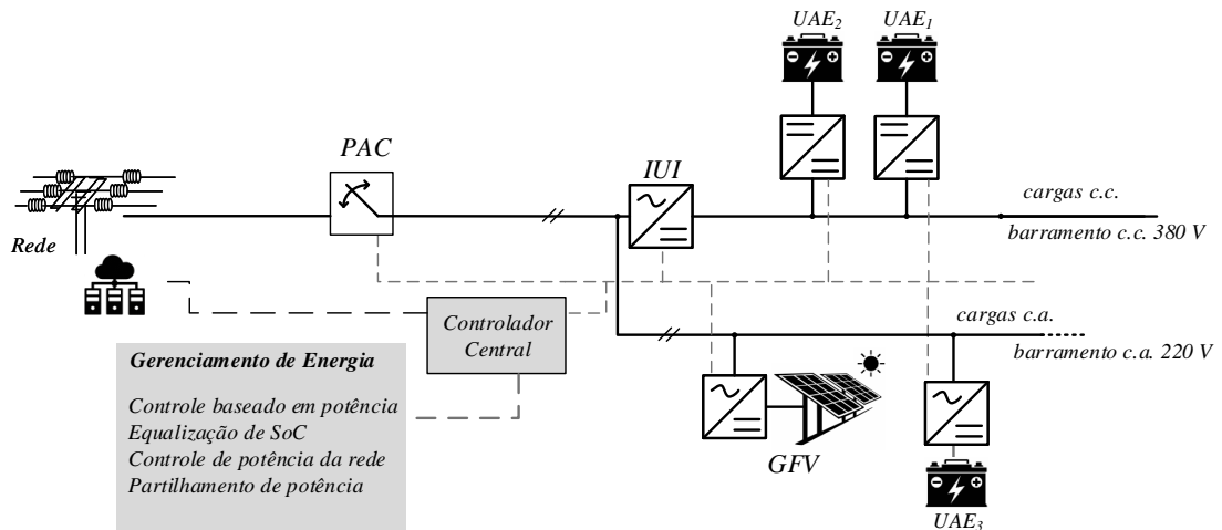
Figura 2.5: Estrutura Nanorrede Experimental.
