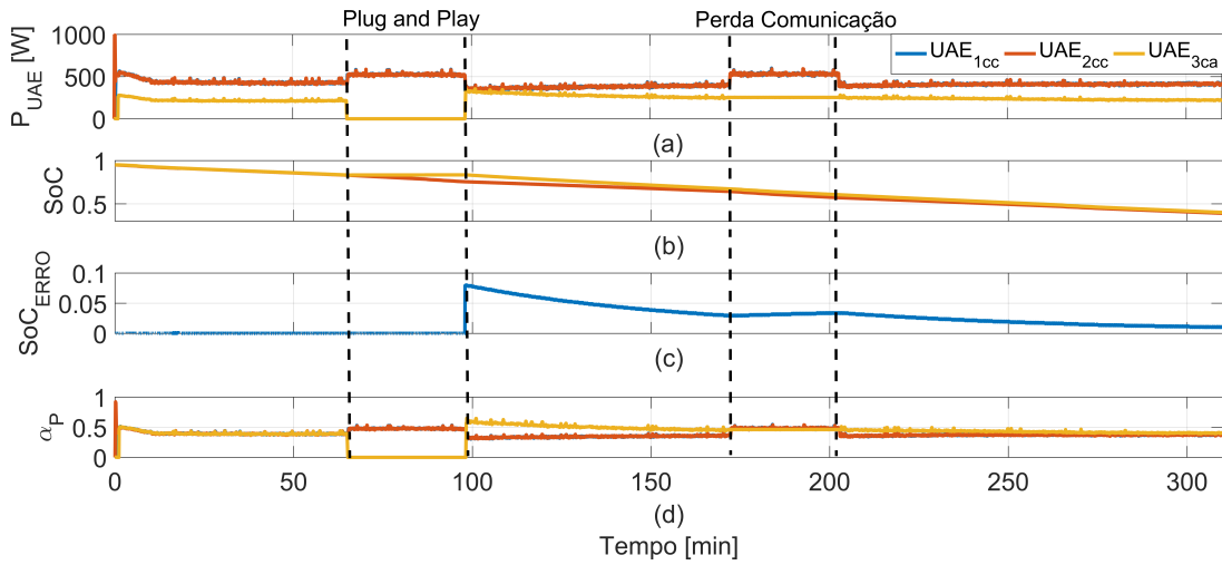
Figura 4.26: Grandezas das UAEs - Quinto Experimento.
