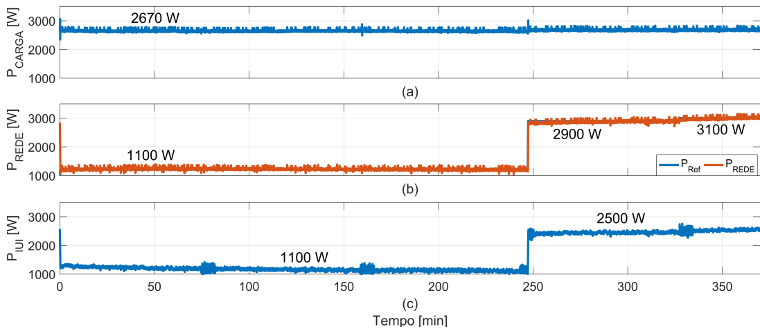
Figura 4.11: Medidas de Potência - Primeiro Experimento.
