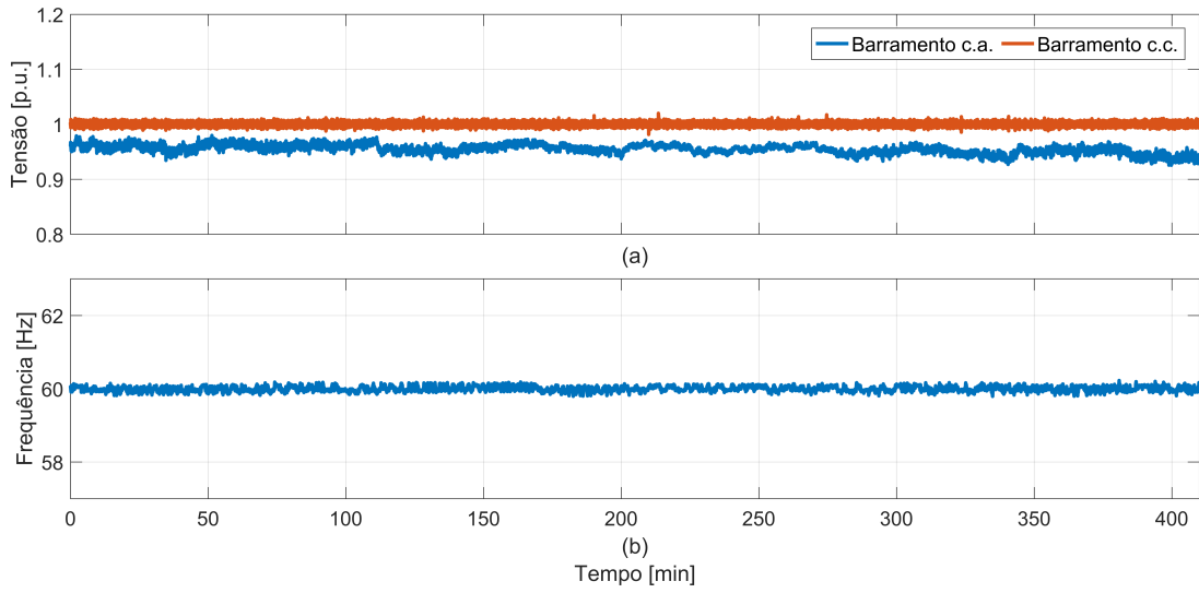
Figura 4.16: Medidas de Tensão e Frequência - Segundo Experimento.
