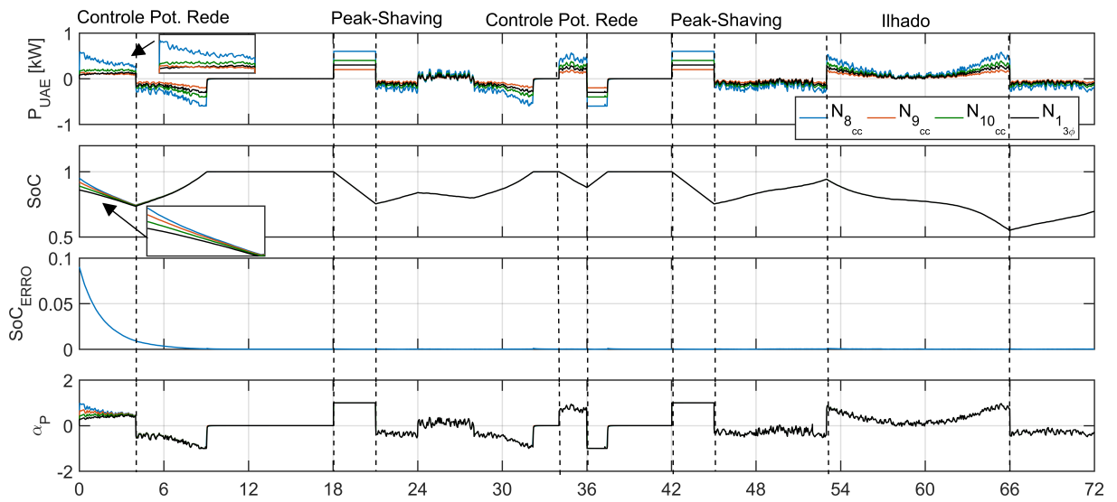
Figura 4.7: Medidas das Unidades de Armazenamento de Energia.
