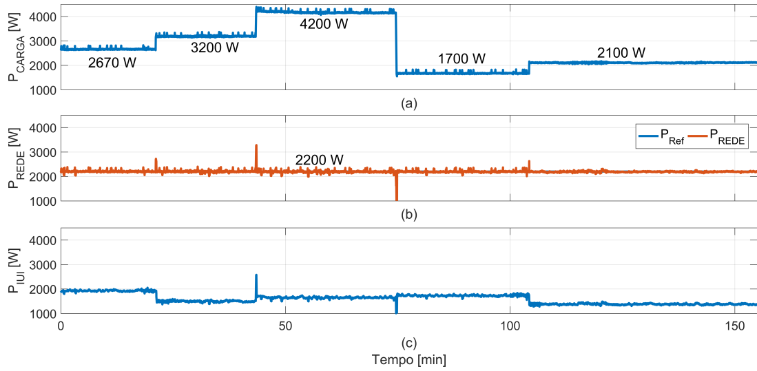
Figura 4.19: Medidas de Potência - Terceiro Experimento.
