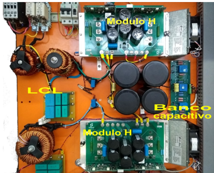
Figura 2.12: Montagem Experimental do Conversor IUI.
