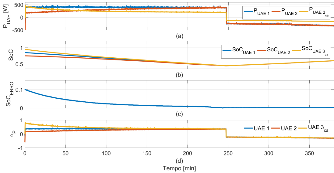
Figura 4.10: Grandezas das UAEs - Primeiro Experimento.
