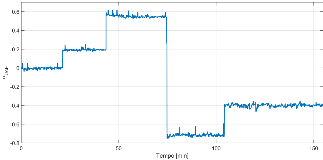
Figura 4.21: Coeficiente Escalar - Terceiro Experimento.
