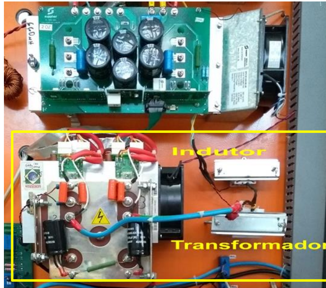
Figura 2.7: Conversor DAB Montado.
