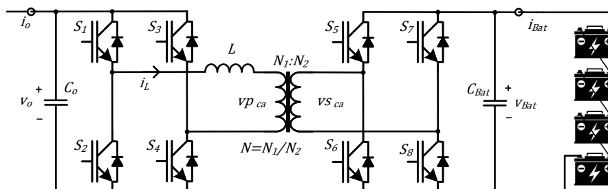
Figura 2.6: Conversor DAB.
