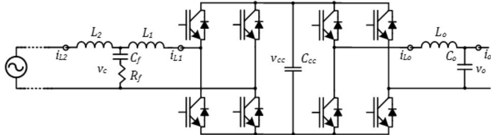
Figura 2.11: Topologia do Conversor IUI Monofásico.
