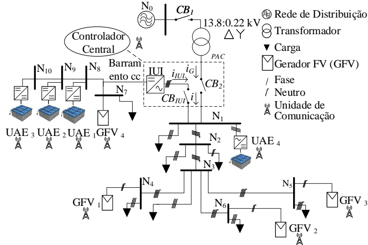
Figura 4.1: Estrutura da Microrrede Híbrida Utilizadas nas Simulações.
