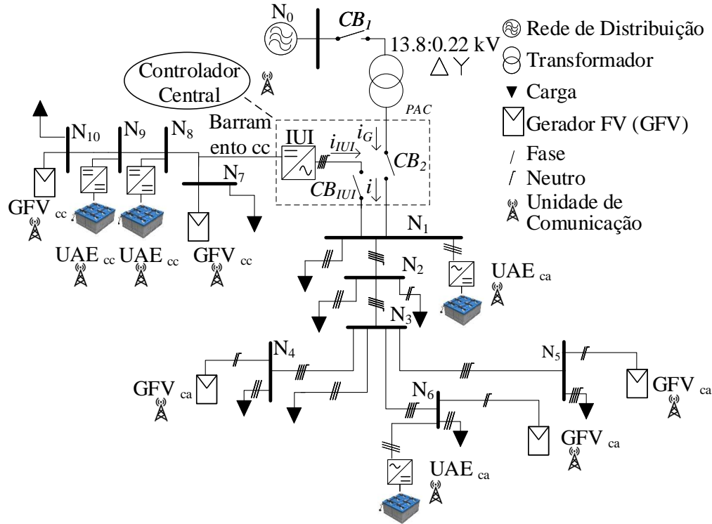
Figura 2.1: Estrutura da Microrrede Híbrida Proposta.
