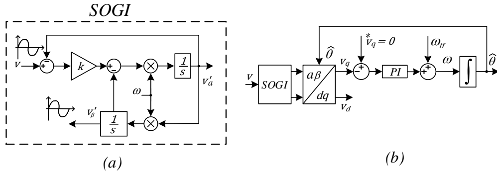
Figura 2.15: Estrutura do Algoritmo PLL.
