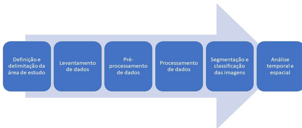
Figura 2 Fluxograma dos procedimentos metodológicos, Fonte Os autores
