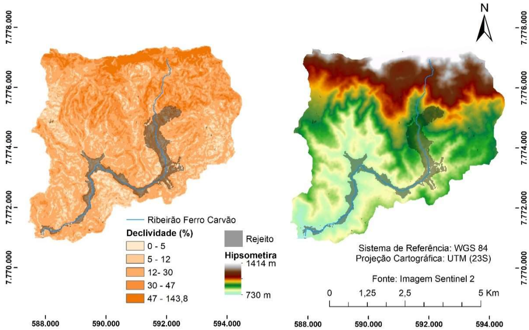
Mapa de declividade (%) e mapa hipsométrico (m) da Sub bacia em Brumadinho
