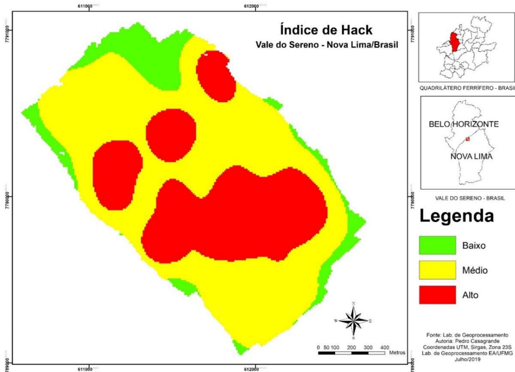
Figura 3: Índice de Hack da área
