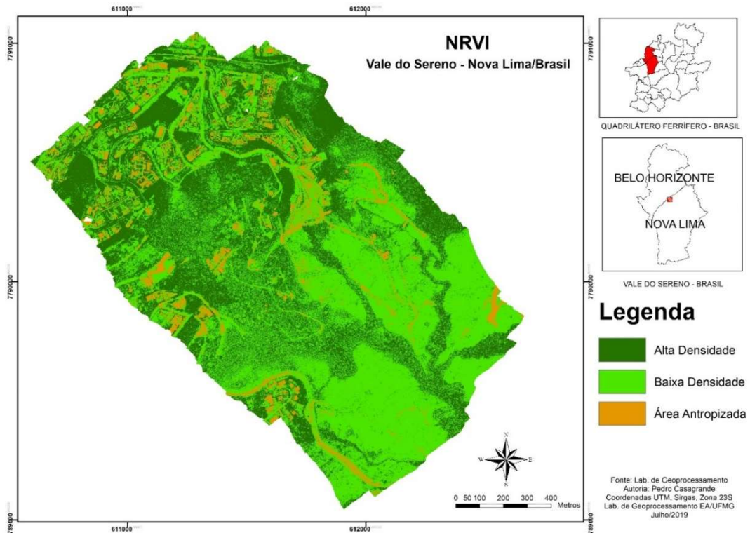
Figura 4: NRVI da área
