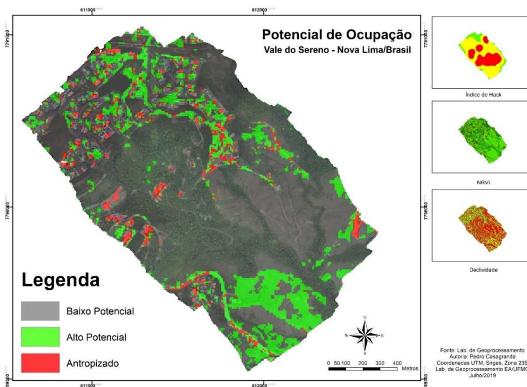
Figura 6: Potencial de ocupação
