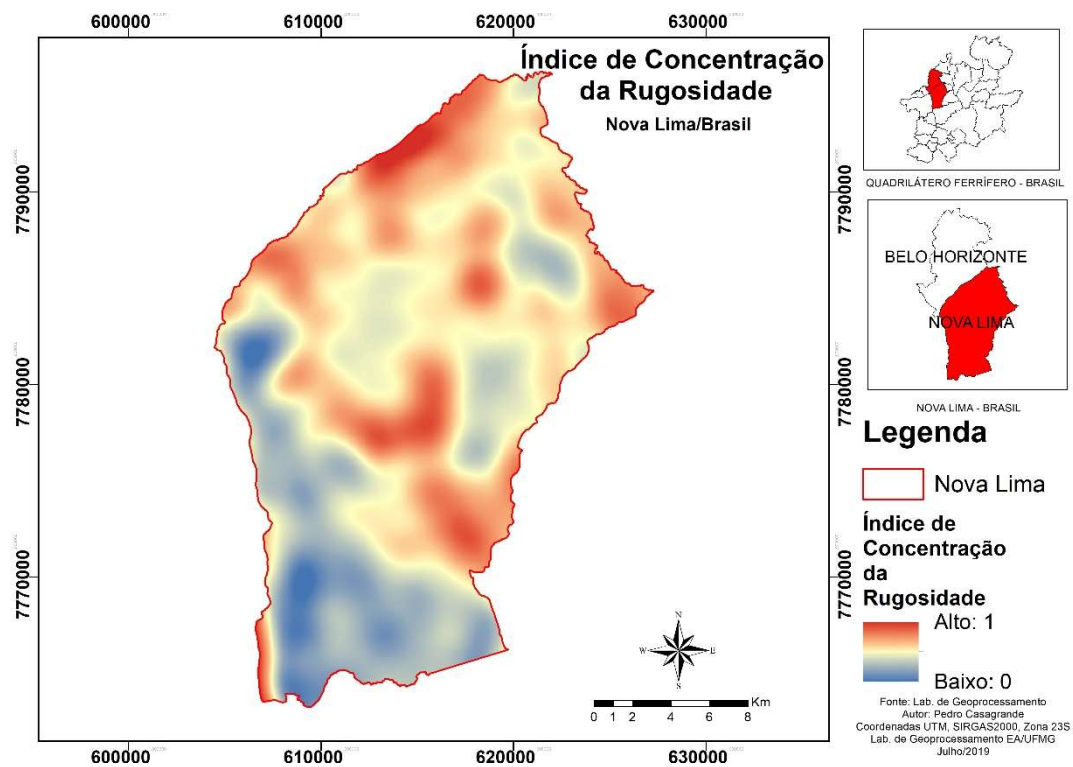
Figura 5: Mapa do Índice de Concentração da Rugosidade.
