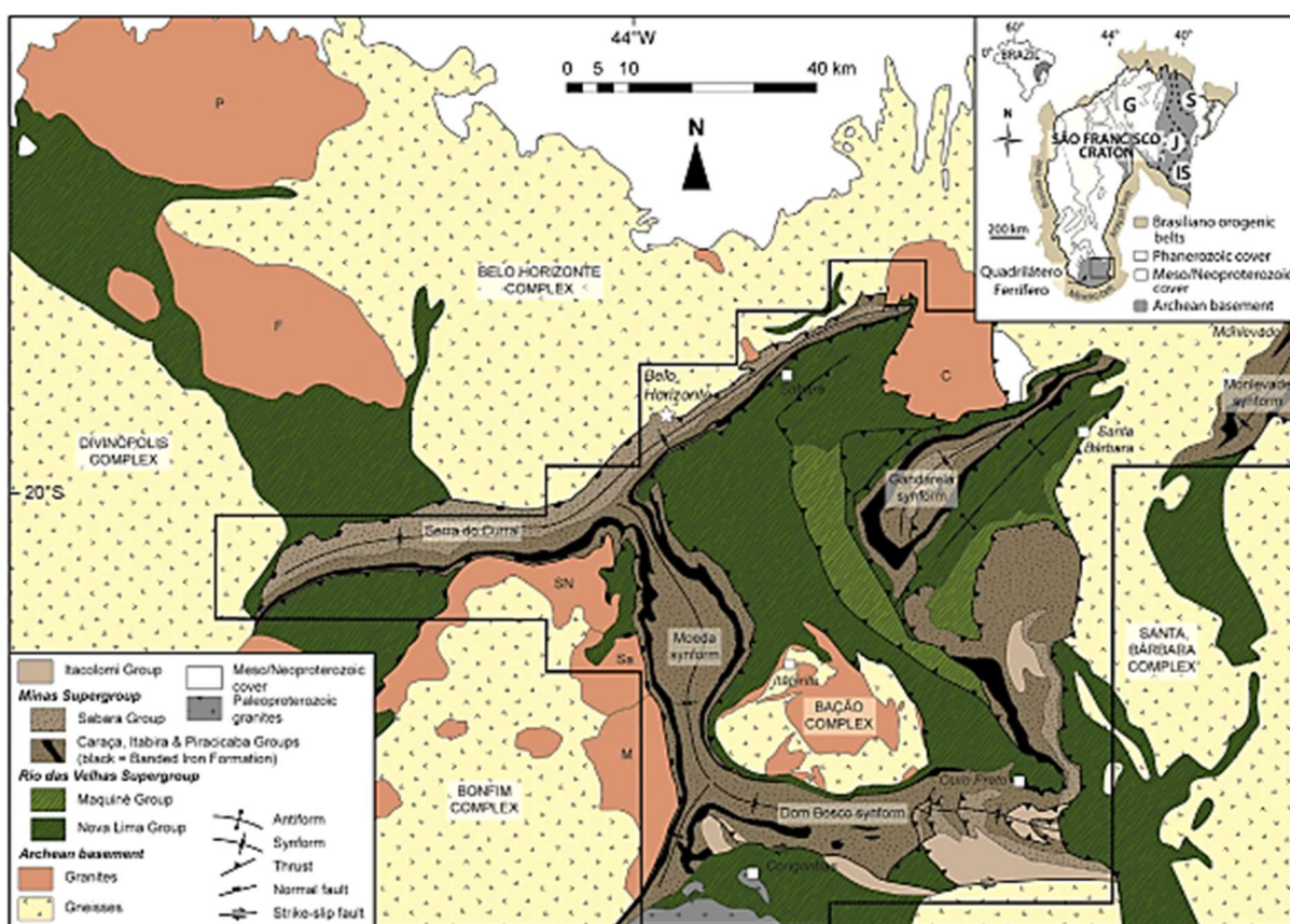
Figura 4: Mapa Geológico do Quadrilátero Ferrífero. Fonte: Farina et al , 2015.
