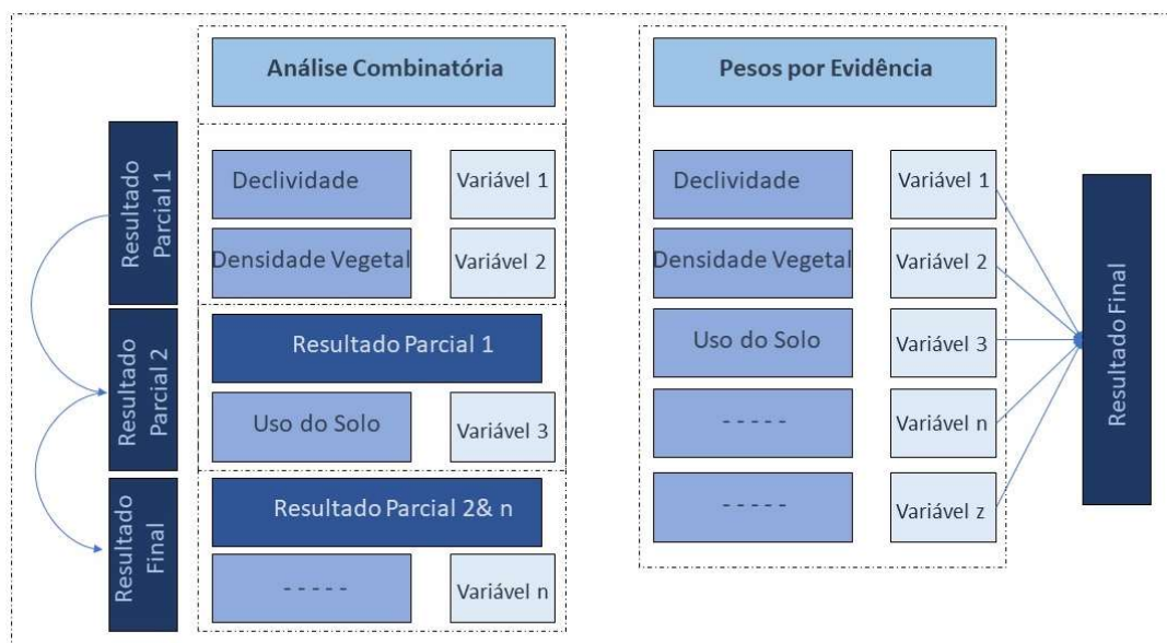
Figura 1: Esquema metodológico, exemplo que compara os dois métodos multicritérios. Na Análise Combinatória o processo ocorre por etapas de análise par a par, gerando resultados parciais, sucessivamente caso seja acrescentado mais variáveis ( n variáveis) até a última análise que será o resultado final. Na etapa de Pesos e Evidência, a análise ocorre com todas as variáveis ao mesmo tempo, onde cada uma recebe um peso gerando um ranking classificatório como resultado final. Fonte: O autor, modificado de Rocha et al (2018).
