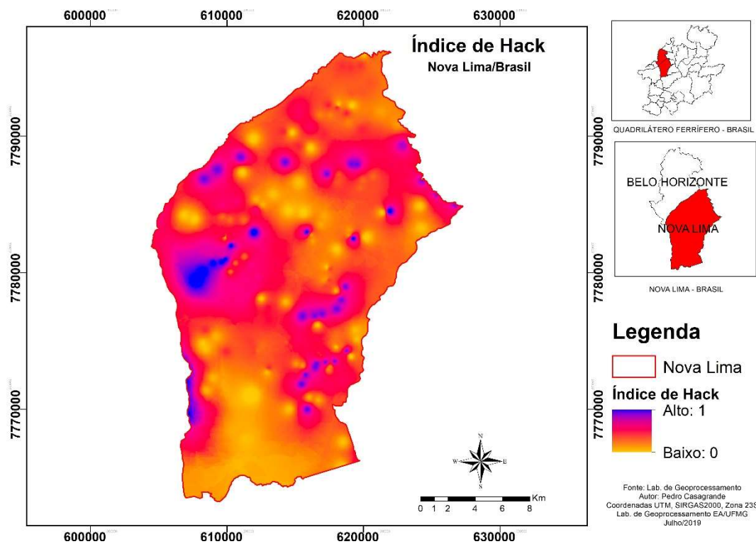
Figura 6: Mapa do índice de Hack
