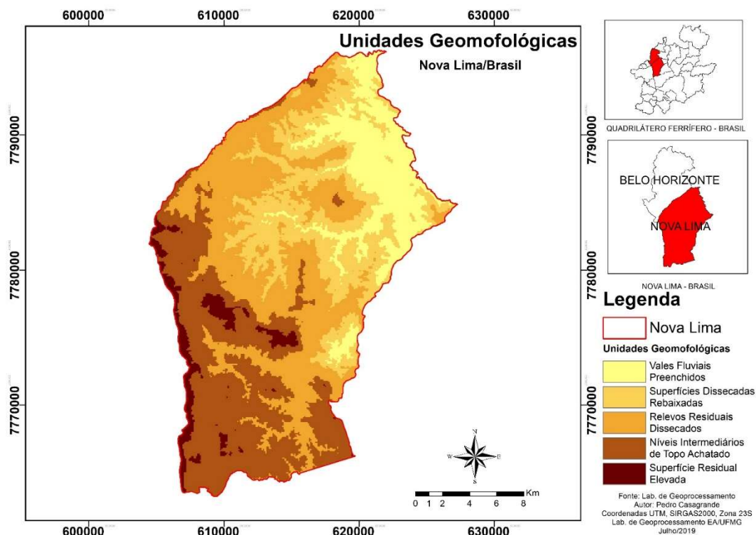
Figura 3: Mapa das unidades geomorfológicas do Município de Nova Lima
