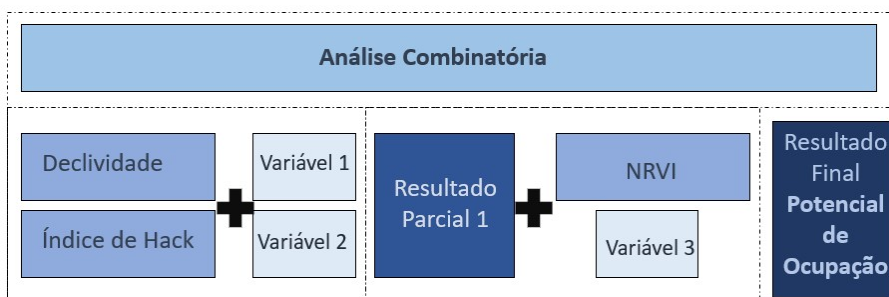
Figura 5: Lógica da Análise Combinatória
