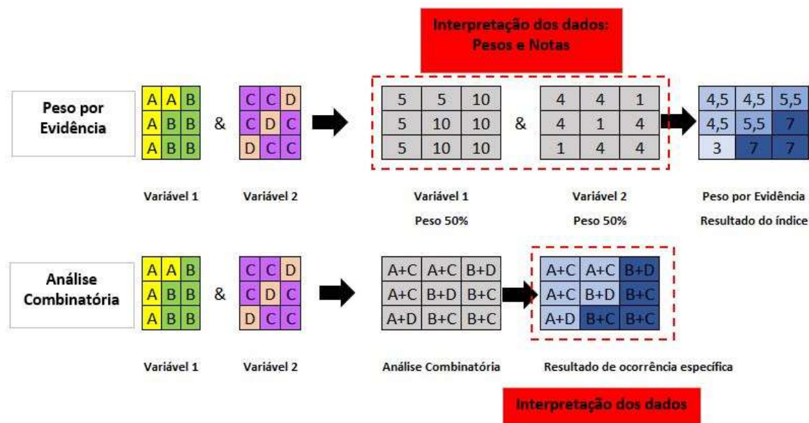
Figura 2: Na análise por Pesos de Evidência, é raciocinado a importância de cada variável em uma etapa anterior ao resultado final, que se apresenta como índice, no qual, por sua vez, não se consegue reconhecer o papel individual de cada variável, chegando-se a um resultado quantitativo e ordenado. Na Análise Combinatória, o raciocínio sobre o papel de cada variável acontece diante dos resultados parciais (ou final), segundo o significado da combinação obtida, logo, obtém-se um resultado qualitativo e seletivo. Fonte: O autor, modificado de Rocha et al (2018).
