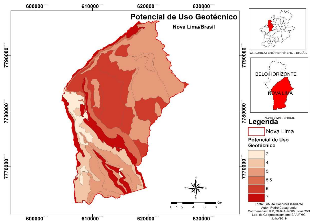
Figura 4: Mapa de Unidades Geotécnica (Parizzi, et al 2010).
