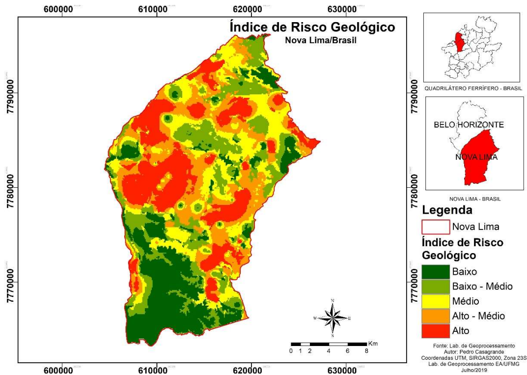
Figura 8: Mapa Índice de Risco Geológico.
