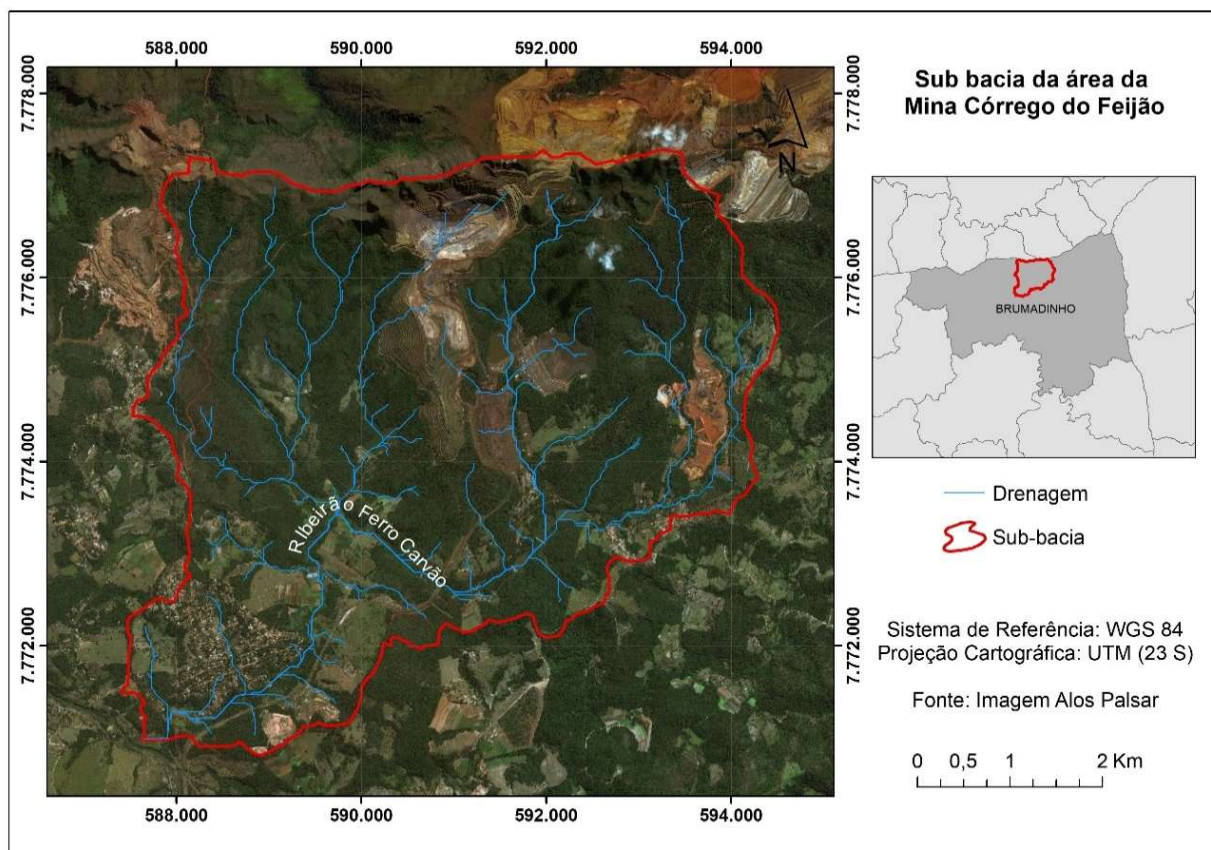
Figura 3 Mapa de localização da área de estudo. Bacia do Córrego de Feijão, Brumadinho/MG, Fonte Os autores
