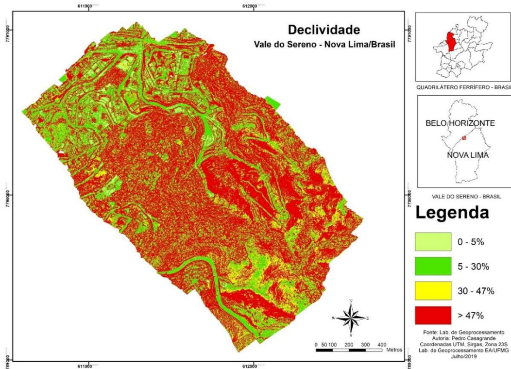
Figura 2: Declividade da área
