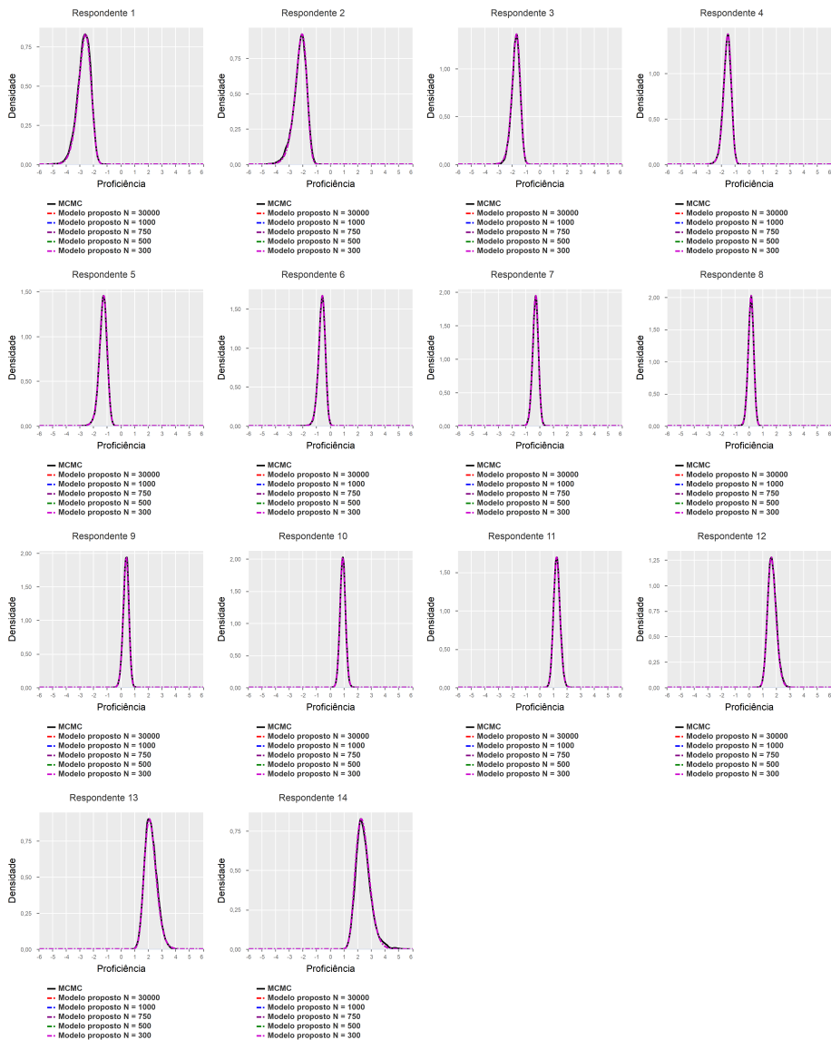
Figura 4 – Densidade da proficiência obtida via MCMC e a obtida pela metodologia proposta para diferentes tamanhos de cadeia dos parâmetros dos itens.
