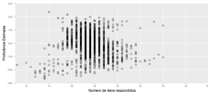
Figura 18 – Gráfico de dispersão - Proficiência estimada pelo teste adaptativo x Número de itens respondidos.
