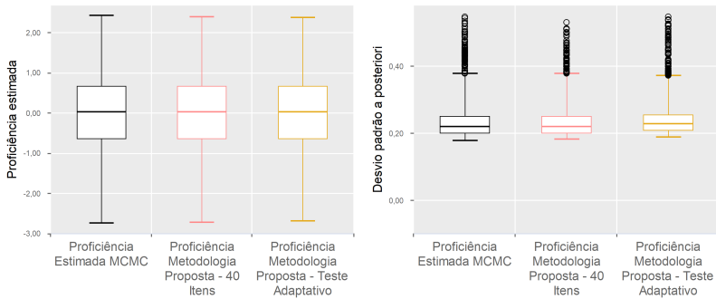
Figura 12 – Boxplot das proficiências e desvios padrão obtidos via MCMC, via metodologia proposta com 40 itens e através do teste adaptativo para os 2000 indivíduos do estudo de simulação.
