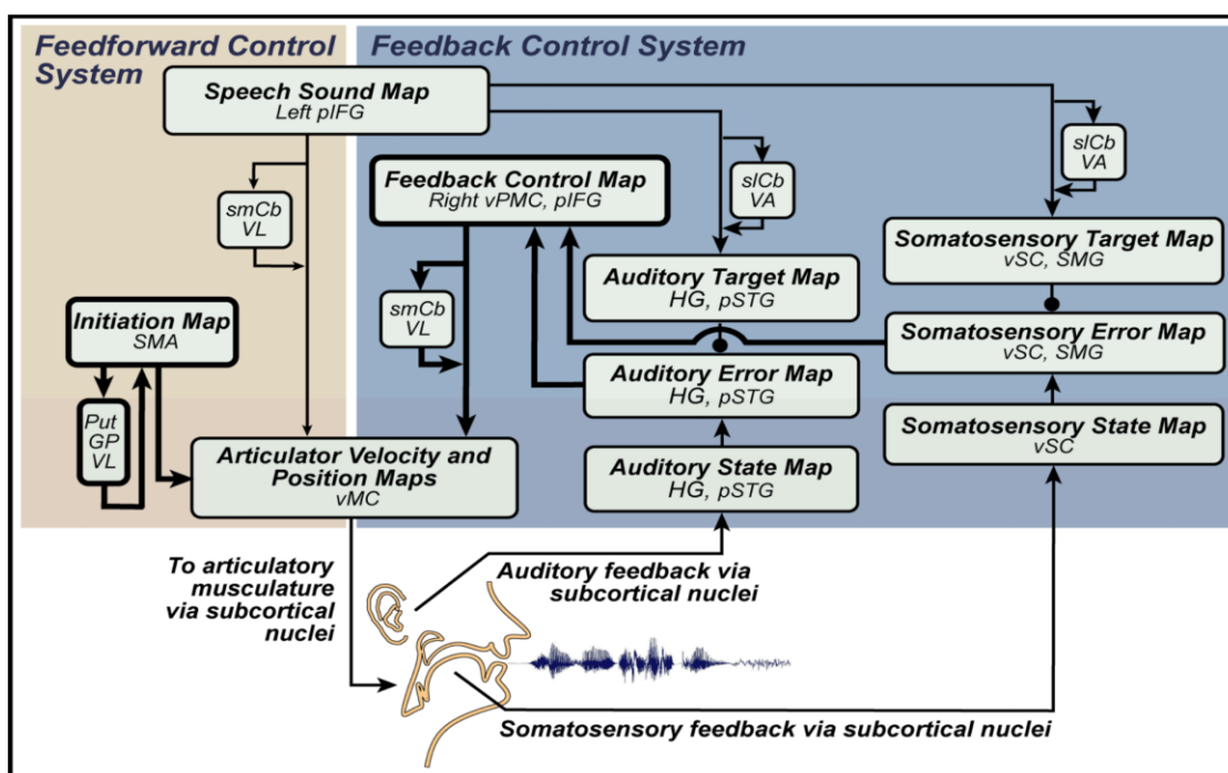
Figura 6 - Modelo DIVA de aquisição e produção de fala
