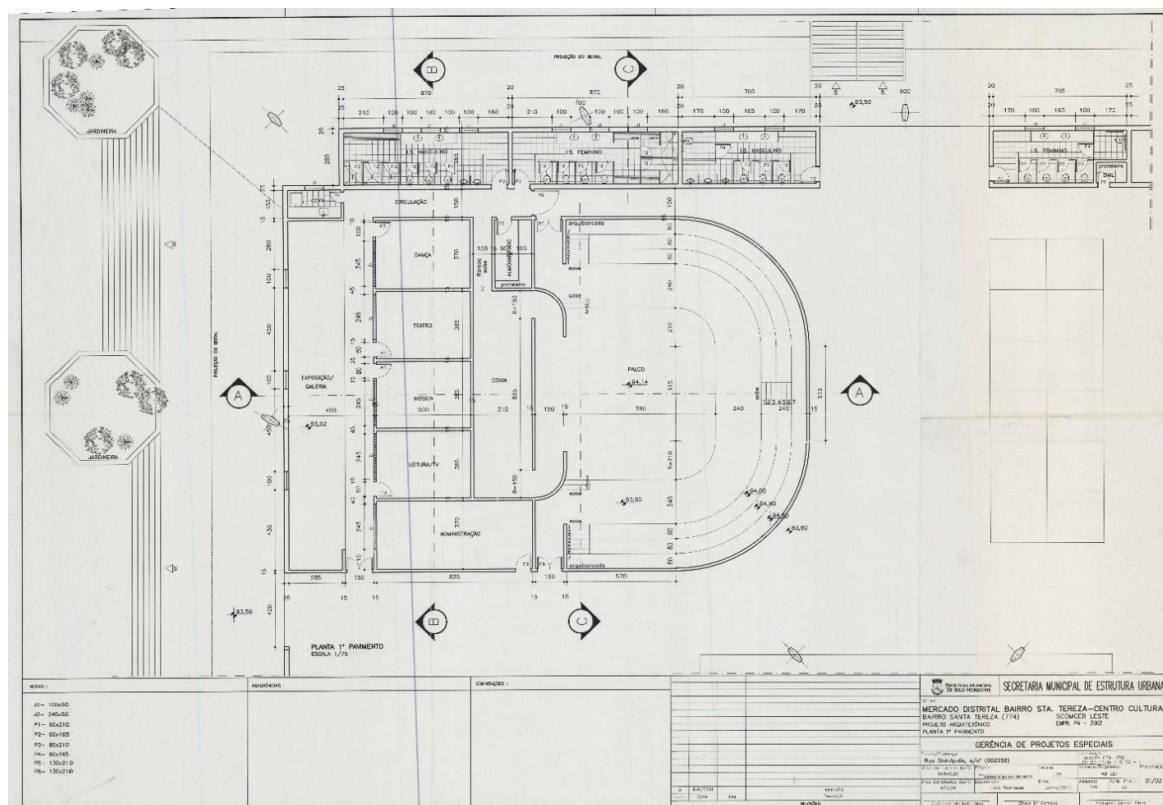
Figura 32 - Projeto arquitetônico do Mercado Distrital Bairro Santa Tereza - Centro Cultural (2002)
