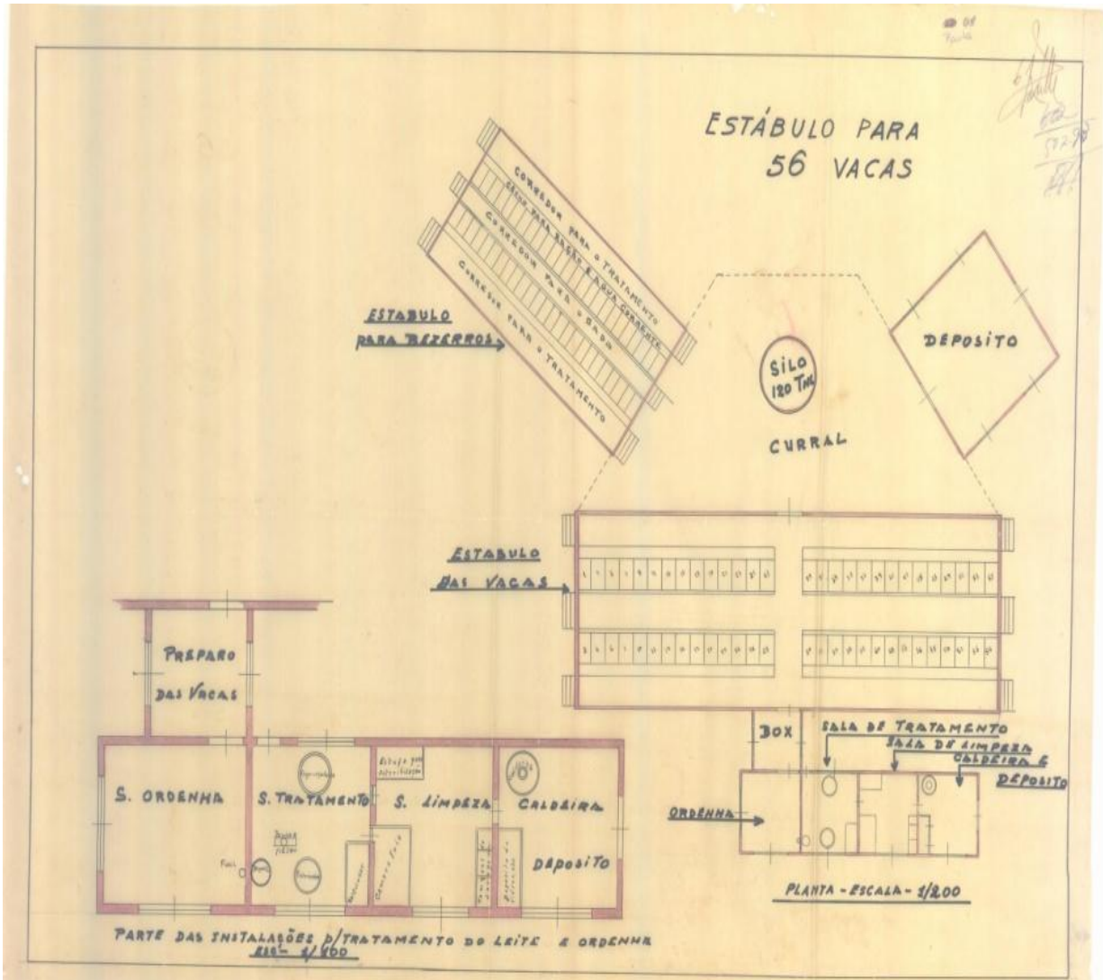
Figura 8 - Parte das instalações para tratamento do leite e ordenha (1948)
