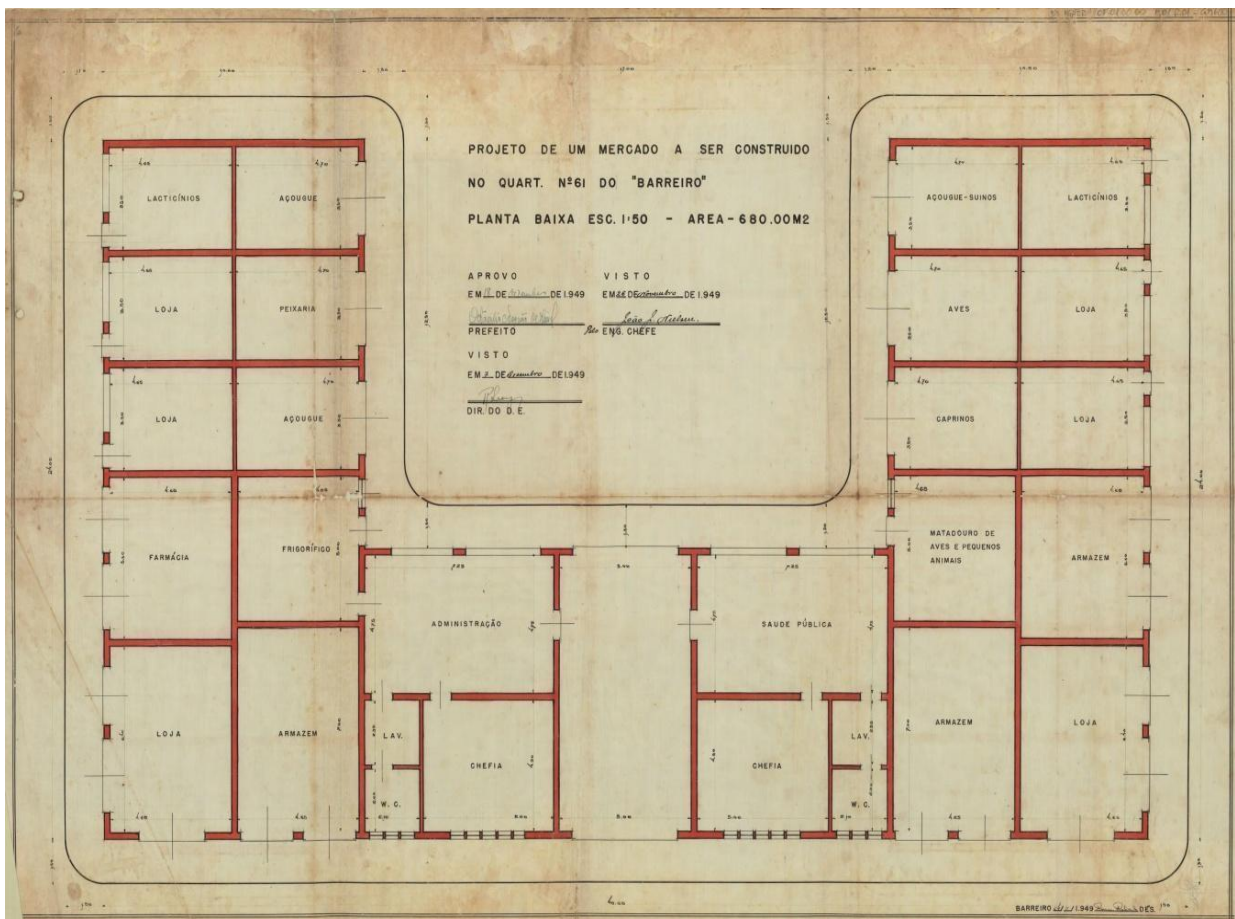
Figura 9 - Projeto de um mercado a ser construído no Barreiro (1949)
