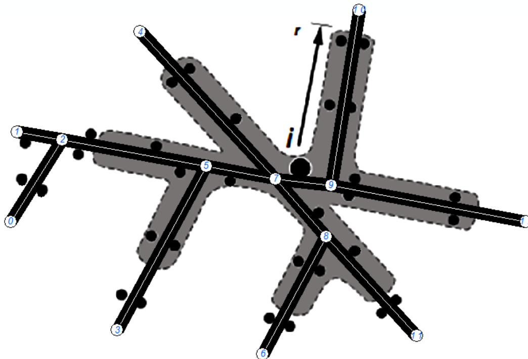
Figura 2: Centralidade por alcance, num raio r .
