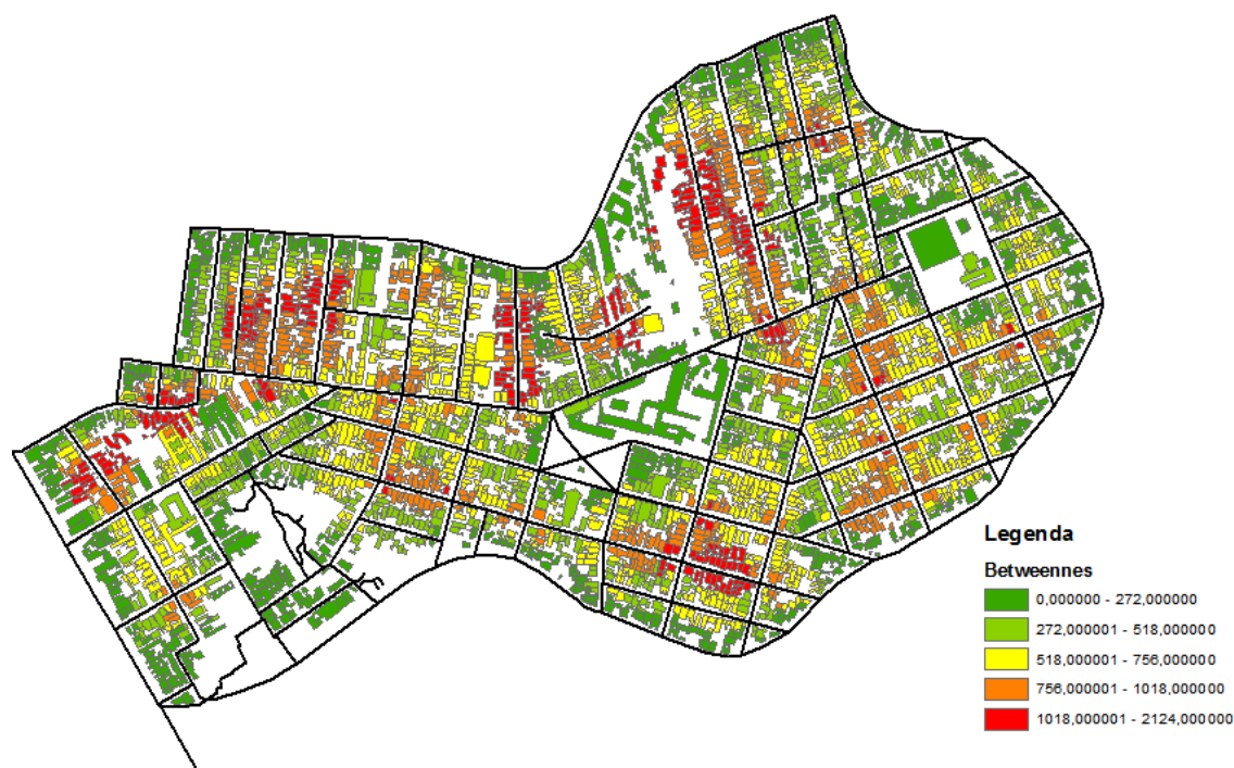
Figura 5: centralidade pela menor rota.
