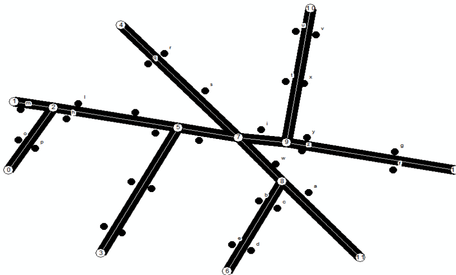
Figura 1: elementos do modelo de rede urbana.
