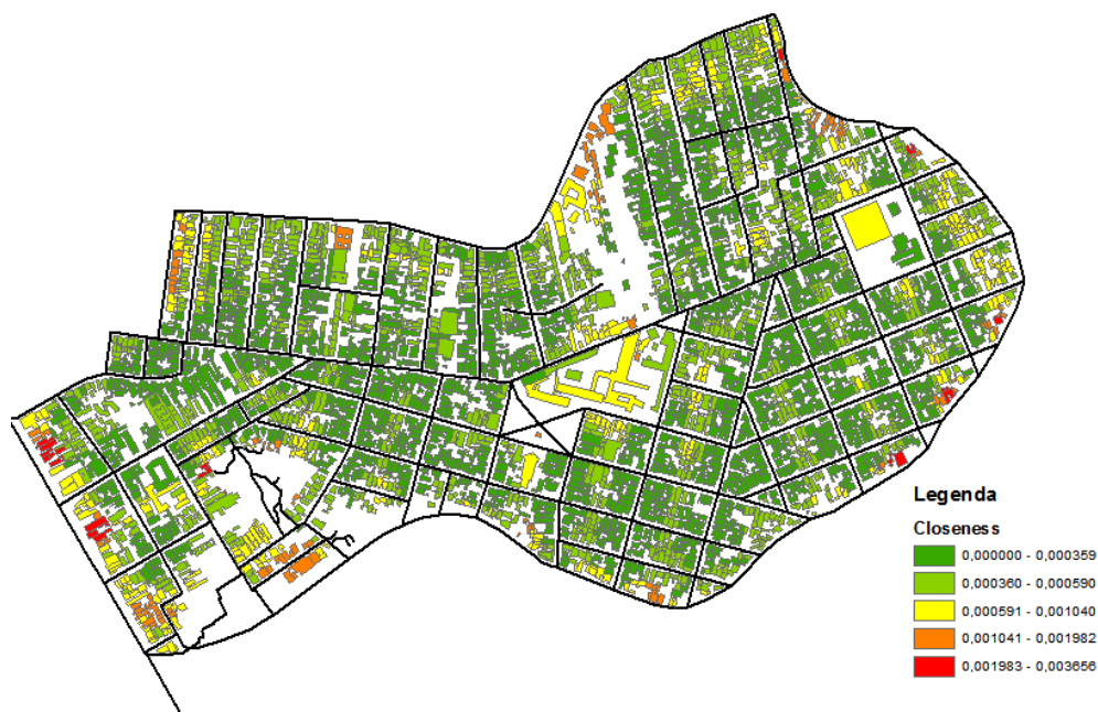
Figura 4: Centralidade por proximidade
