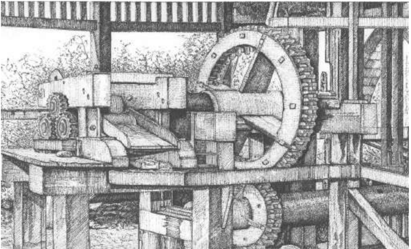
Detalhe da moenda e dos rodetes de engenho d'água. Fazenda da Cachoeira. Município de Dom Joaquim, Minas Gerais. Fotografia de Marcelo M. Godoy (1993). Reprodução em bico-de-pena, por Almir Costa (2003).
