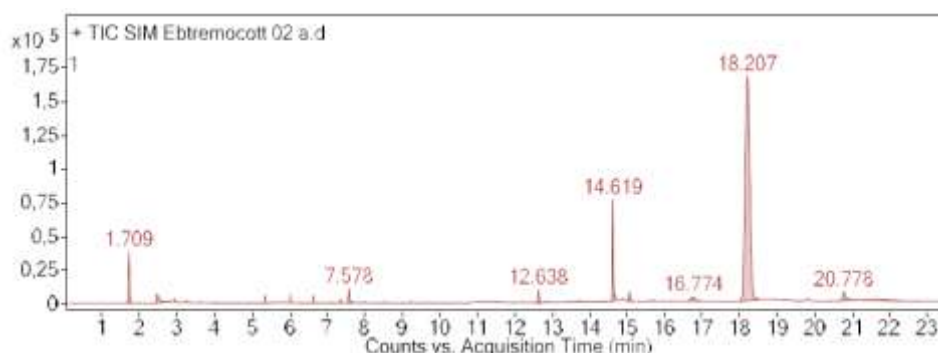
Figura 2: Perfil cromatográfico do extrato de tremçoço com tratamento térmico.
