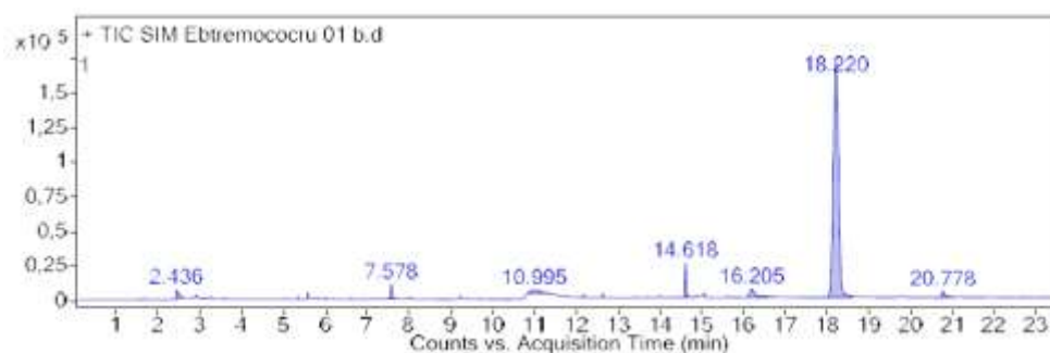
Figura 1: Perfil cromatográfico do extrato de tremçoço cru.
