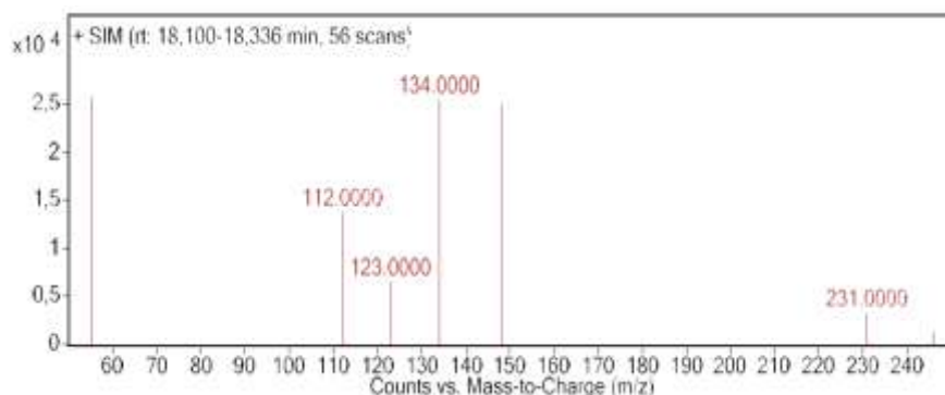
Figura 3: Perfil de fragmentação do pico de lupanina encontrado em 18,2 minutos em extrato de farinha de tremçoço.
