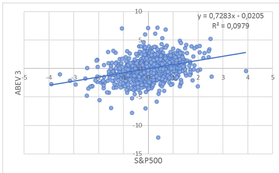
FIGURA 2 – Dispersão com ajuste linear dos retornos ABEV3 e S&P500. Fonte: Elaboração própria com dados da Economatica®.
