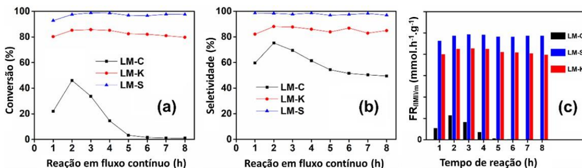
Figura 5.8: Comportamento catalítico de LM-C, LM-S e LM-K para (a) Conversão de BzOH em BzD, (b) Seletividade para formação de IMI por acoplamento de BzD à ANL em fase gasosa e (c) Taxa de formação de IMI pela massa de catalisador ( FR_{(IMI)/m} ).
