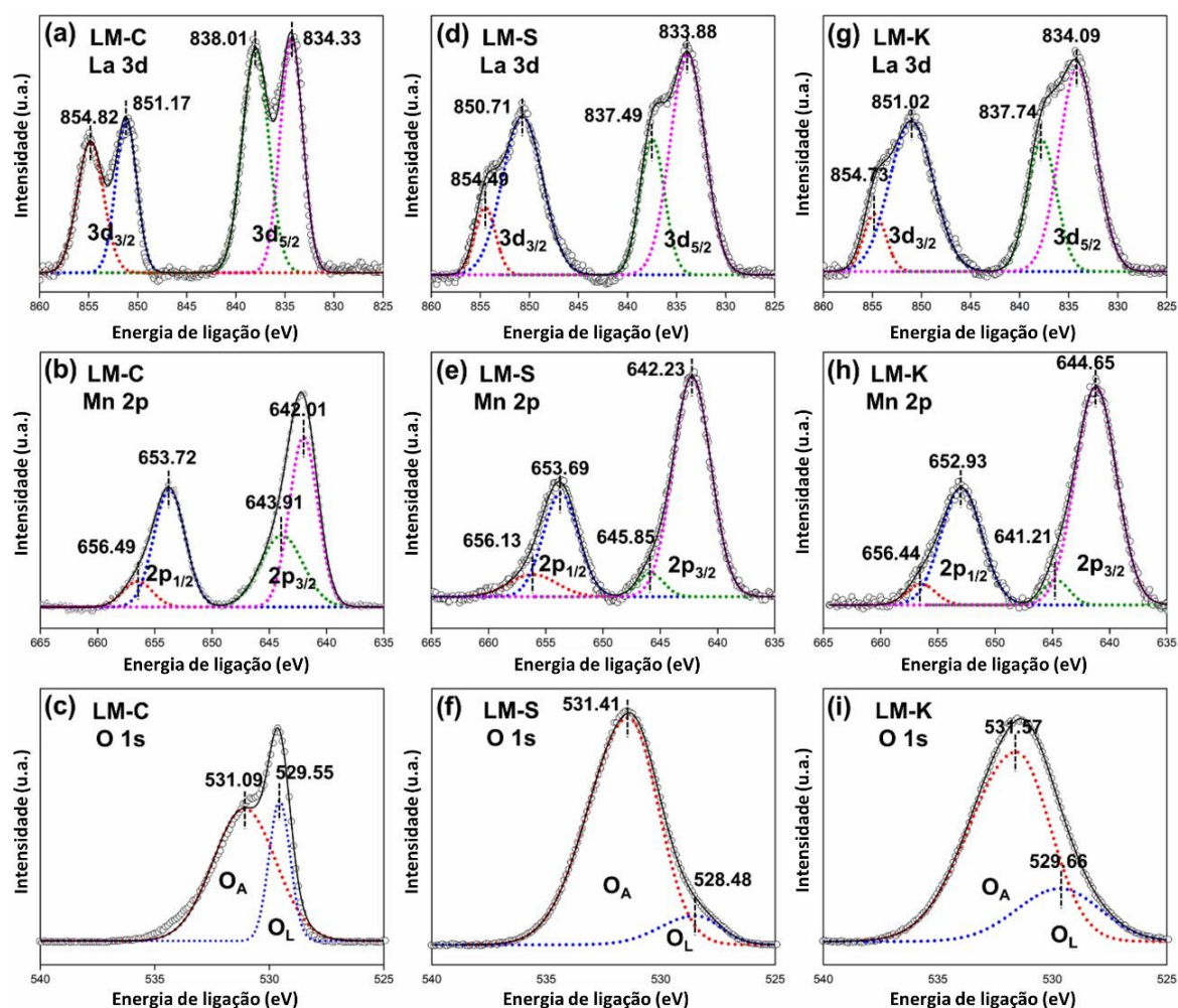
Figura 5.6: Espectros La 3d, Mn 2p, O 1s XPS de perovskitas LM-C (a, b, c), LM-S (d, e, f) e LM-K (g, h, i).
