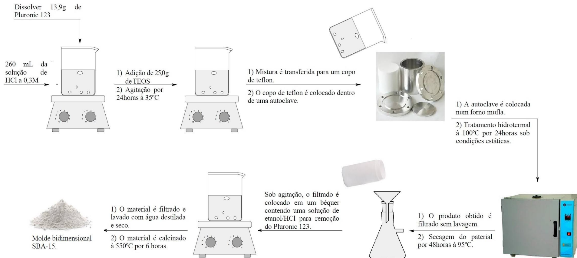
Figura 4.2: Procedimento que será adotado na síntese do molde rígido bidimensional SBA-15.
