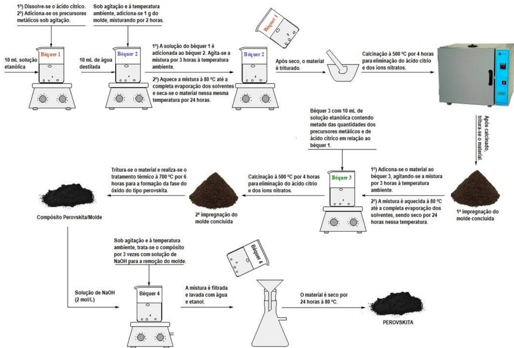
Figura 4.3: Procedimentos adotados para a síntese dos óxidos do tipo perovskitas pelo método nanocasting . Fonte: Próprio autor.
