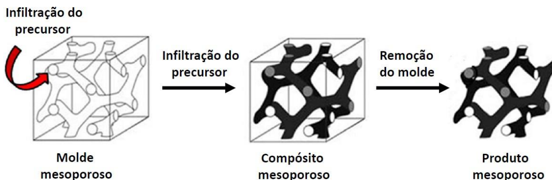
Figura 3.5: Representação esquemática das etapas envolvidas na síntese de material com estrutura de poros ordenada mediante uso de sílica KIT-6 como molde rígido.
