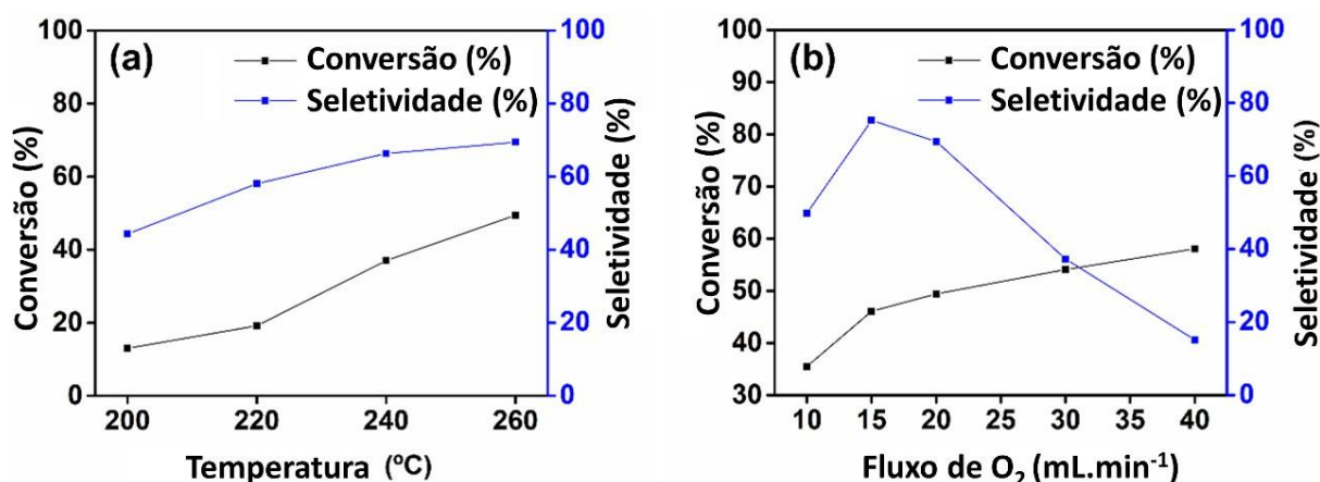
Figura 5.7: Comportamento catalítico do LM-C em função (a) da temperatura de reação e (b) do fluxo de O 2 .
