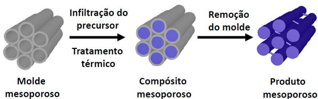
Figura 3.4: Representação esquemática das etapas envolvidas na síntese de material com estrutura de poros ordenada mediante uso de sílica SBA-15 como molde rígido.
