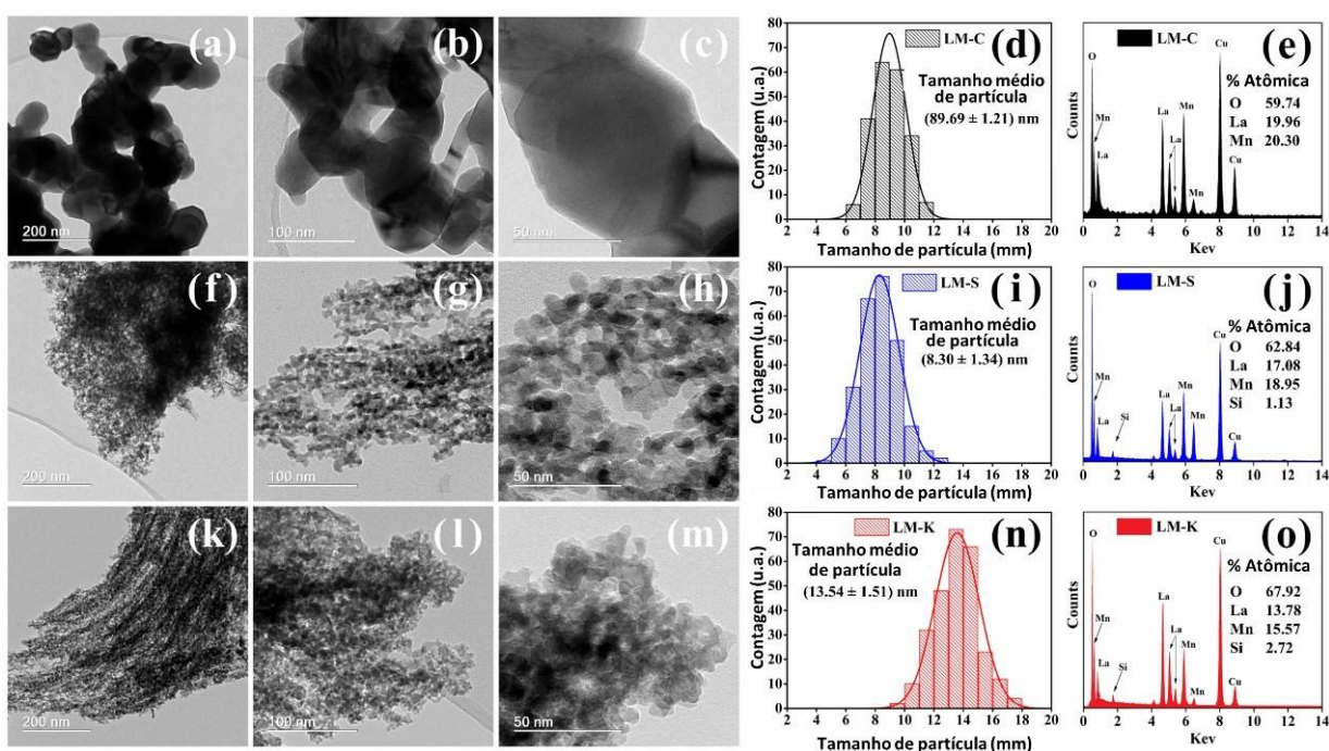
Figura 5.4: Micrografias MET de (a-c) LM-C, (f-h) LM-S e (k-m) LM-K. Distribuições de tamanho de partícula de (d) LM-C, (i) LM-S e (n) LM-K. Espectros EDS de (e) LM-C, (j) LM-S e (o) LM-K.
