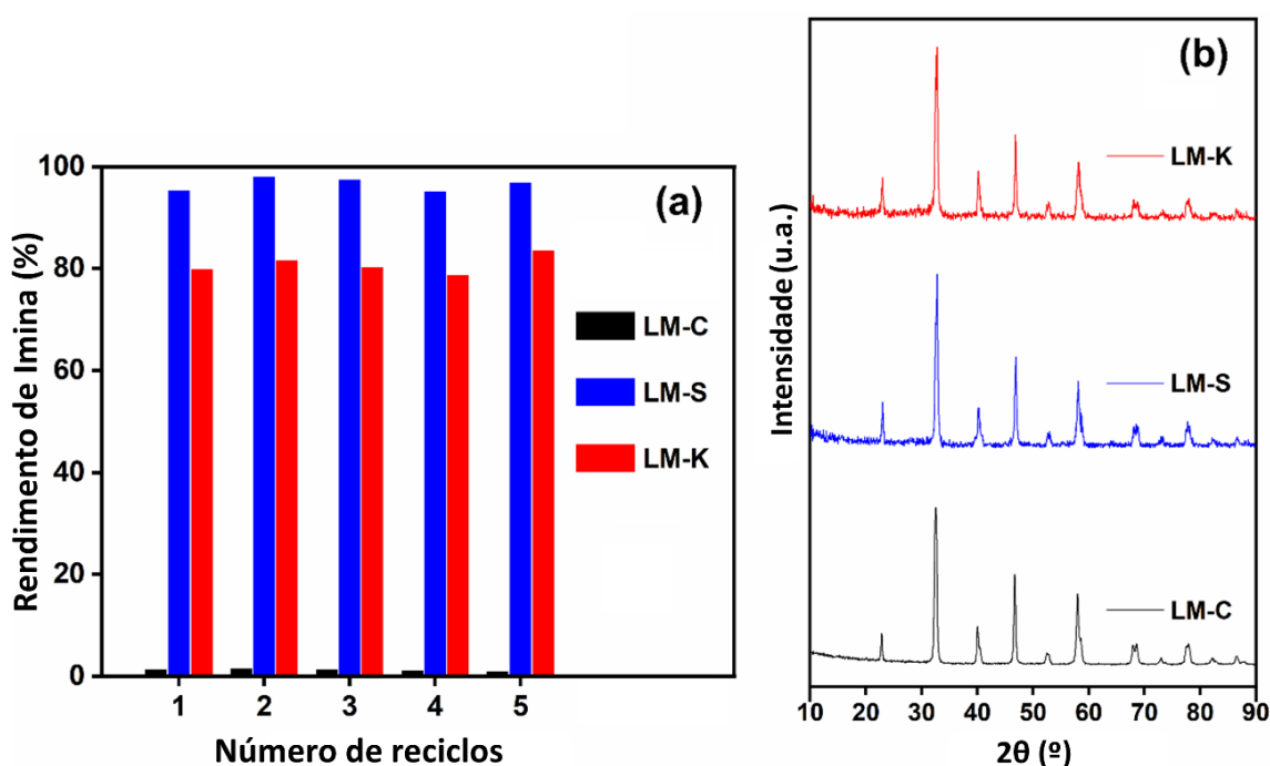
Figura 5.6: (a) Atividade catalítica de LM-C, LM-S e LM-K em sucessivos ciclos. (b) Padrões de XRD coletados para esses catalisadores após serem reciclados e reutilizados por cinco vezes.
