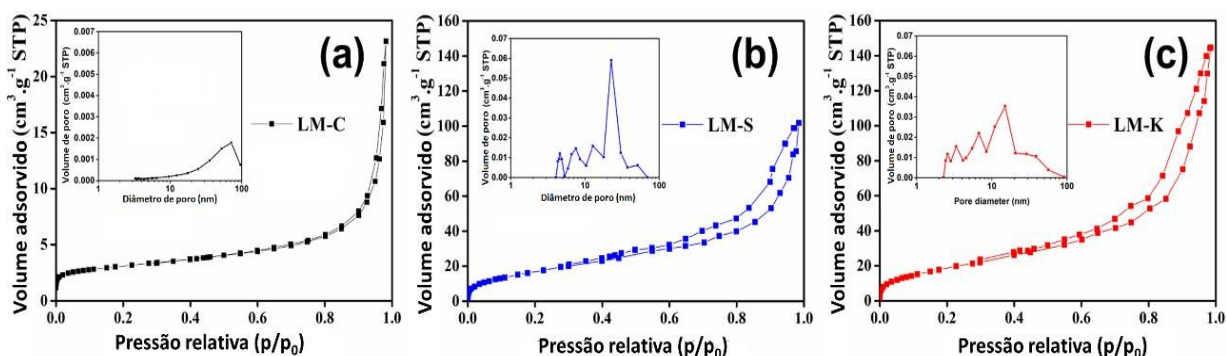
Figura 5.3: Isothermas de sorção de \text{N}_2 e distribuições de tamanhos de poros de (a) LM-C, (b) LM-S e (c) LM-K.
