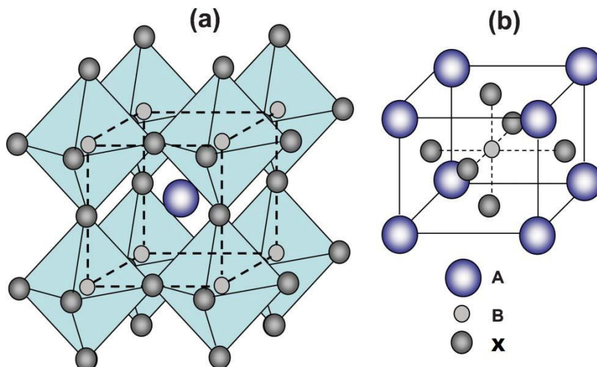
Figura 3.2: Estrutura de perovskita ABX_3 : (a) octaedro de compartilhamento de borda ( BX_6 ) com íon no sítio A coordenado por 12 íons do sítio X; (b) cátion no sítio B no centro da célula.
