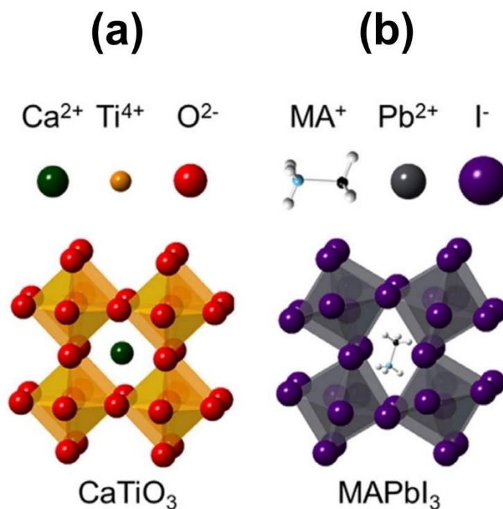
Figura 3.3: Representação da estrutura de óxidos do tipo perovskita (não está em escala): (a) Perovskita inorgânica com íon \text{Ca}^{2+} ocupando o sítio A e (b) perovskita híbrida com cátion da molécula metilamônio (MA) ocupando o sítio A.
