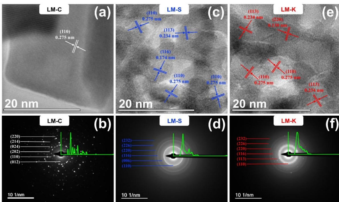
Figura 5.5: Imagens MET de alta resolução de (a) LM-C, (c) LM-S e (e) LM-K. Padrões SAED de perovskitas (b) LM-C, (d) LM-S e (f) LM-K.
