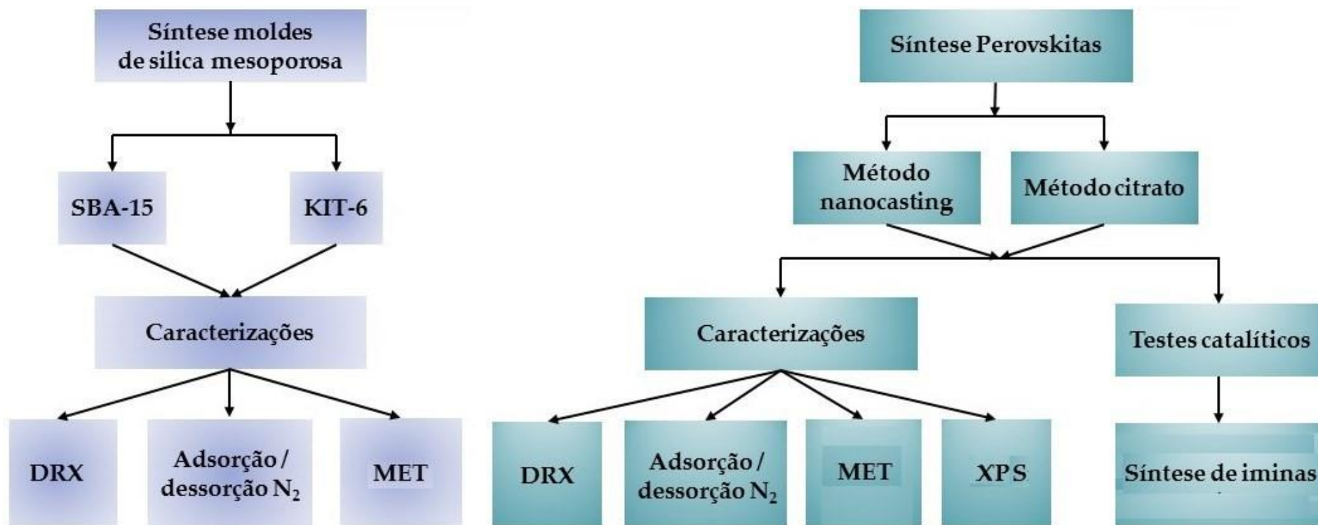
Figura 4.1: Fluxograma resumido das etapas de síntese de \text{LaMnO}_3 e testes catalíticos.
