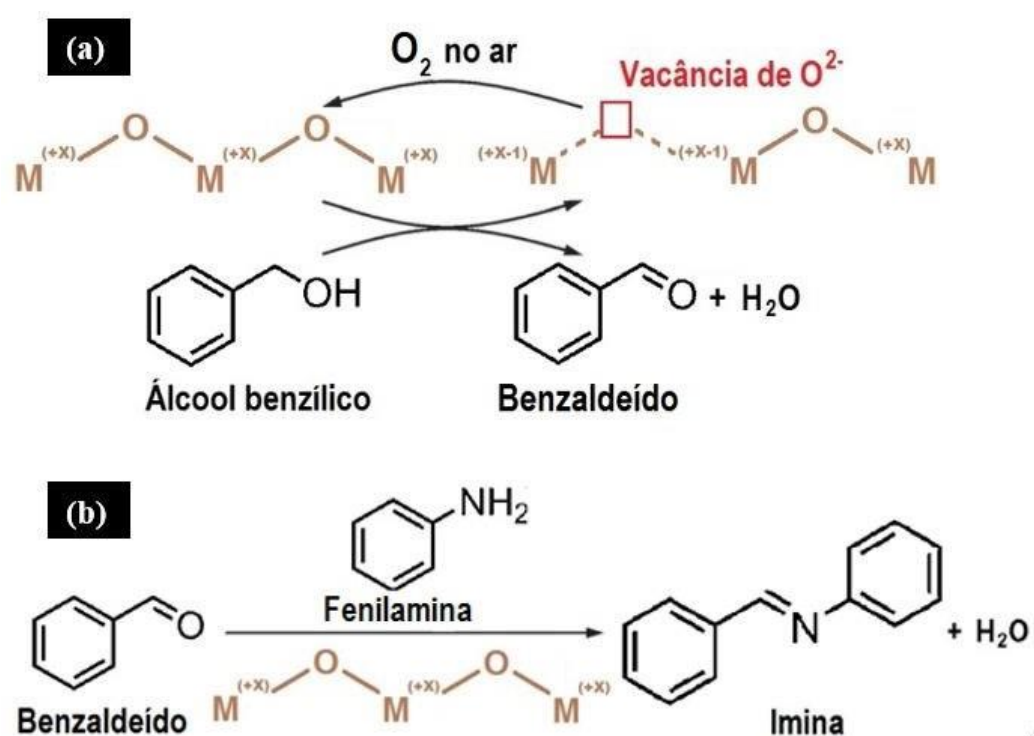
Figura 3.7: Mecanismo de reação para a formação de imina por meio do acoplamento oxidativo de álcoois e aminas: (a) Reação de formação do benzaldeído e (b) reação de condensação.
