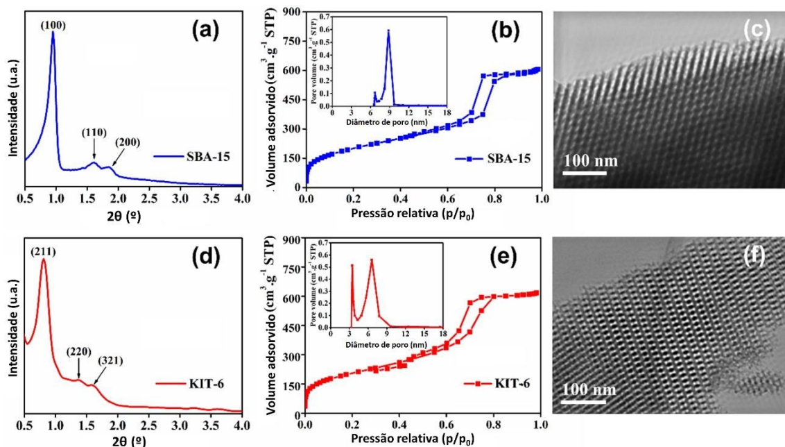
Figura 5.1: Padrão de DRX de baixo ângulo para (a) SBA-15 e (d) KIT-6. Isotermas de sorção de N_2 e distribuição de tamanhos de poros de (b) SBA-15 e (e) KIT-6. Micrografias obtidas por MET para (c) SBA-15 e (f) KIT-6.
