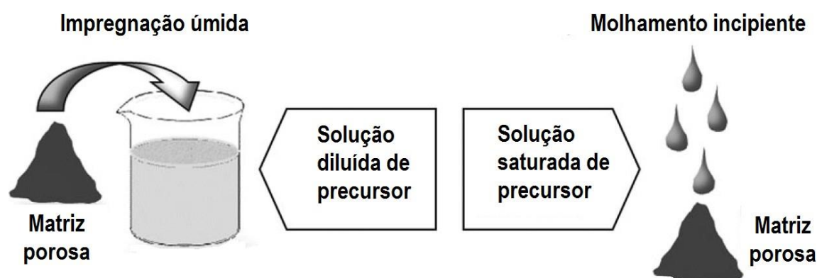
Figura 3.6: Desenho esquemático das técnicas de impregnação úmida e molhamento incipiente para a infiltração de espécies precursoras em matrizes de estruturas porosas.
