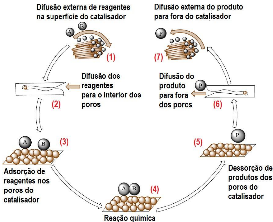
Figura 3.1: Etapas envolvidas na catálise heterogênea: A e B são os reagentes e P é o produto. Fonte: Adaptado de Unnikrishnan & Srinivas (2016) [47].
