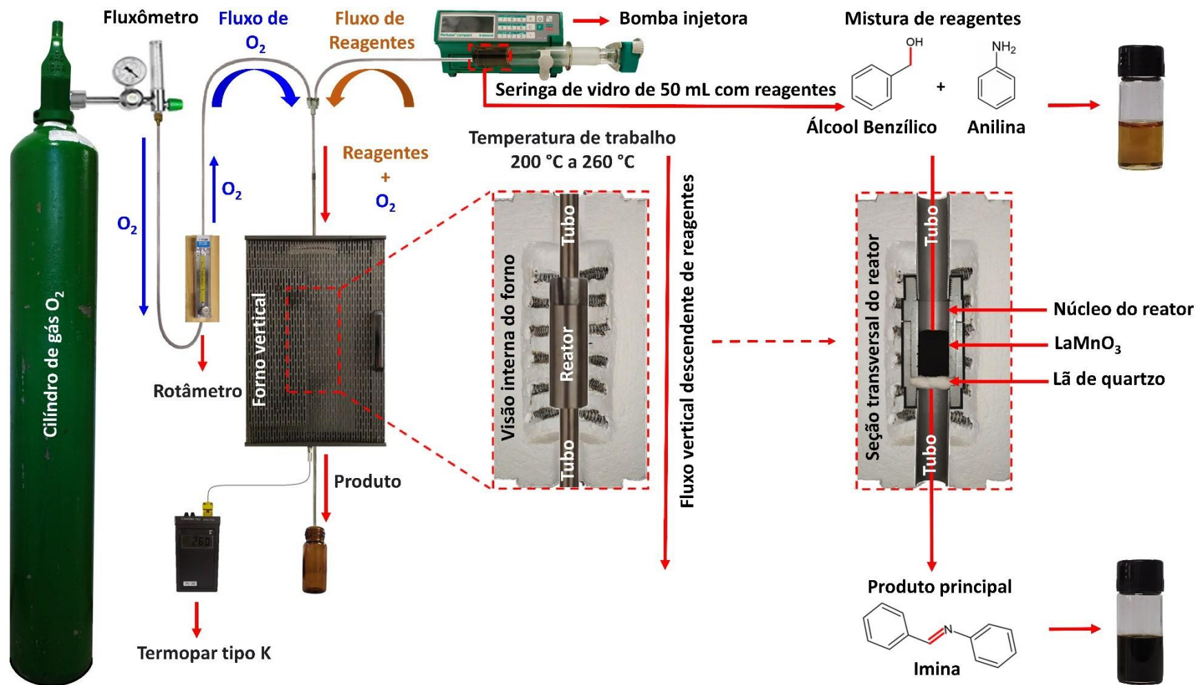
Figura 4.4: Montagem real dos instrumentos e equipamentos utilizados na síntese de imina.
