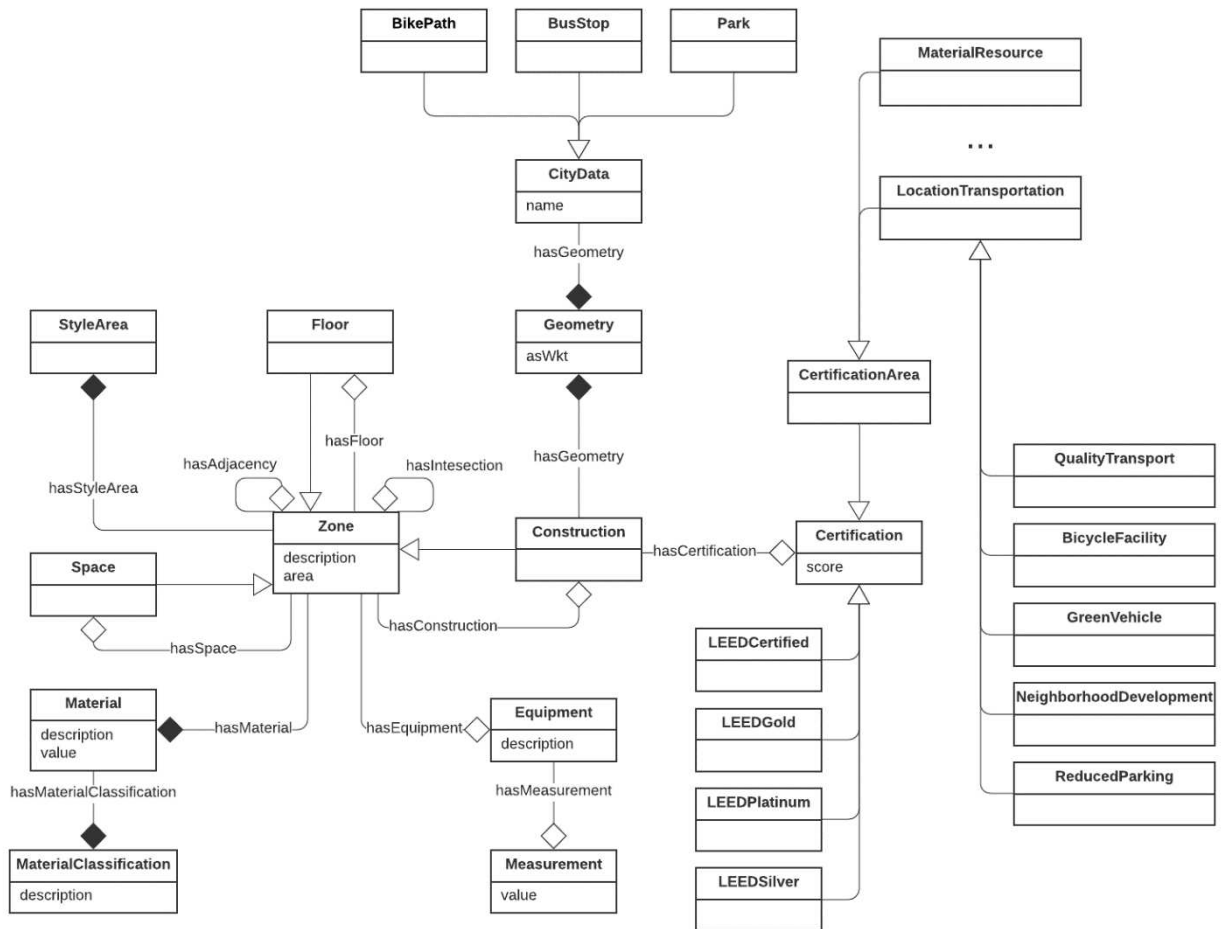
Figura 2: Ontologia simplificada
