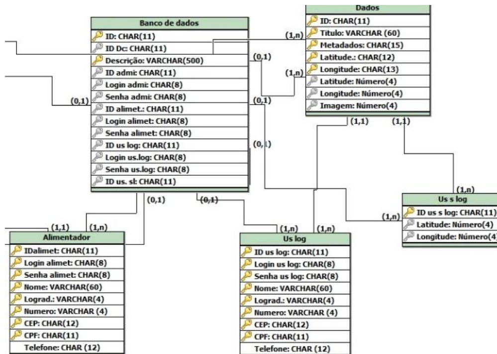
Figura 5: Diagrama entidade/relacionamento
