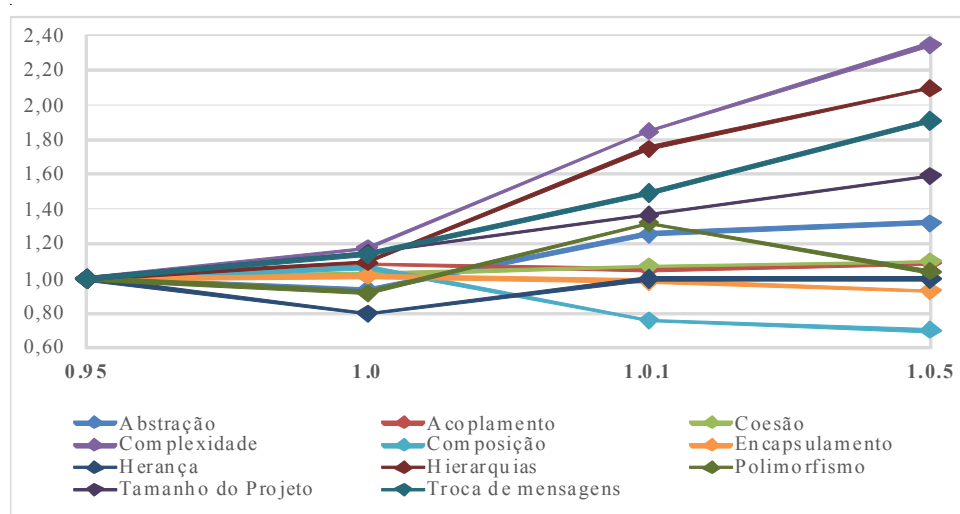
Figura 2 - Resultado das propriedades de projeto baseado no QMOOD
