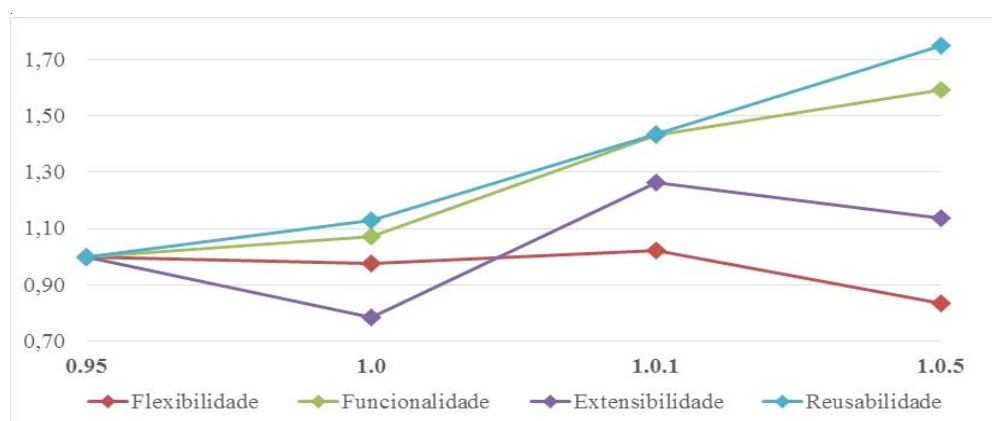
Figura 3 - Resultado dos atributos de qualidade Flexibilidade, Funcionalidade, Extensibilidade e Reusabilidade.
