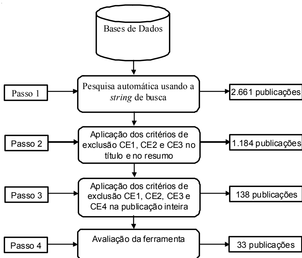
Figura 1 - Estratégia de pesquisa para a questão de pesquisa Q4
