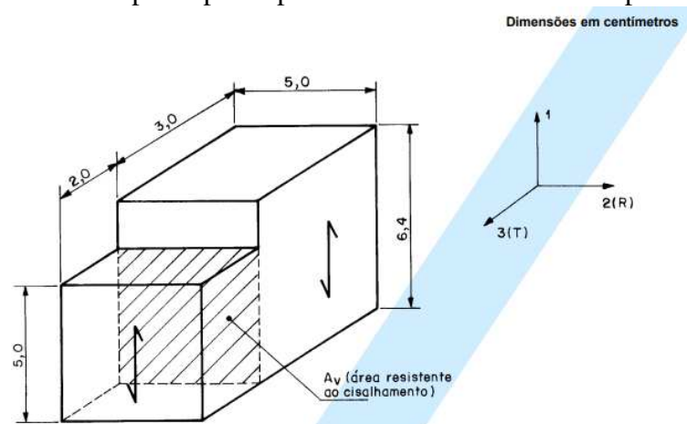
Figura 1: Padrão do corpo de prova para ensaios de cisalhamento paralelo às fibras
