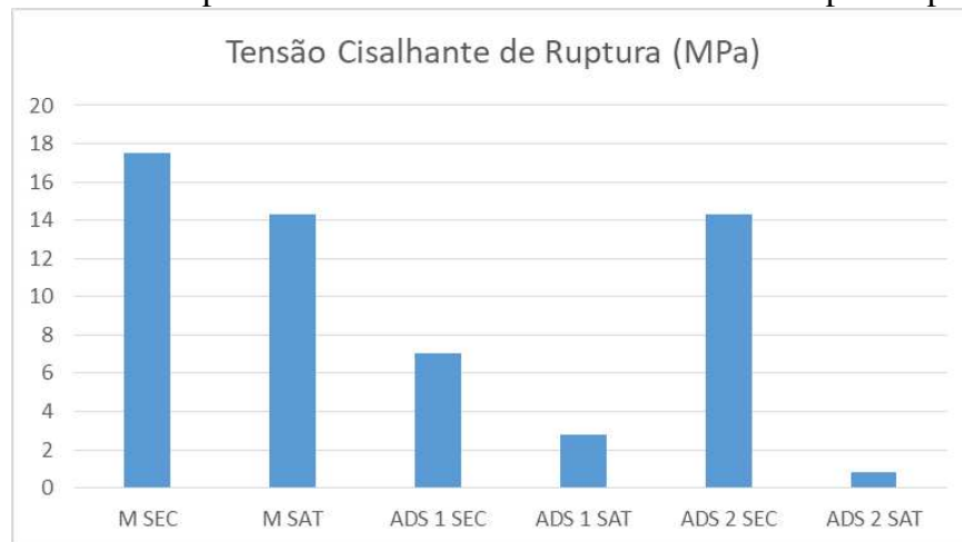
Gráfico 1: Comparativo de Tensão de cisalhamento dos corpos de prova
