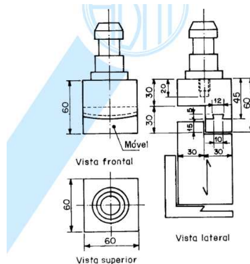
Figura 2: Dispositivo para ensaios de cisalhamento paralelo às fibras
