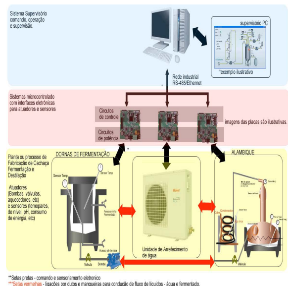
Figura 3 – Diagrama da planta piloto automatizada.
