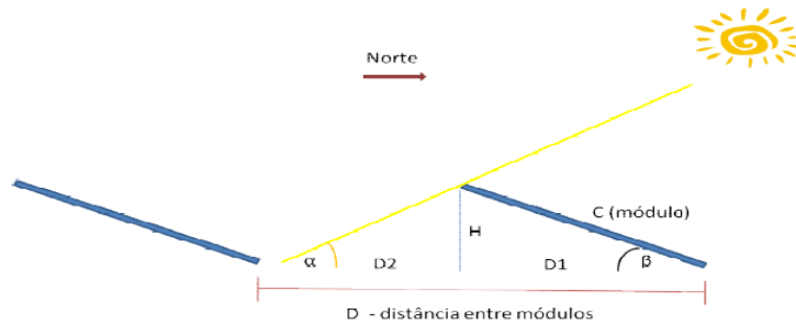
Figura 3- Triângulo de representação da posição do painel instalado.
