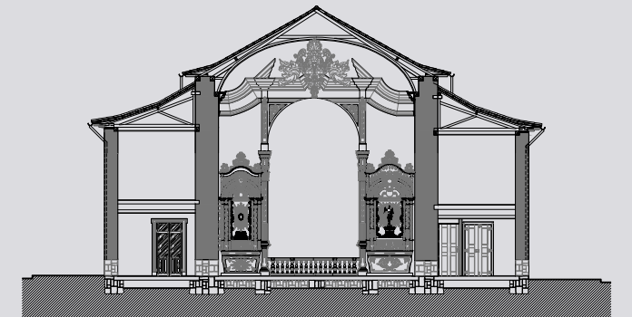
CORTE TRANSVERSAL BB
