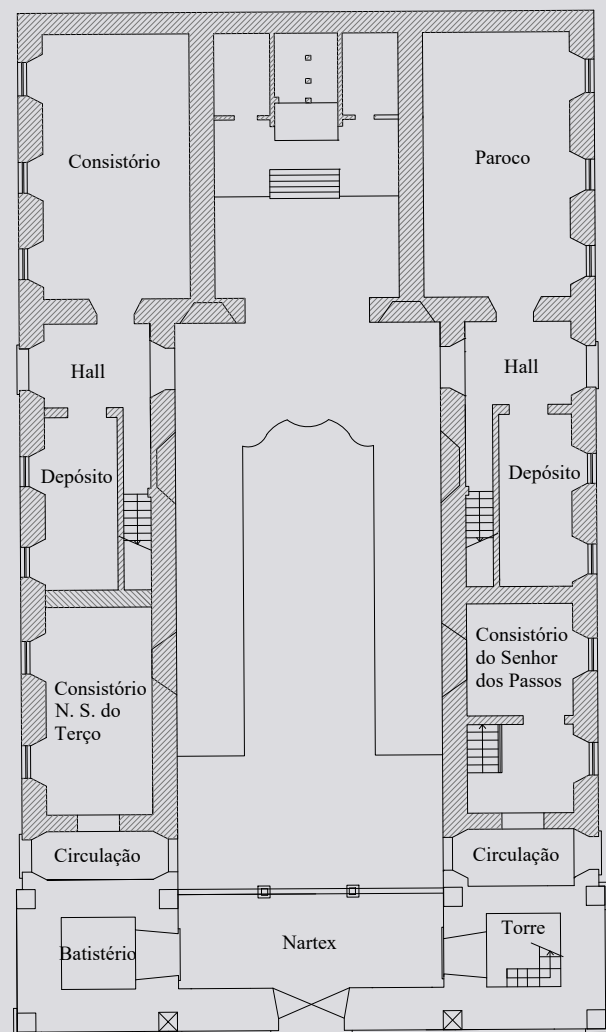
PLANTA NÍVEL TÉRREO - 1750
