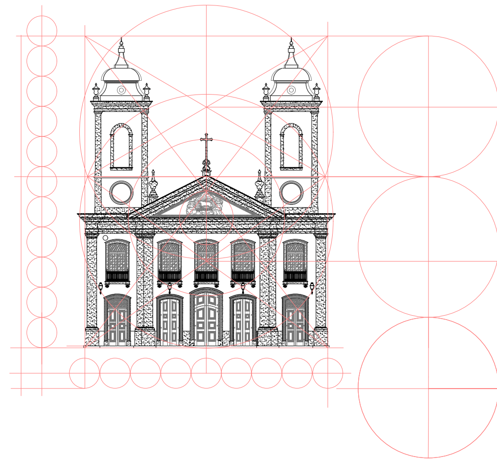
Fig. 55 – Os estudos dos traçados geométricos que orientaram o projeto da atual Catedral Basílica de Nossa Senhora do Pilar, estão de sobremaneira imbuídos da cultura arquitetônica neoclássica, pautada na racionalidade projetual e no conceito de rigor e ordem arquitetônica, o que faz com que seja impossível não atribuir esse projeto a um arquiteto erudito, com pleno conhecimento do que se fazia em termos de arquitetura e urbanismo na Corte do Rio de Janeiro entre 1820 a 1860. Neste sentido, pensamos, que o arquiteto e ferreiro Jesuino José Ferreira, que inclusive fez um risco para nova Prefeitura em 1830, seja um bom candidato a ser o arquiteto responsável por esse risco, ainda que maiores estudos precisem ser feitos. Fonte: Reconstrução gráfica feita pela arquiteta Luiza Salles Araújo
