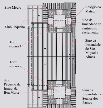
PLANTA TORRES
