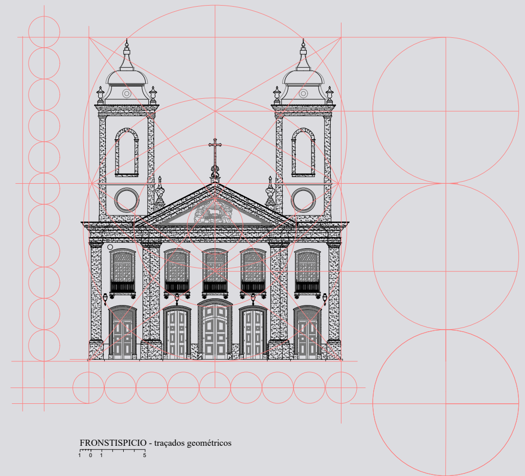
FRONSTISPICIO - traçados geométricos 1 0 1 5
