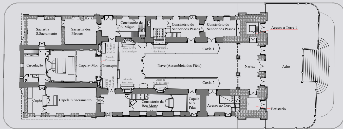
PLANTA BAIXA
