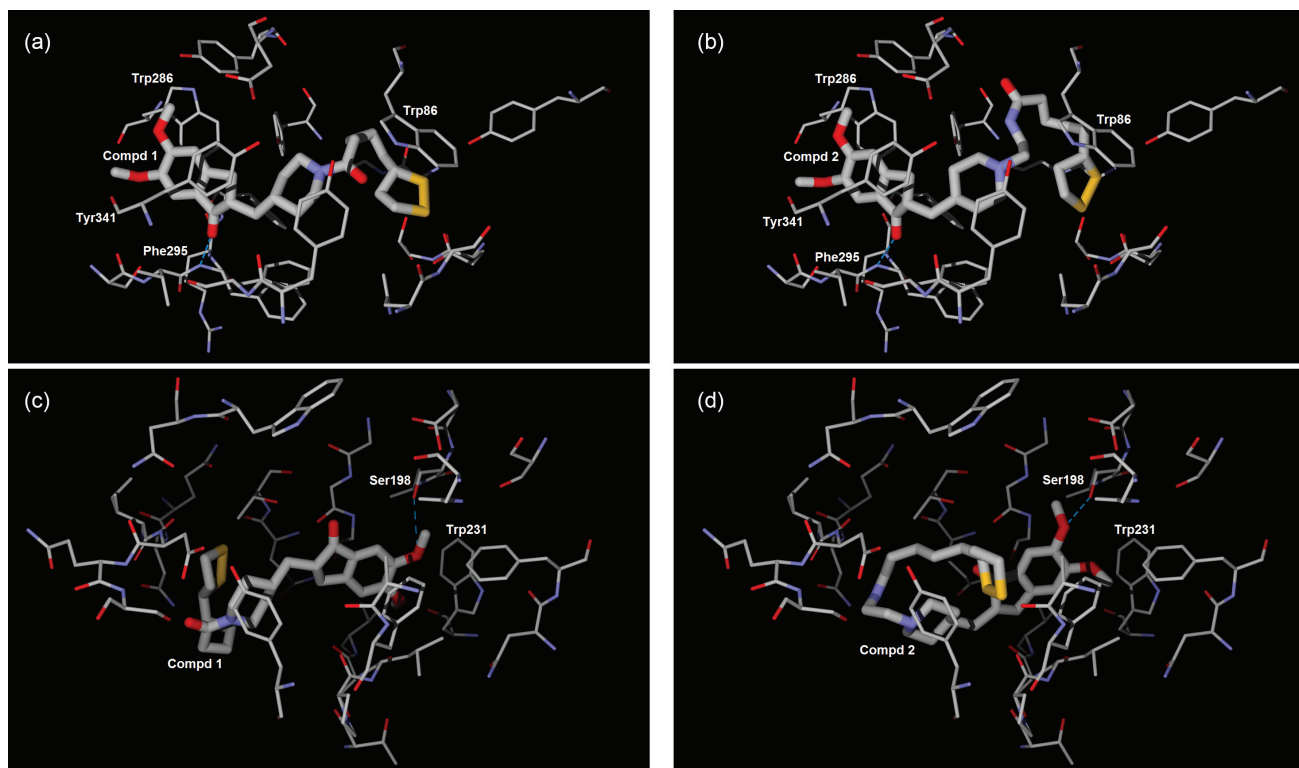
Figure 5. Docking models for (a) AChE ( 1 ); (b) AChE ( 2 ); (c) BuChE ( 1 ); (d) BuChE ( 2 ).
