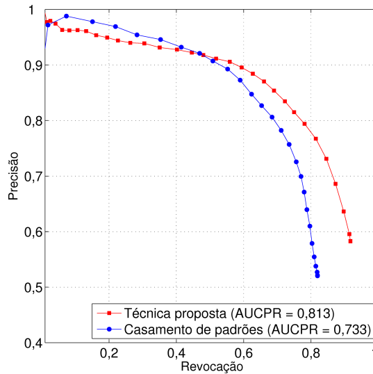
Figura 2: Curvas precisão-revoação obtidas para a técnica proposta (medida de blobness - linha vermelha) e para a técnica casamento de padrões (linha azul) usando todos os quadros do vídeo de MI.
