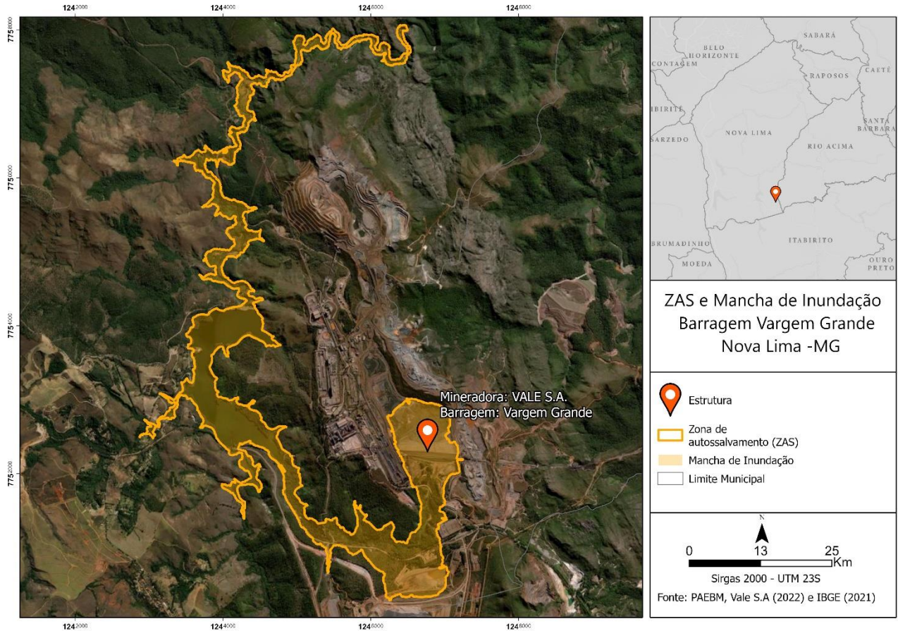
Figura 2 – ZAS e Mancha de Inundação da Barragem Vargem Grande (Nova Lima - MG)
