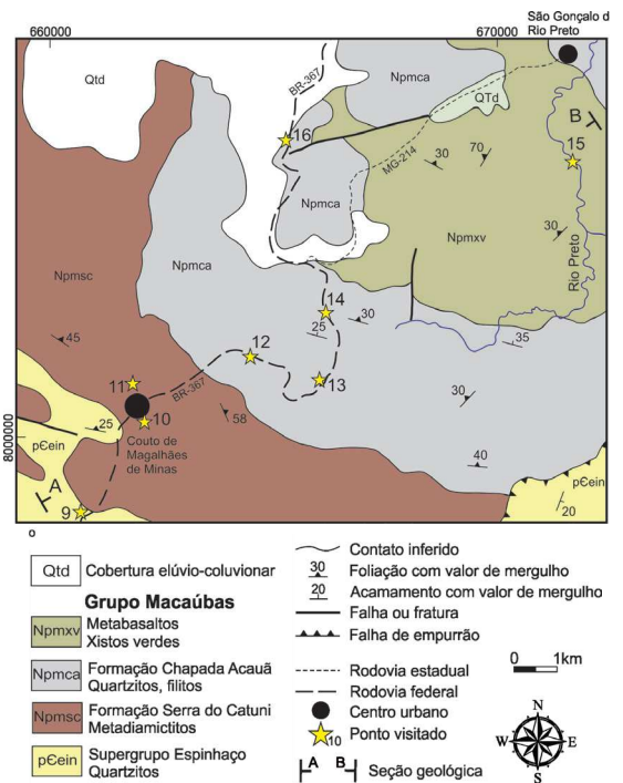
Figura 5. Mapa geológico simplificado de Couto de Magalhães de Minas com localização dos pontos visitados. Veja localização da seção geológica A-B. Modificado de Tupinambá et al. 1996
