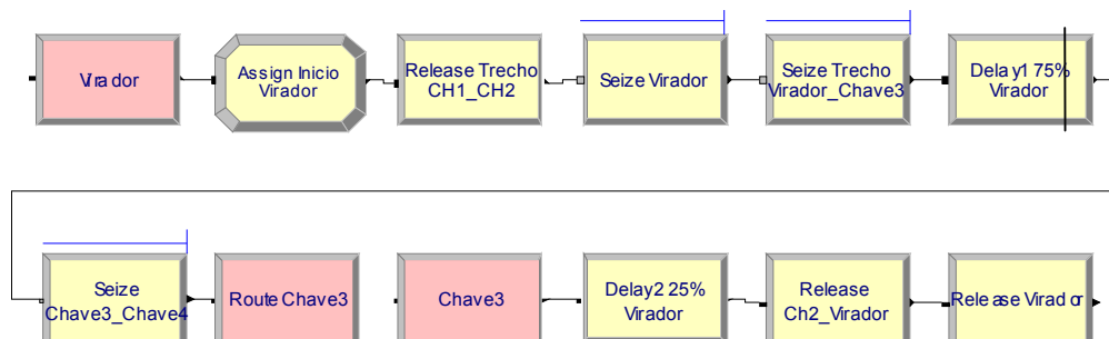
FIGURA 4.5 - Lógica do modelo para as atividades no virador
