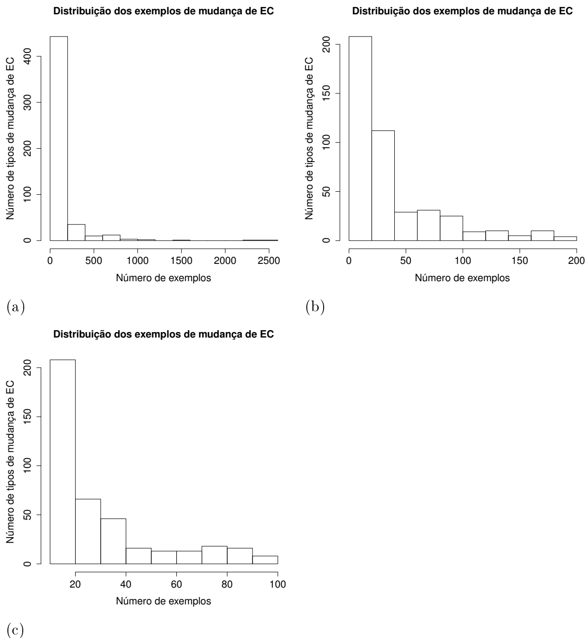
Figura 4.8: O número de exemplos de mudanças de EC é apresentado no eixo x e o número de tipos de mudanças de EC é apresentado no eixo y . Em (a) o histograma mostra o número de exemplos de mudanças de EC para todos os 508 tipos de mudanças de EC com pelo menos 10 exemplos; em (b) somente tipos de mudanças com menos de 200 exemplos são apresentadas; em (c) tipos de mudanças com menos que 100 exemplos são exibidos. O limite superior definido para o número de exemplos do conjunto controle foi a mediana do número de exemplos de mudança de EC, que é 27. Tal valor é mais representativo que a média, que é 102,2 com desvio padrão 224,6.
