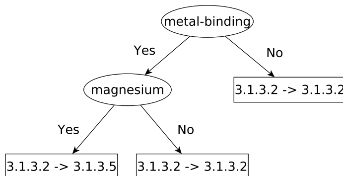
Figura 4.11: Árvore de decisão gerada com base nos dados da Tabela 4.6.
