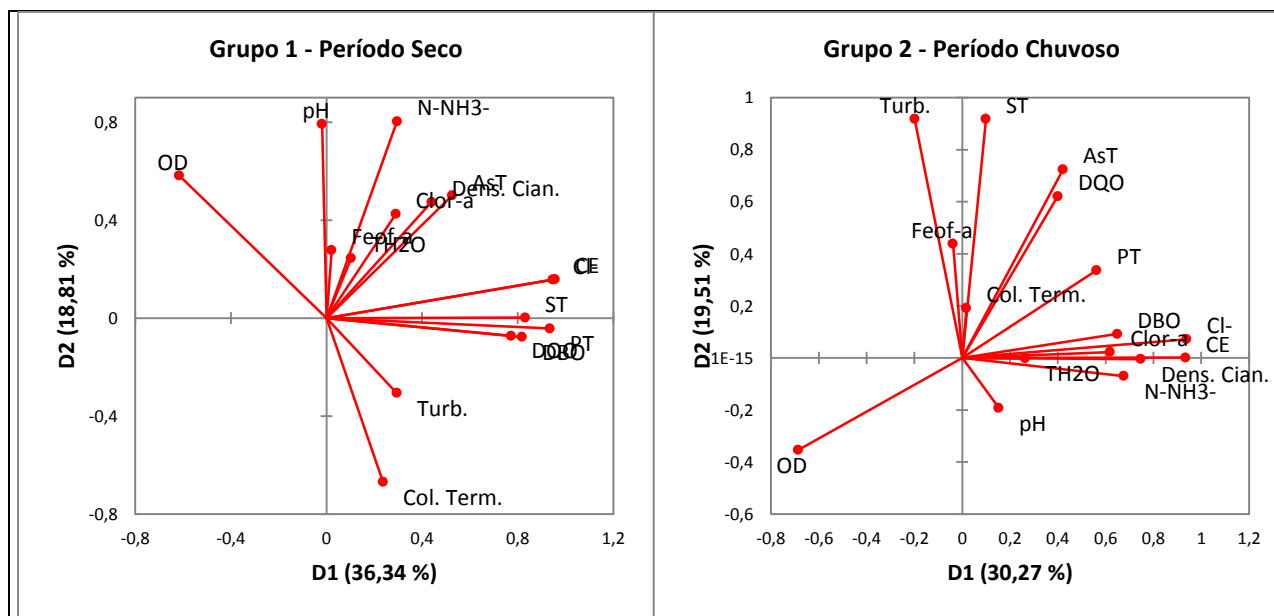
Figura 5.3. Gráficos das cargas dos dois primeiros fatores extraídos após rotação varimax das Componentes Principais, referentes à análise temporal do banco de dados de monitoramento mensal do rio das Velhas.
