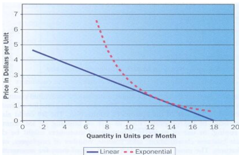
Figura 3.22 – Curvas típicas de demanda de água. Eixo das abscissas em unidades de consumo mensal. Eixo das ordenadas em US$ por unidade consumida. Fonte: Billings & Jones, 2008
