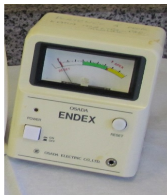
Fig.4 – Localizadores eletrônicos de forame apical utilizados no estudo: Romipex e Endex.
