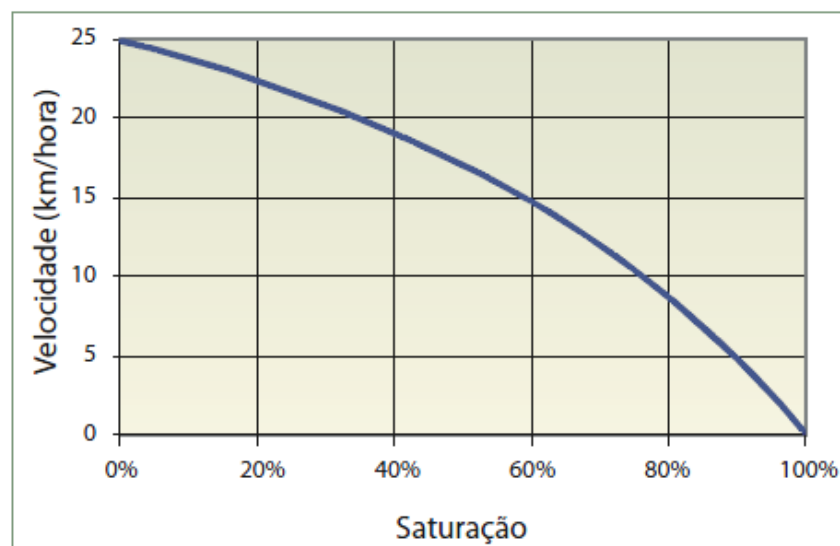
Figura 2.6 – Impacto da saturação na velocidade dos veículos nas estações (Manual de BRT, 2008, p. 267)
