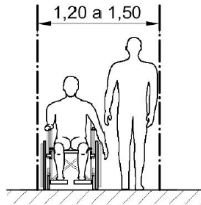
Figura 4.44 – Largura para deslocamento em linha reta – cadeirante e pedestre (NBR 9050/2004, p. 6)
