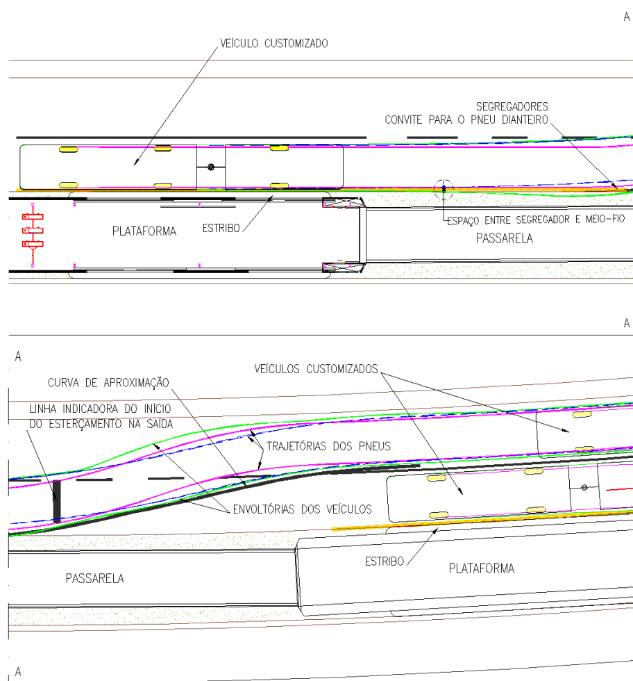
Figura 4.36– Projeto de definição dos elementos de auxílio à atracagem do BRT MOVE (BHTRANS, 2013)
